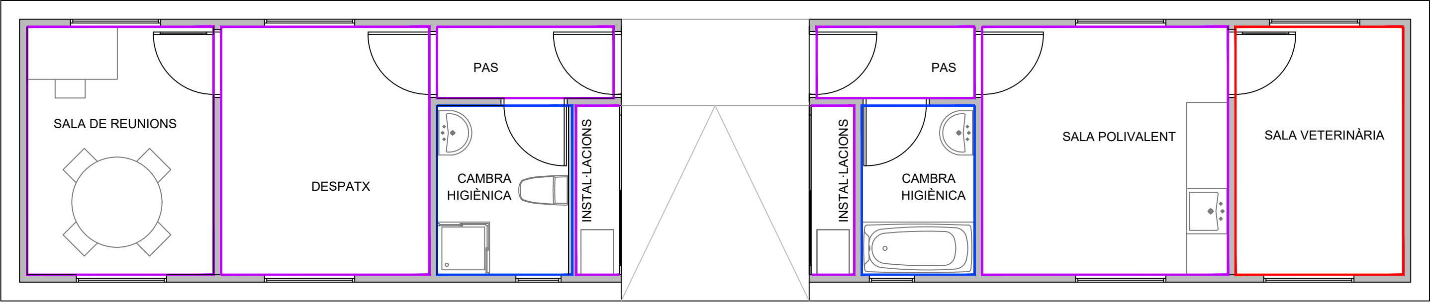
PLANTA E: 1/50
