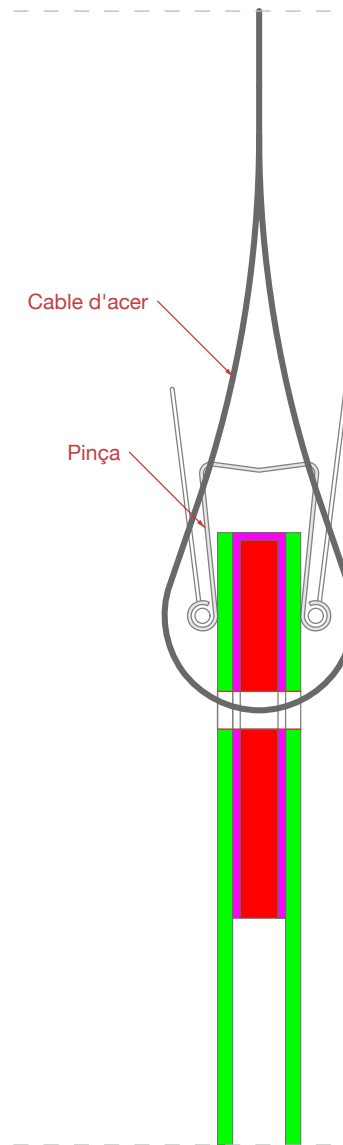
Detall A - Escala 1:1 Sistema de suspensió cortina
