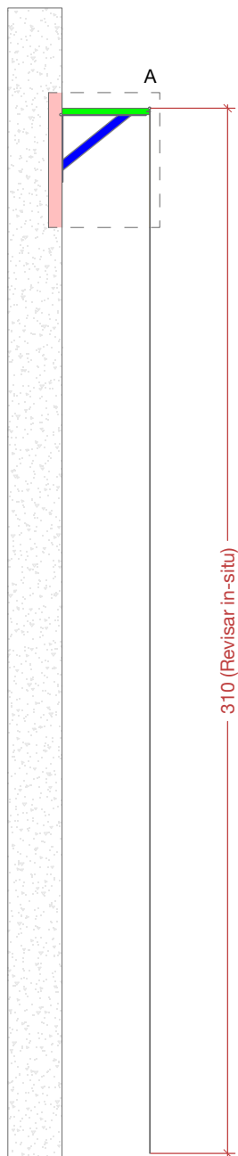
Secció A-A Escala 1:20
