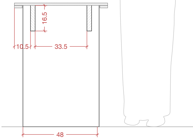
Secció A-A
