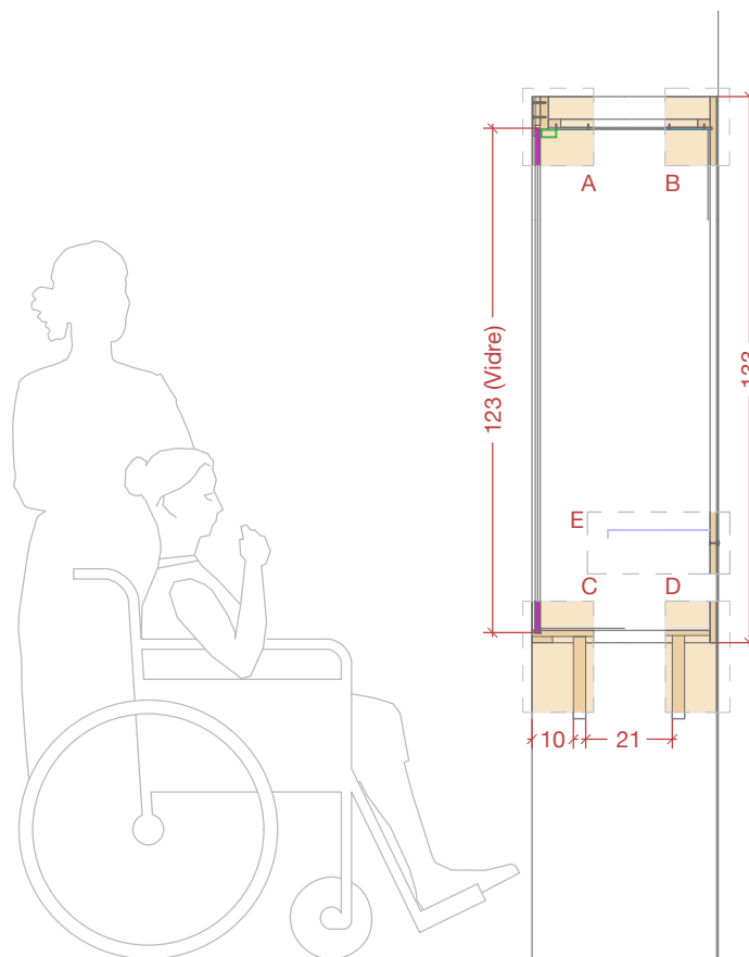
Secció Lateral
