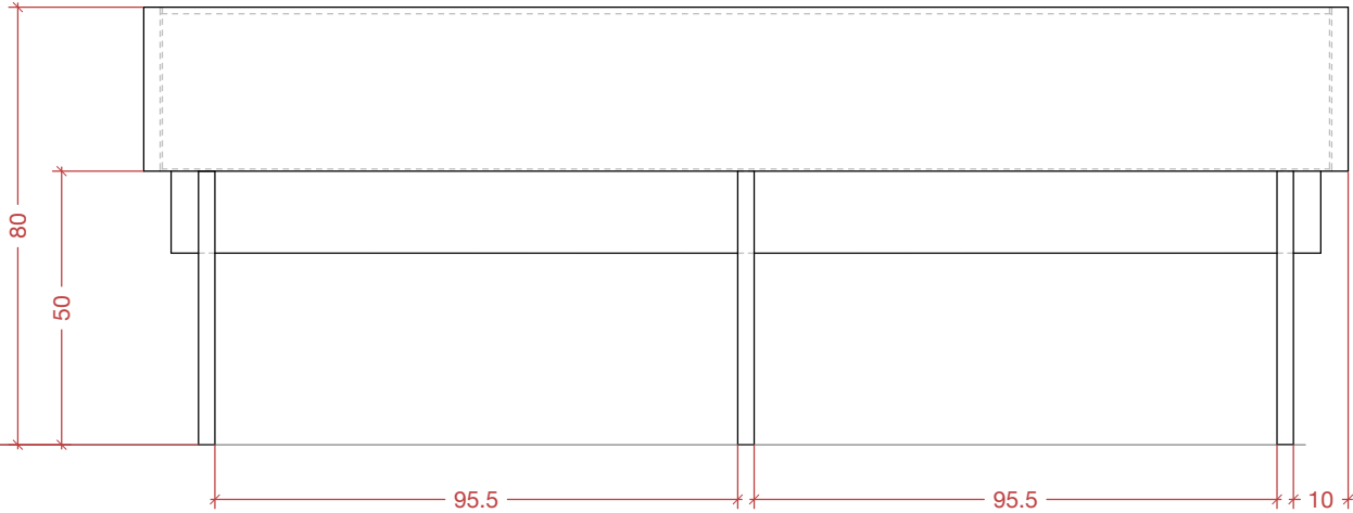
Alçat
