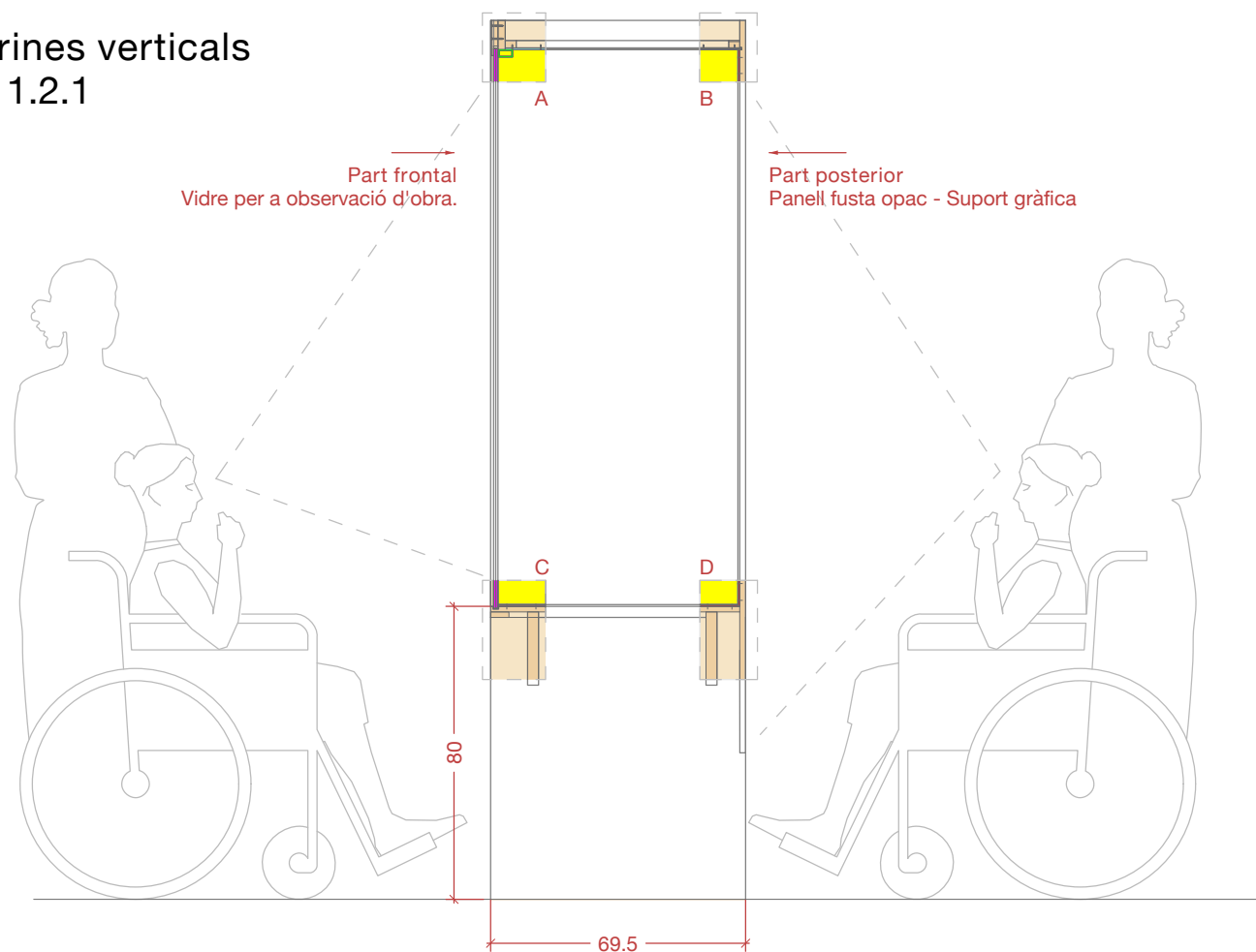
Secció Lateral
