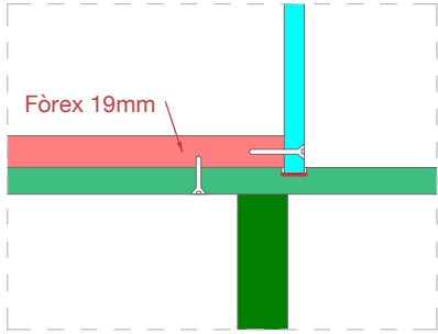
Detall A - Escala 1:5 Urna amb requeriments especials.
