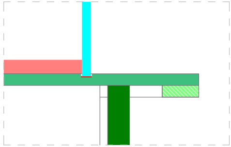
Detall C - Escala 1:5 Sistema constructiu sobre
