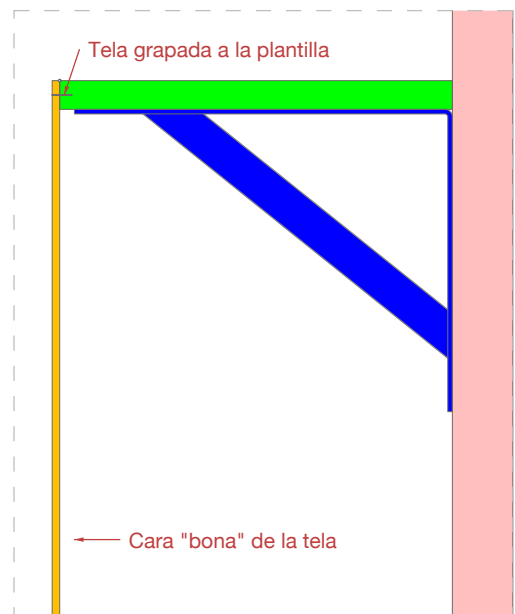
Detall A - Escala 1:2.5 Unió plantilla-cortina
