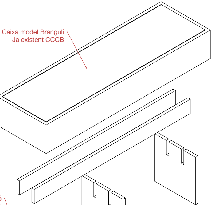
Potes de nova construcció DM 30 mm | Lacat a 3 capes
