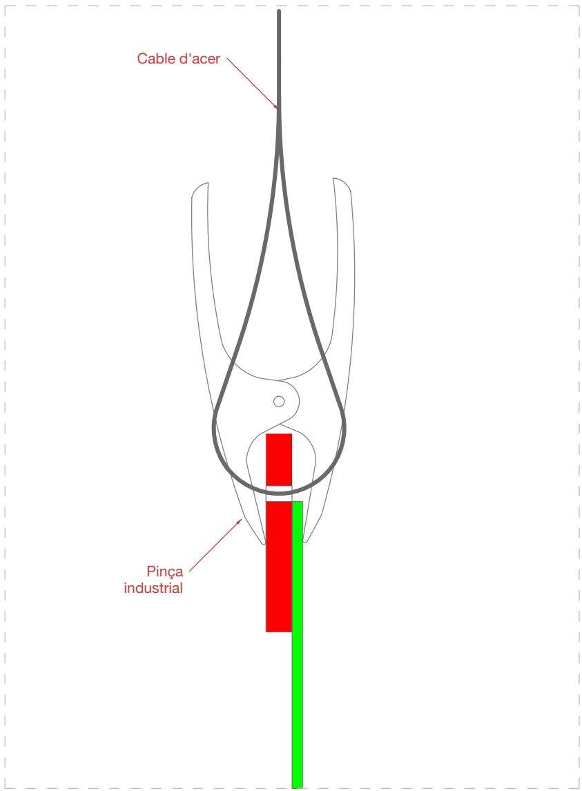
Detall A - Escala 1:1 Sistema de suspensió obra
