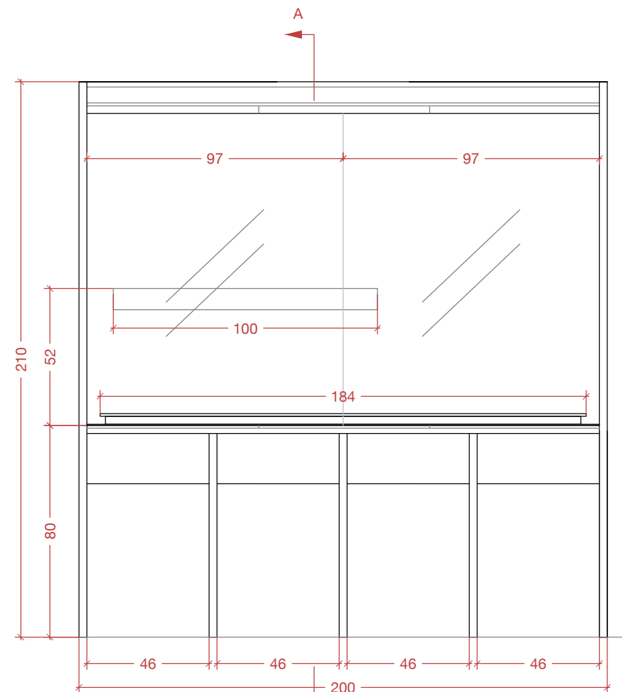
Alçat
