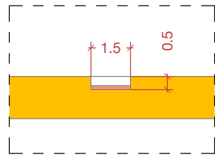
Detall D - Escala 1:2 Rebaix al sobre amb les mateixes dimensions que les urnes per a col·locar-hi espuma aïllant
