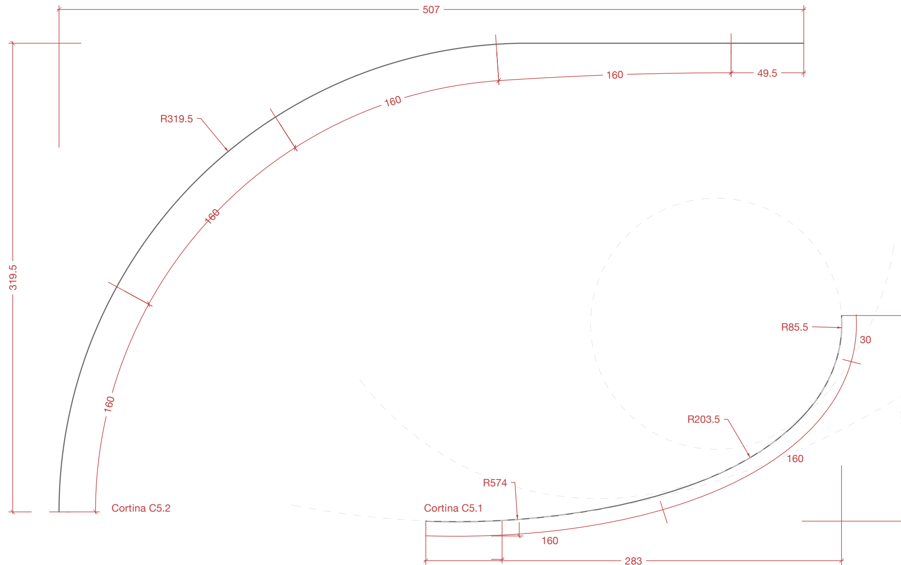
Detall A - Escala 1:1 Sistema de suspensió cortina
