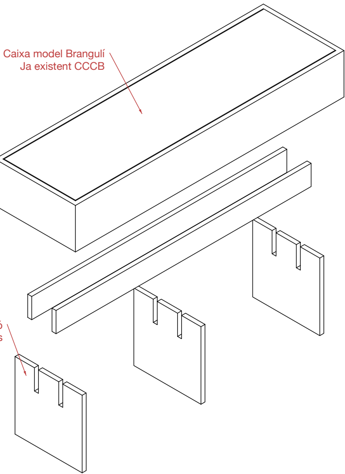
Vista isomètrica Explosionat
