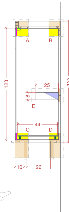
Secció Lateral
