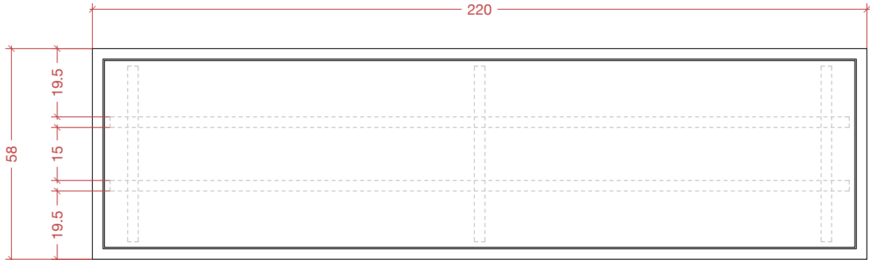
Planta
