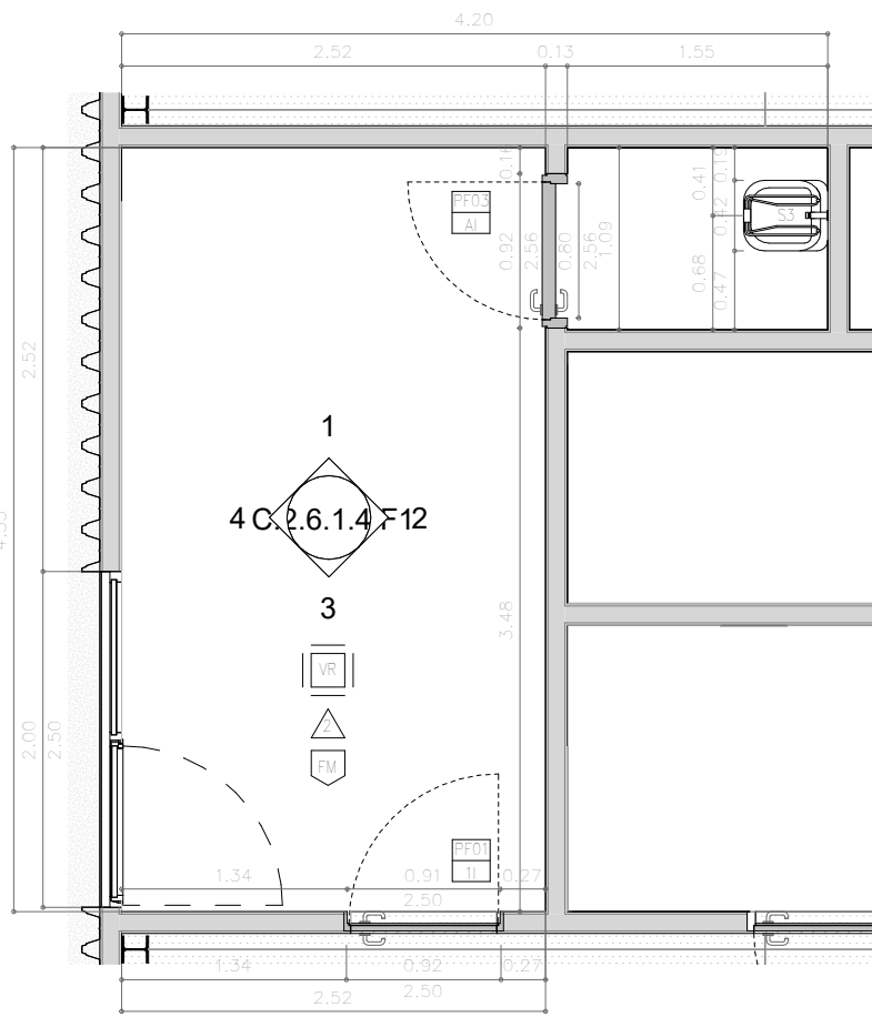
5 PLANTA BAIXA SALA D'INSTAL·LACIONS (+0.00) 1 : 50
