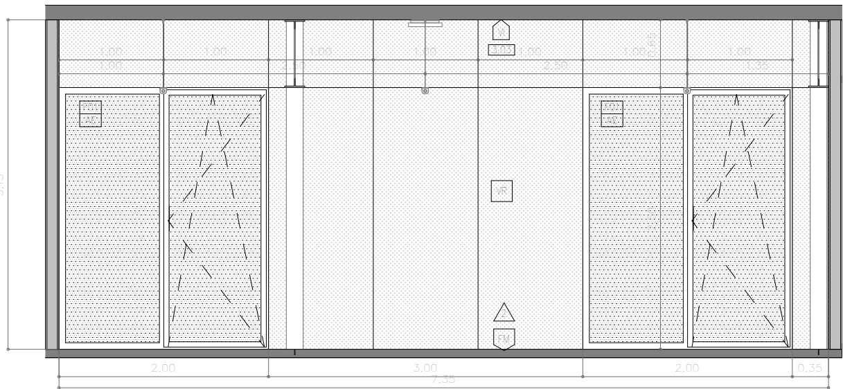
C.2.4.F2 ALÇAT 2 TALLER 1 : 50
