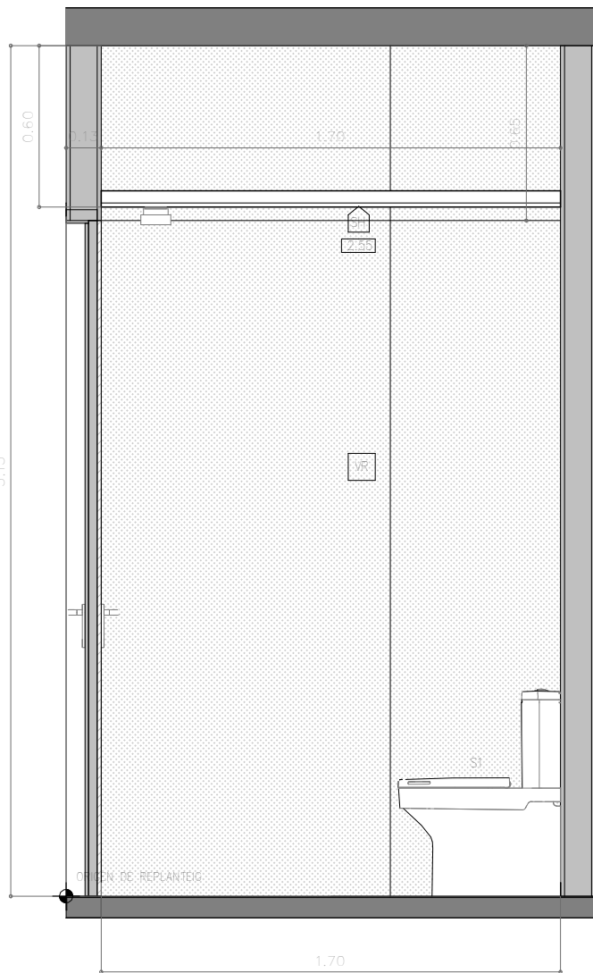
3 ALÇAT INTERIOR BANY 3 1 : 25
