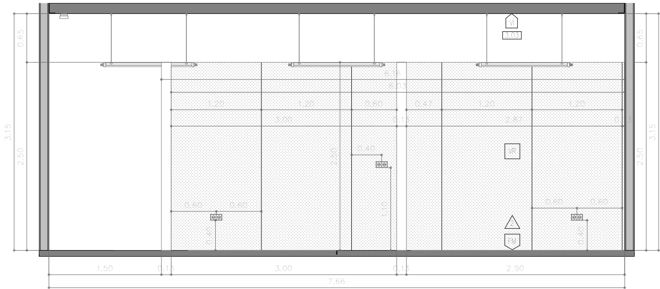
ALÇAT INTERIOR ADMINISTRACIÓ 6 1 : 50
