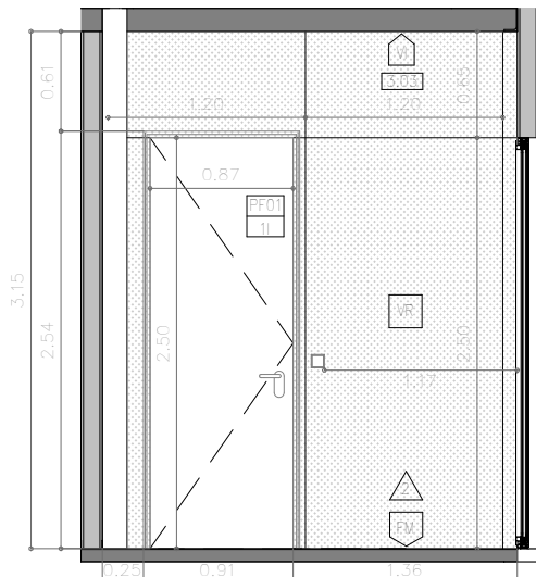
3 ALÇAT INTERIOR SALA D'INSTAL·LACIONS 3 1 : 50
