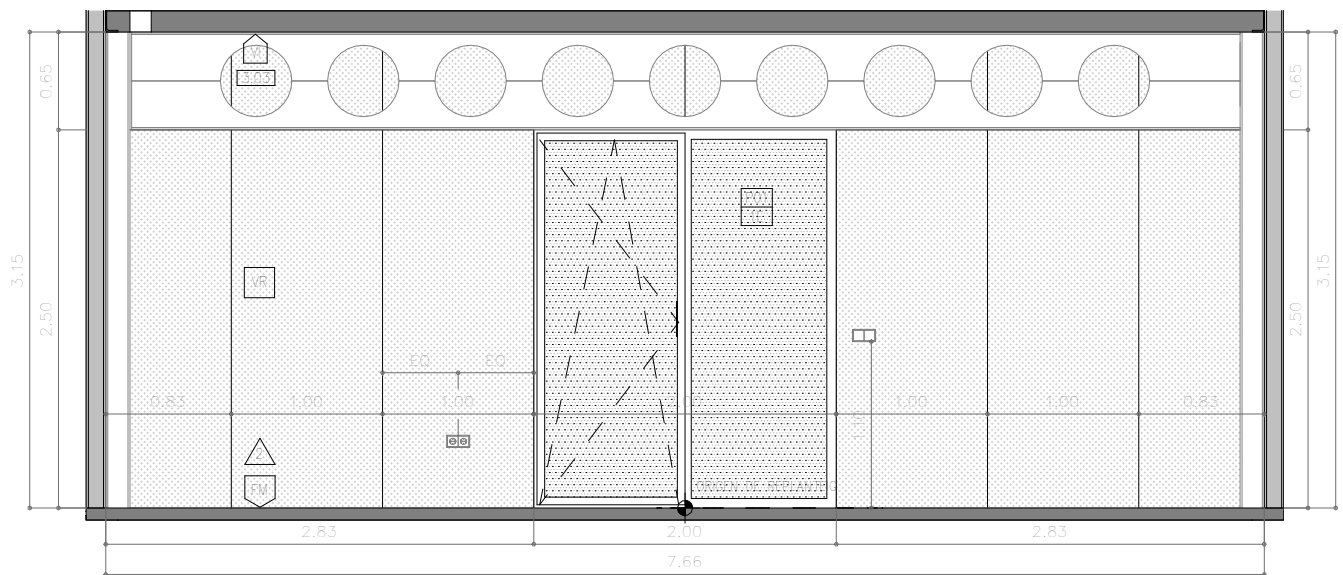
ALÇAT INTERIOR ZONA ADMINISTRATIVA 3
