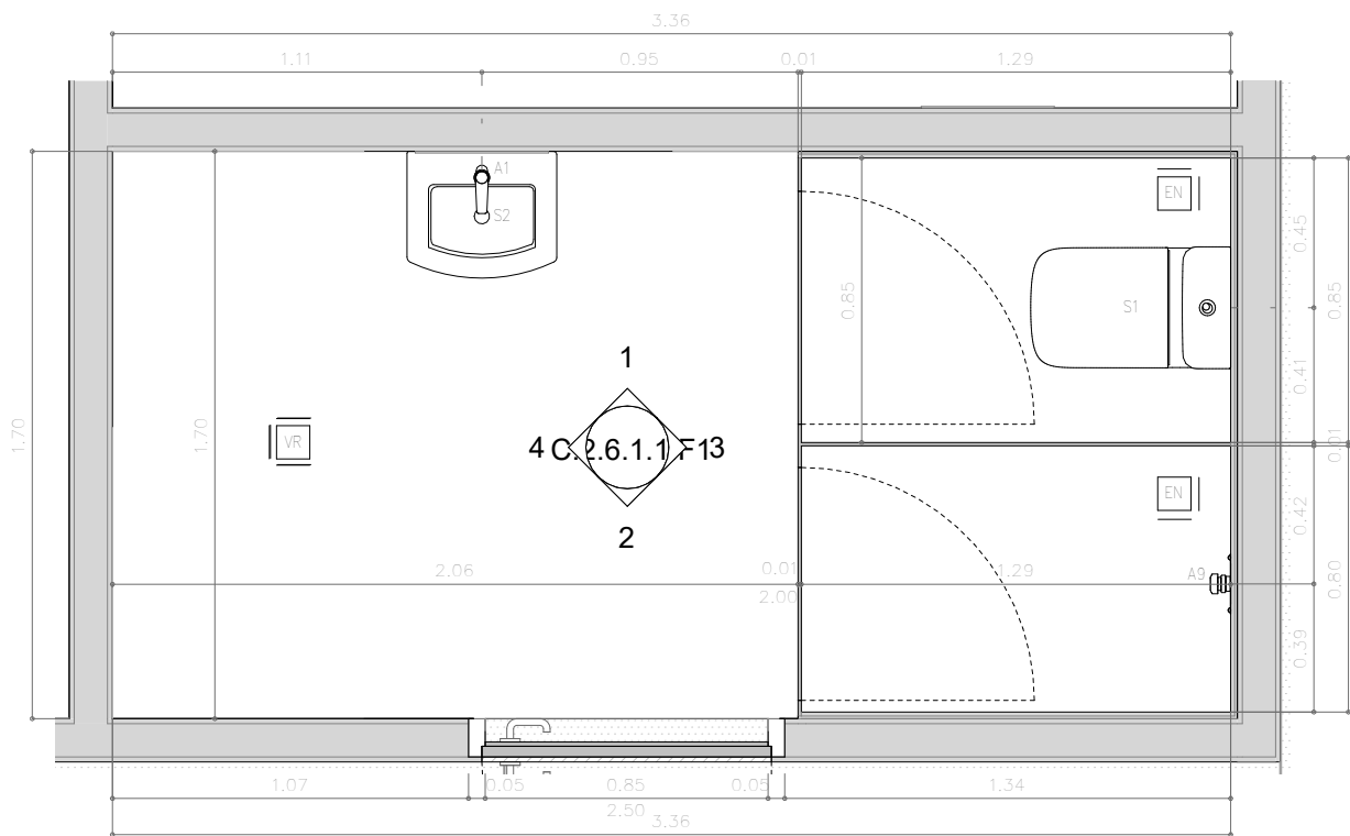
PLANTA BAIXA VESTUARIS (+0.00) 1 : 25
