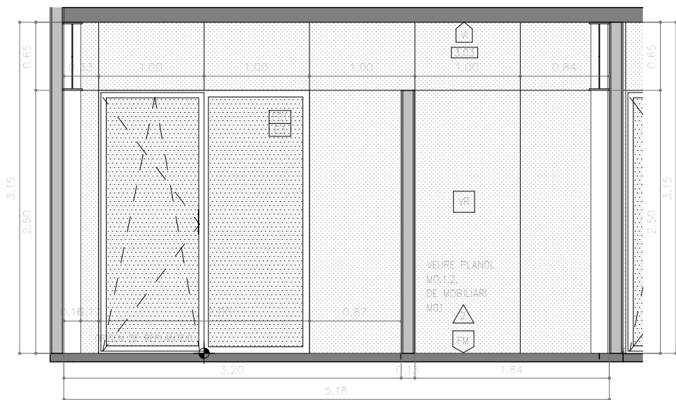
ALÇAT INTERIOR ZONA ADMINISTRATIVA 4
