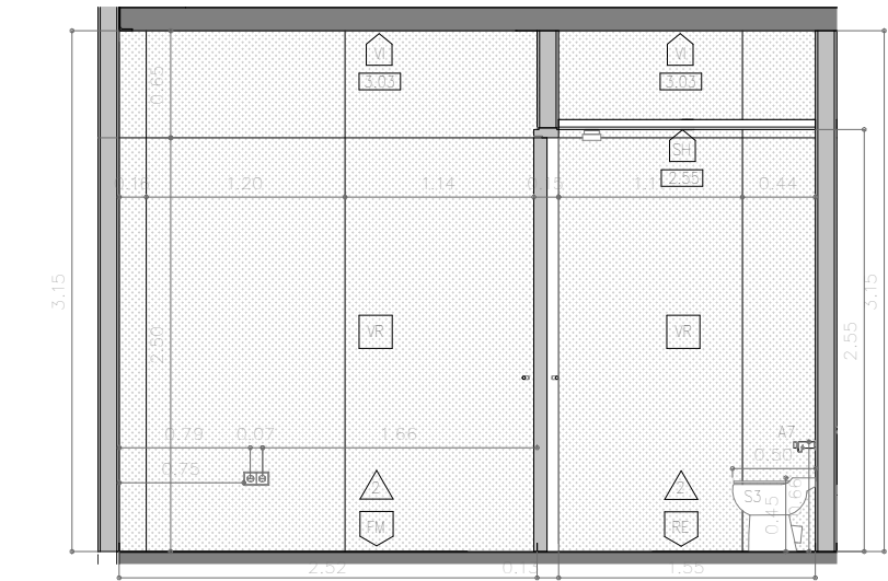
1 ALÇAT INTERIOR SALA D'INSTAL·LACIONS 1 1 : 50
