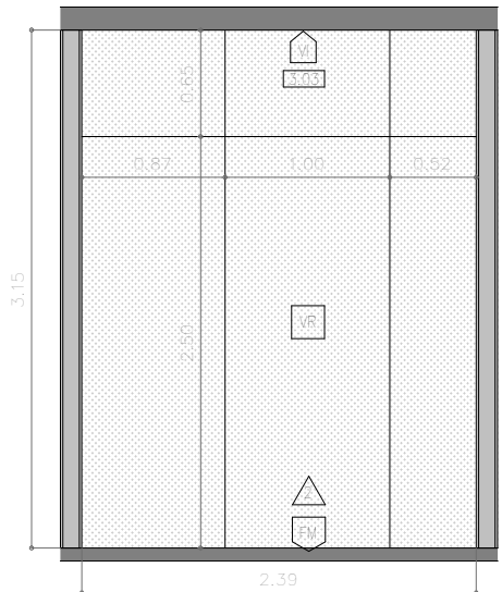
4 ALÇAT 4 MAGATZEM BOTIGA 1 : 50
