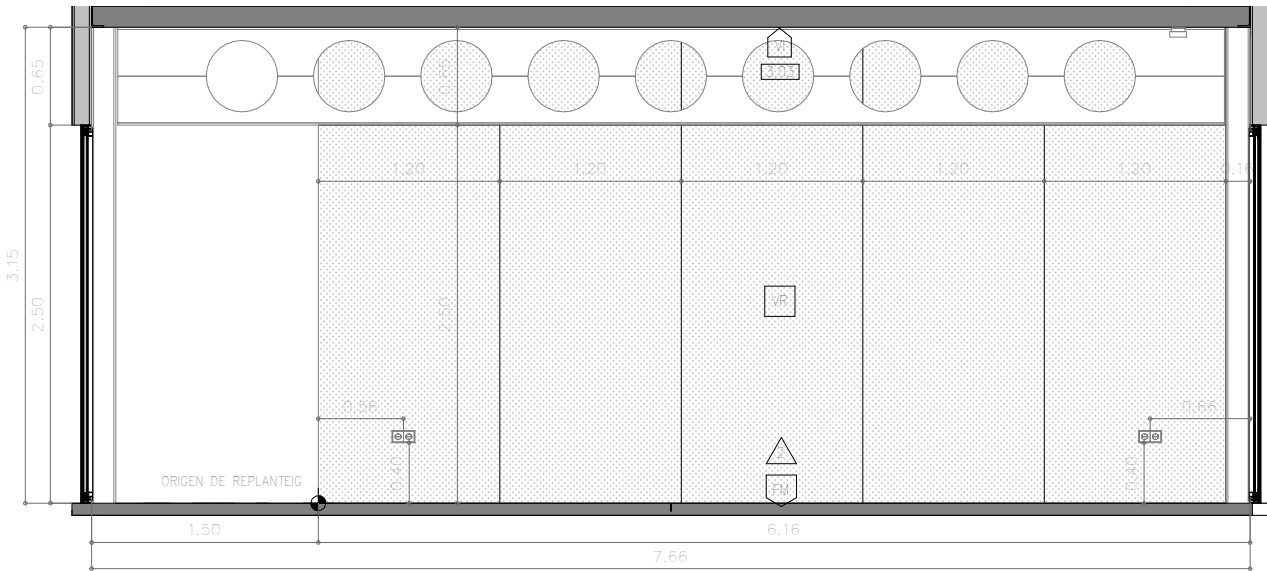
ALÇAT INTERIOR BOTIGA 4 1 : 50
