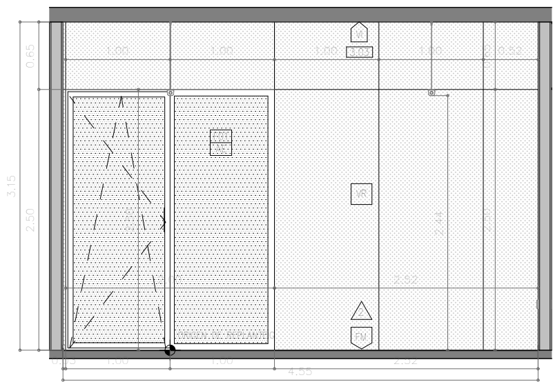
4 ALÇAT INTERIOR SALA D'INSTAL·LACIONS 4 1 : 50
