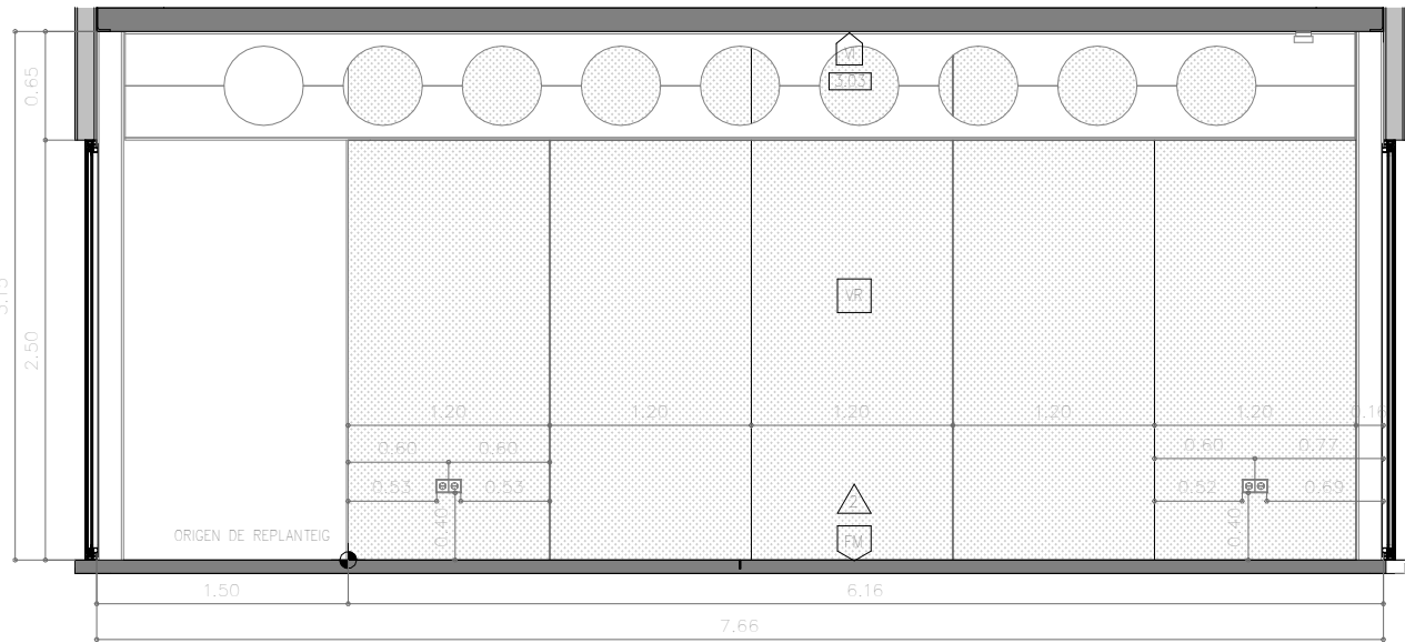
C.2.4.F2 ALÇAT 3 TALLER 1 : 50
