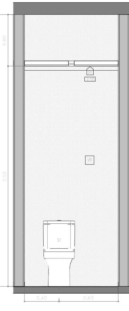
5 ALÇAT INTERIOR BANY 4 1 : 25
