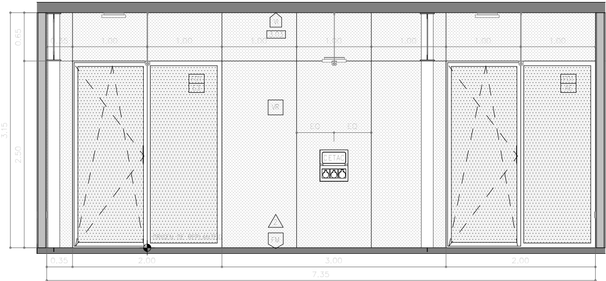
C.2.4.F2 ALÇAT 4 TALLER 1 : 50
