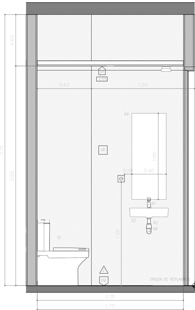
2 ALÇAT INTERIOR BANY 1 1 : 25
