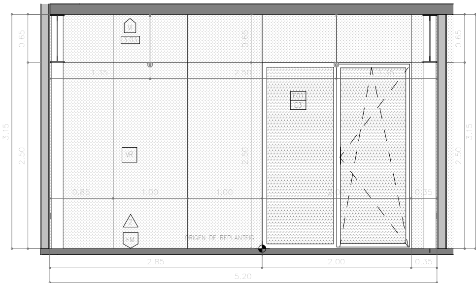
ALÇAT INTERIOR BOTIGA 2 1 : 50
