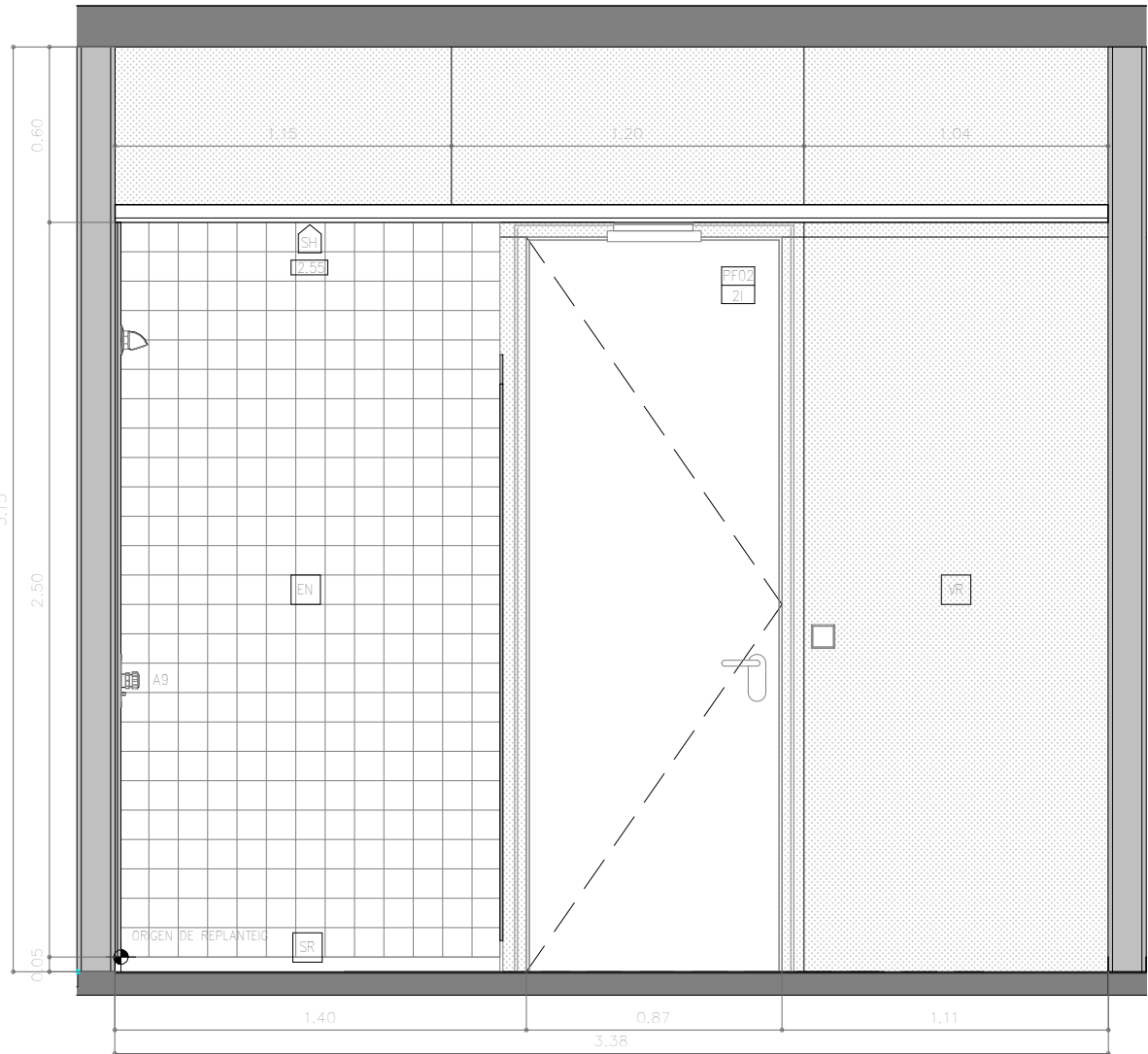
ALÇAT INTERIOR VESTUARIS 2 1 : 25
