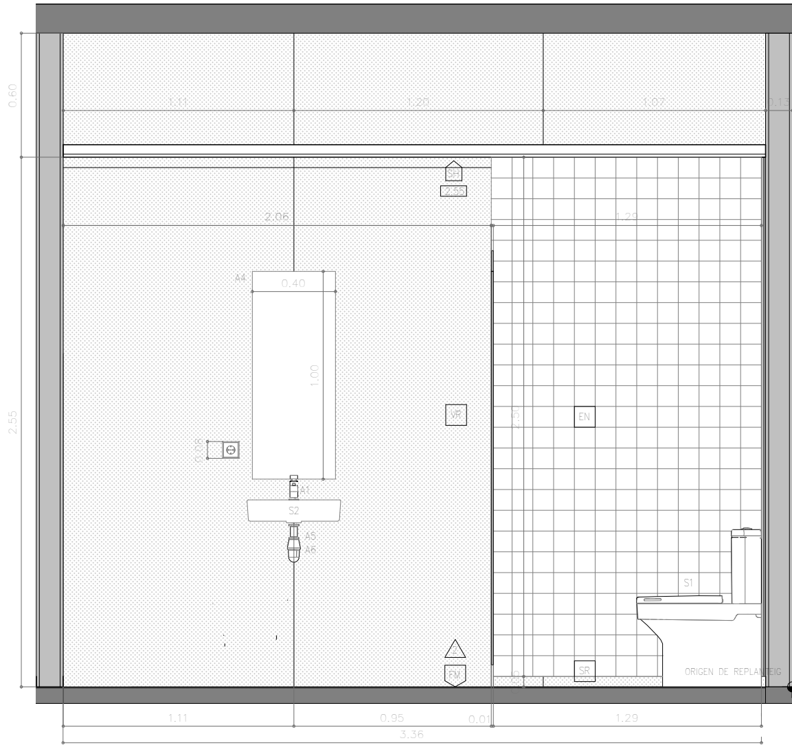
ALÇAT INTERIOR VESTUARIS 1 1 : 25
