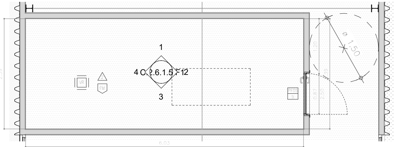
5 PLANTA BAIXA MAGATZEM BOTIGA (+0.00) 1 : 50
