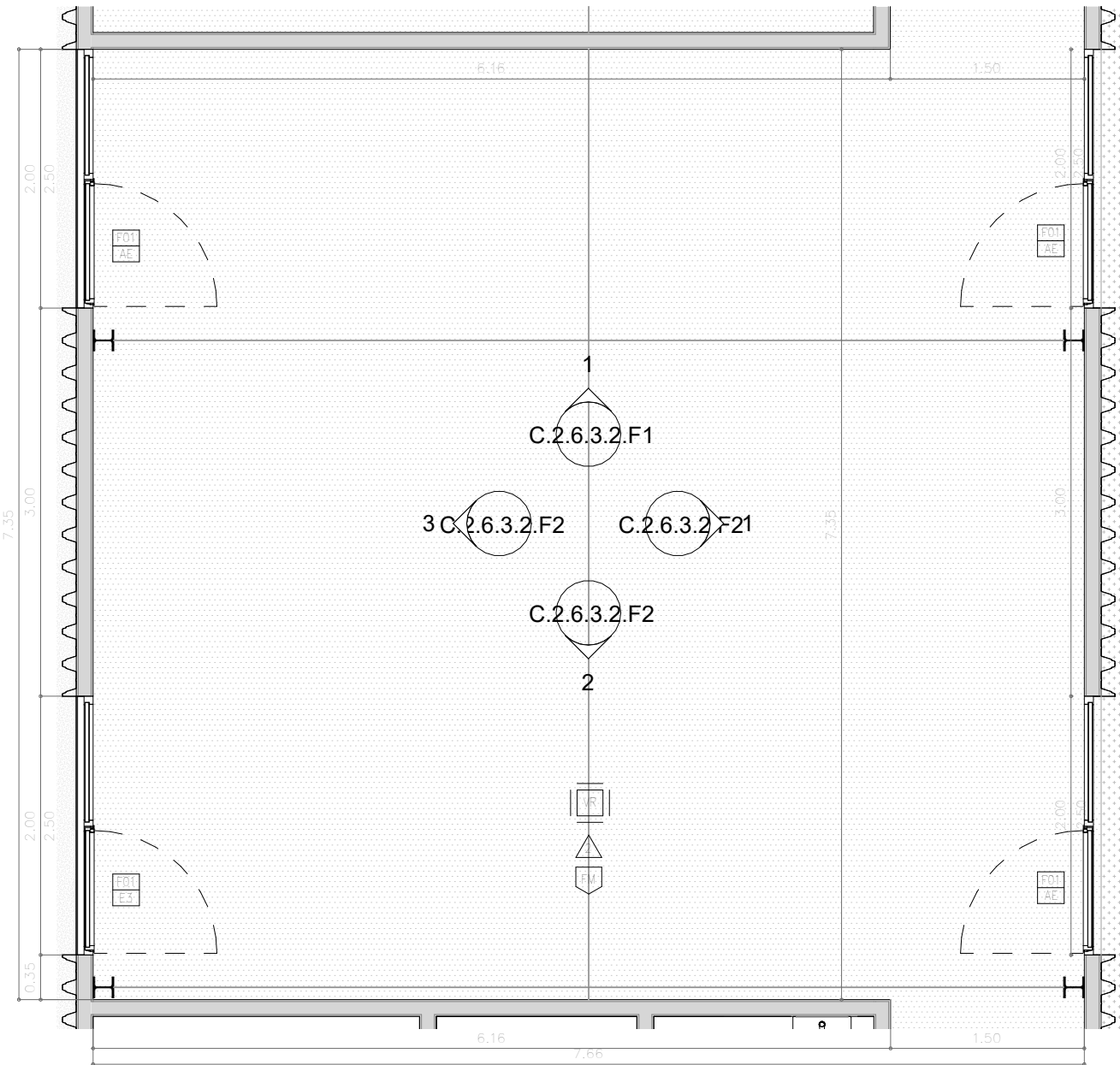
PLANTA TALLER (+0,00)
