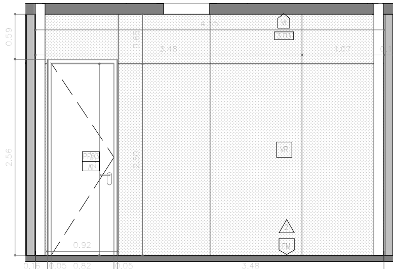
2 ALÇAT INTERIOR SALA D'INSTAL·LACIONS 2 1 : 50
