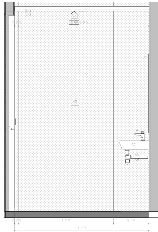
ALÇAT INTERIOR VESTUARIS 4 1 : 25
