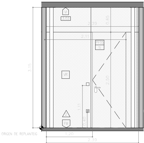
2 ALÇAT 2 MAGATZEM BOTIGA 1 : 50
