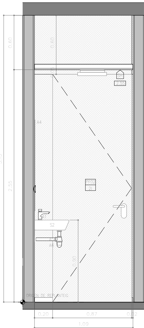
4 ALÇAT INTERIOR BANY 2 1 : 25
