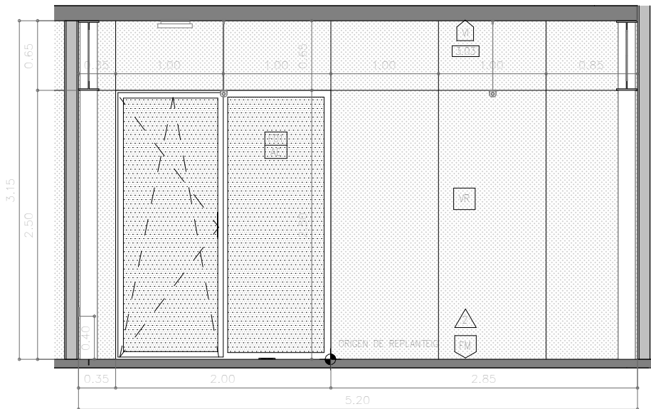
ALÇAT INTERIOR BOTIGA 3 1 : 50
