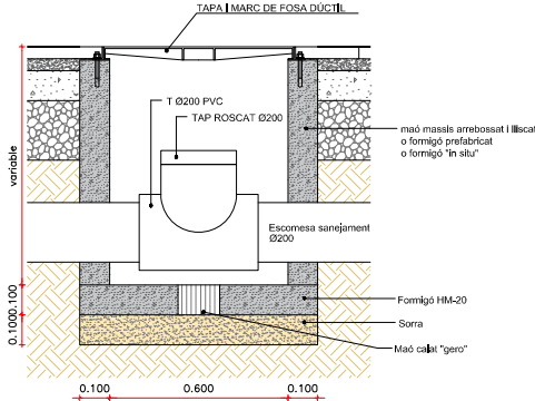
DETALL ESCOMESA SANEJAMENT esc 1/20
