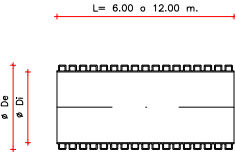
DETALL CANONADA PEAD CORRUGAT EXTERIOR esc 1/20
