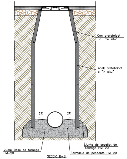
DETALL POU CLAVEGUERAM esc 1/40
