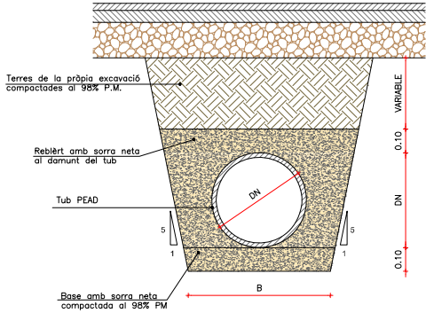
DETALL RASA CLAVEGUERAM esc 1/20
