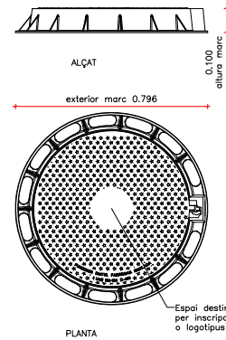
DETALL TAPA I MARC AMB TANCA DE BLOQUEIG I JUNTA D'INSONORITZACIÓ esc 1/20
