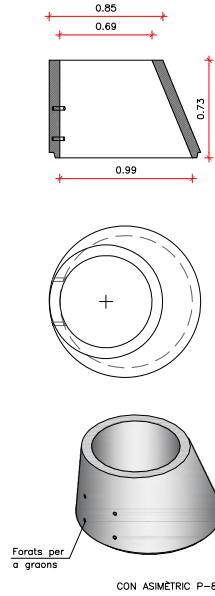
DETALL CON PREFABRICAT esc 1/40
