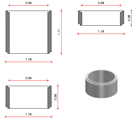
DETALL ANELLS PREFABRICATS esc 1/40
