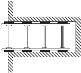
RASA AMB APUNTALAMENT PER A SOBRECÀRREGA
