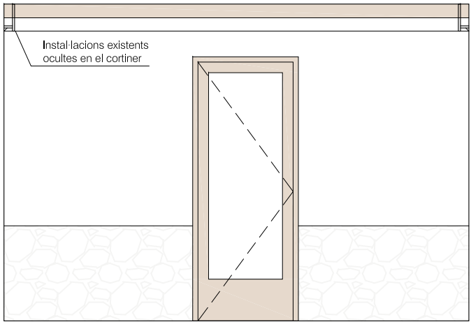
SECCIÓ TRANSVERSAL 2
