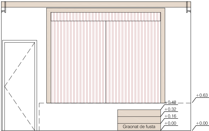
SECCIÓ TRANSVERSAL 1
