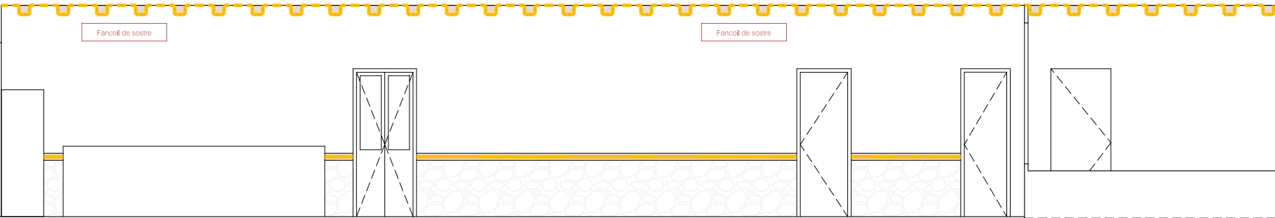
SECCIÓ LONGITUDINAL 1
