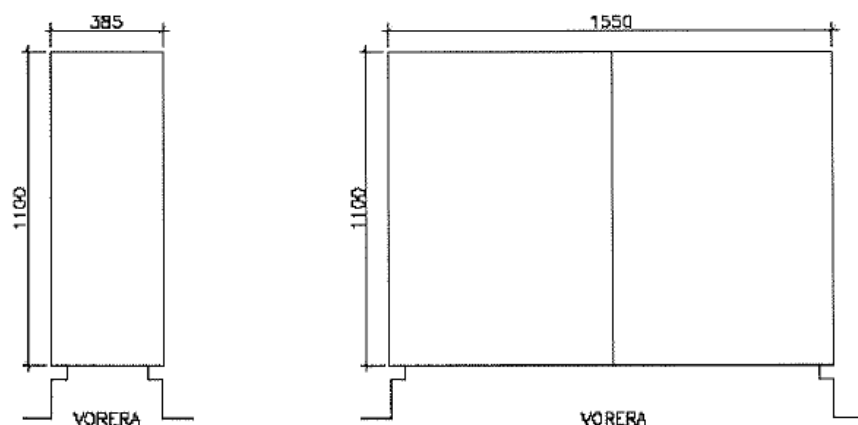
Figura 1 : Armari d'intempèrie TIPUS 1
