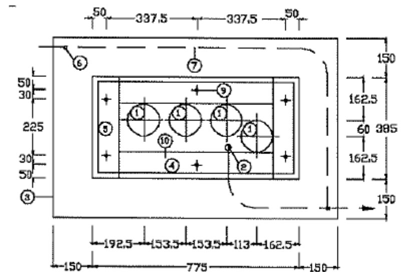
Figura 4: Esquema basament armari Tipus 1
