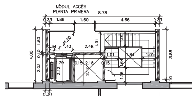
PLANTA PRIMERA
