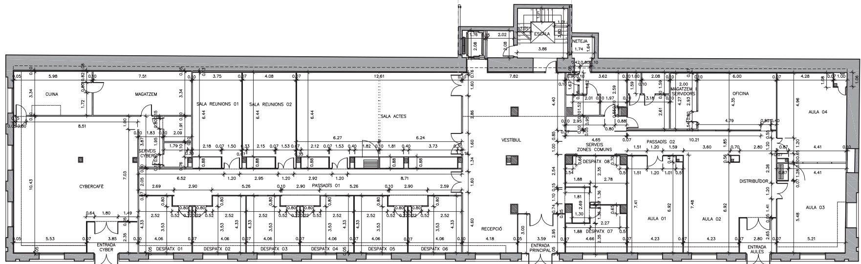
PLANTA BAIXA
