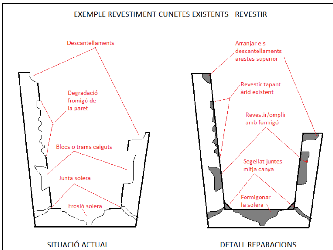
Imatge 2: Croquis cuneta a reparar.
