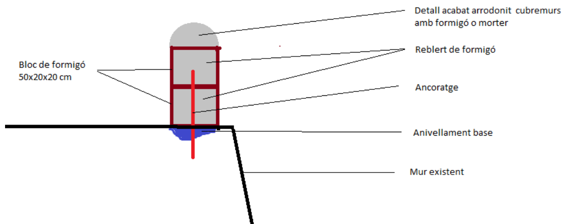
Imatge 1: Croquis mur guardabalast sobre mur existent.
