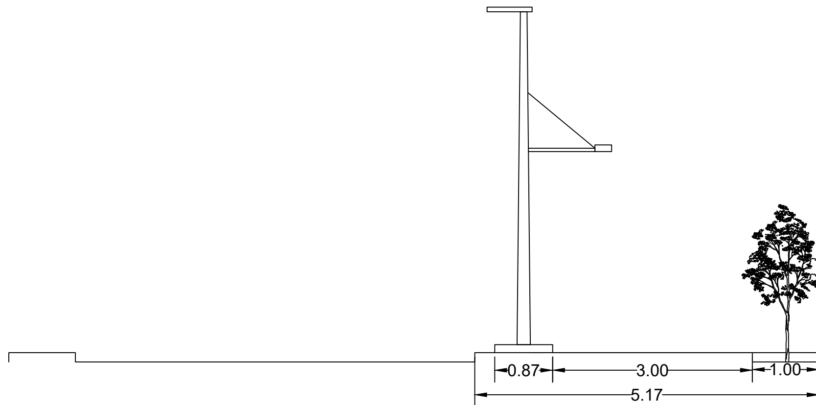
SECCIO DEL CARRER ACTUAL
