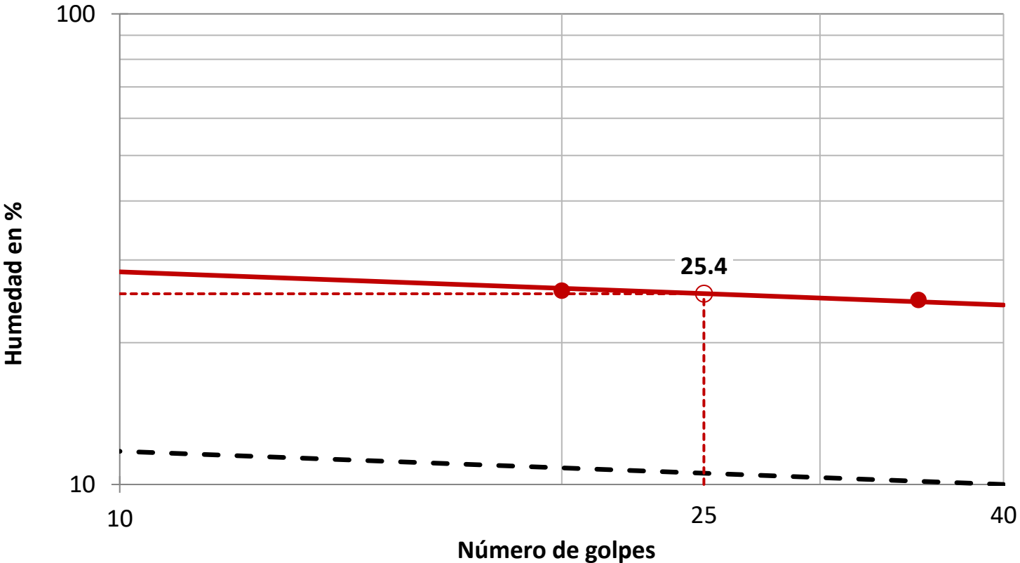
Gráfica límite líquido (LL)
