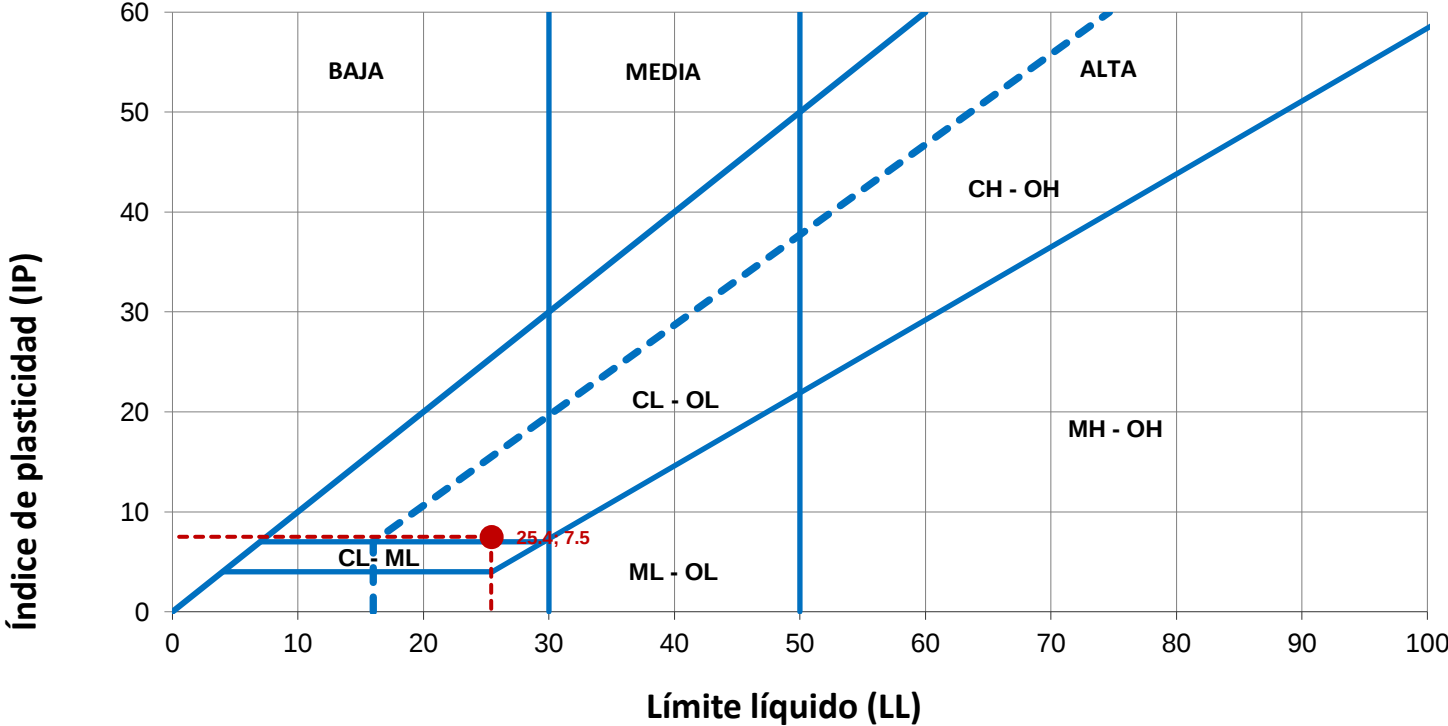
Gráfica de plasticidad de Casagrande (USCS)
