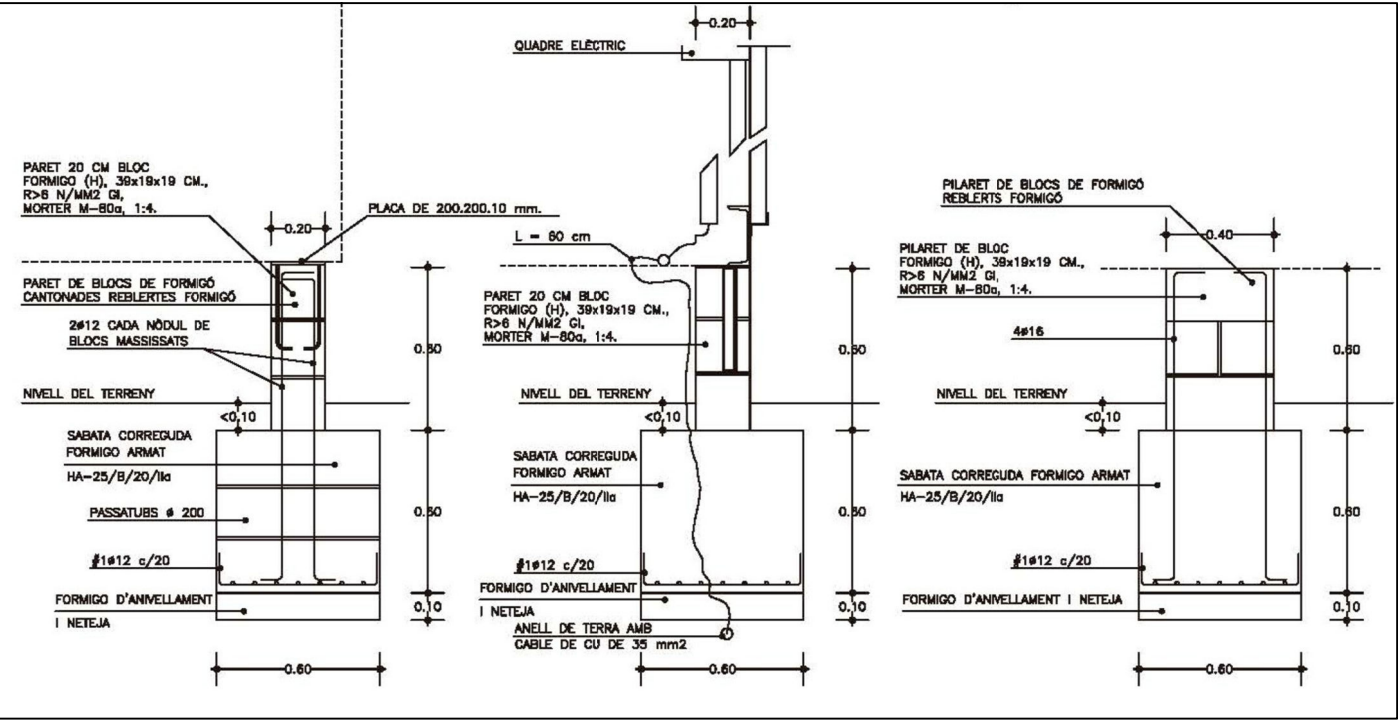
DETALLS CONSTRUCTIUS FONAMENTS
