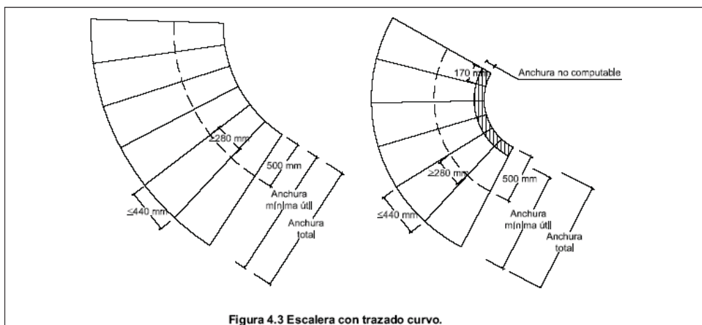
Figura 4.3 Escalera con trazado curvo.
