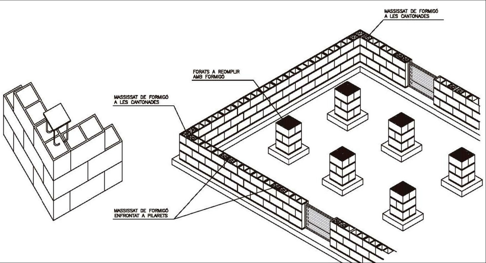
DETALLS CONSTRUCTIUS FONAMENTS
