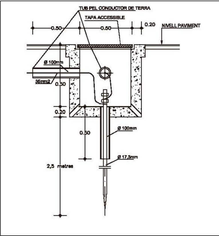
DETALLS CONSTRUCTIUS TOMA DE TERRA
