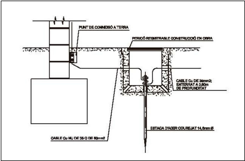
DETALLS CONSTRUCTIUS TOMA DE TERRA
