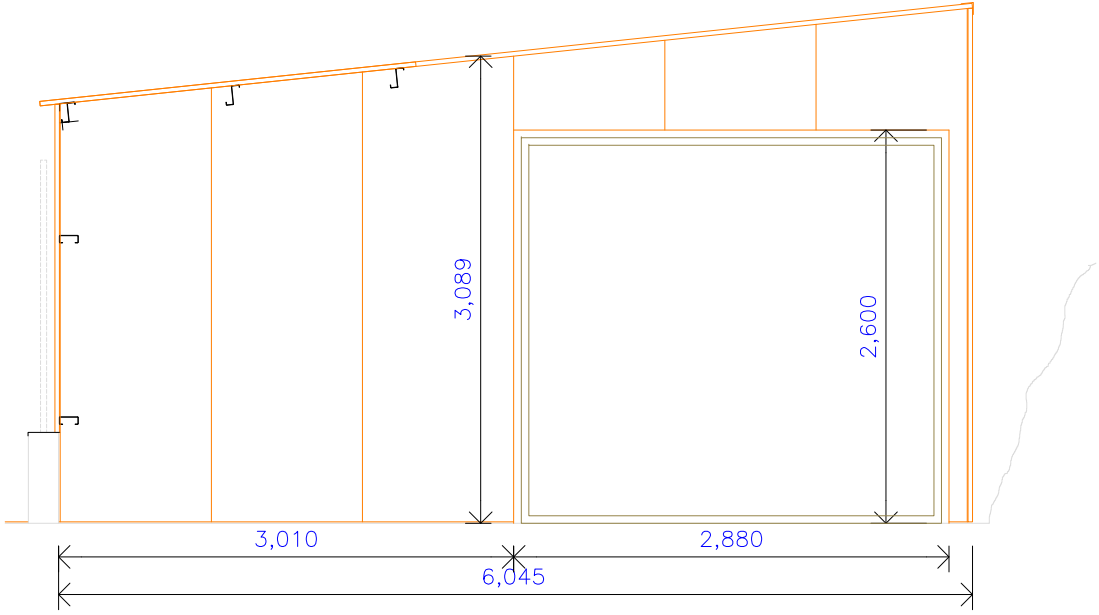
VISTA FRONTAL B-B
