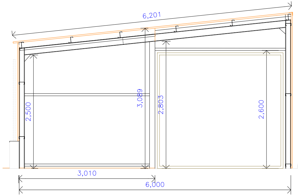
SECCIÓ B-B
