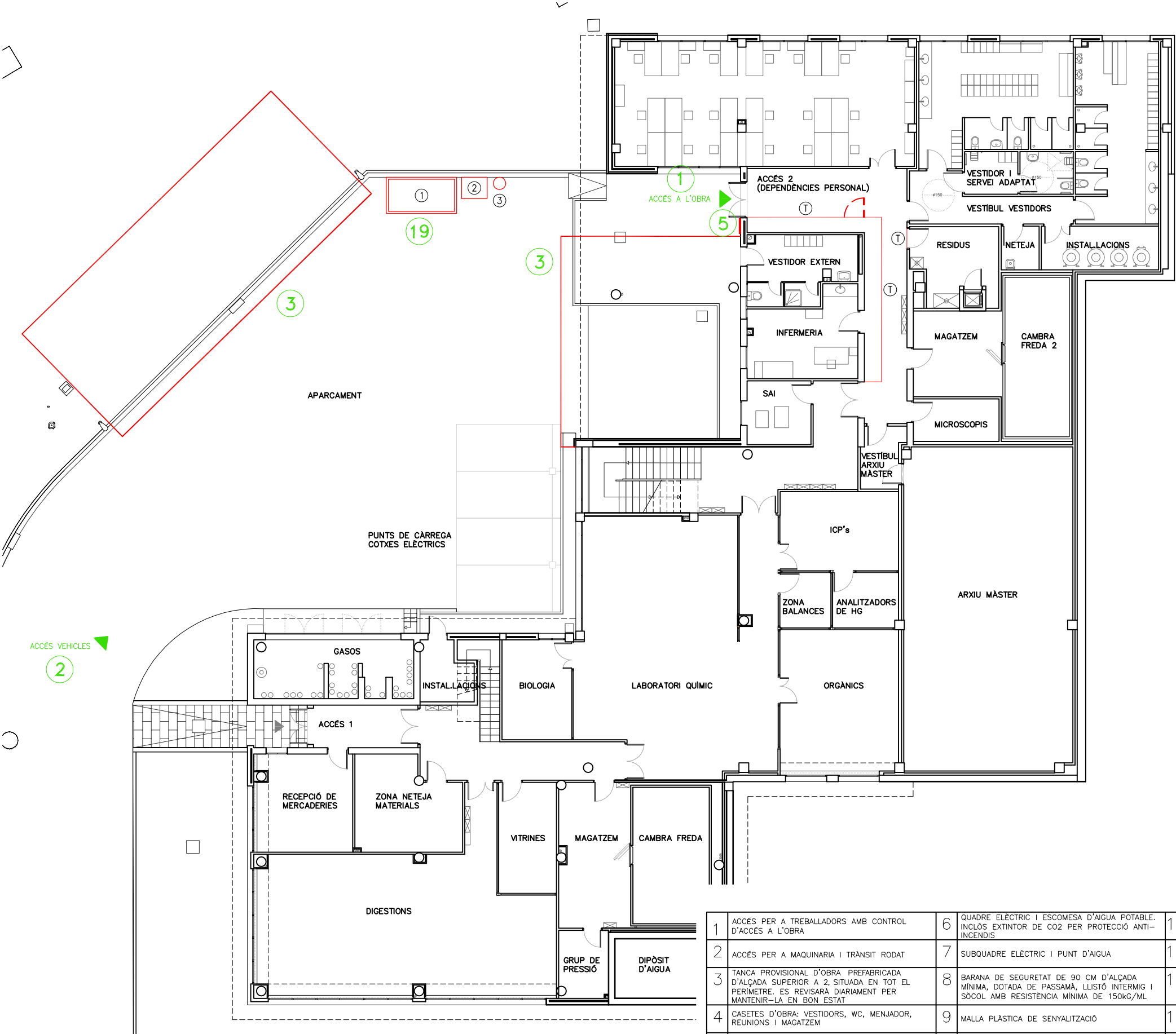
PLANTA SOTERRÀNIA. ESTAT ACTUAL A3 E 1:200
