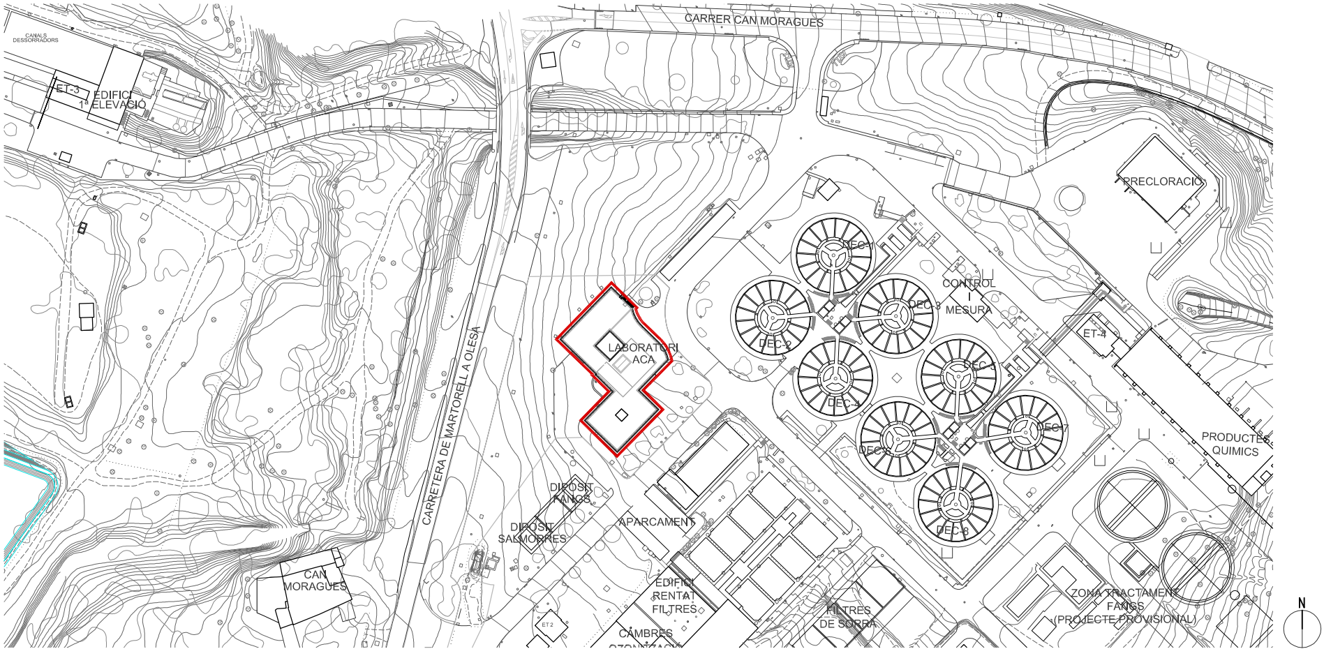
PLÀNOL DE L'EMPLAÇAMENT A3 E 1:2000
