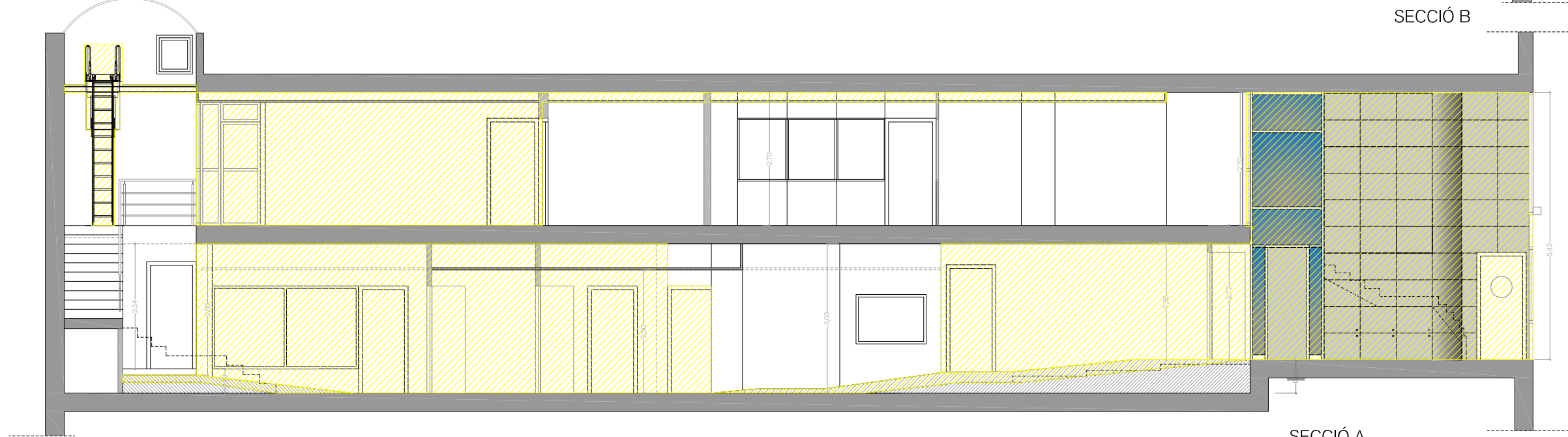
SECCIÓ A
