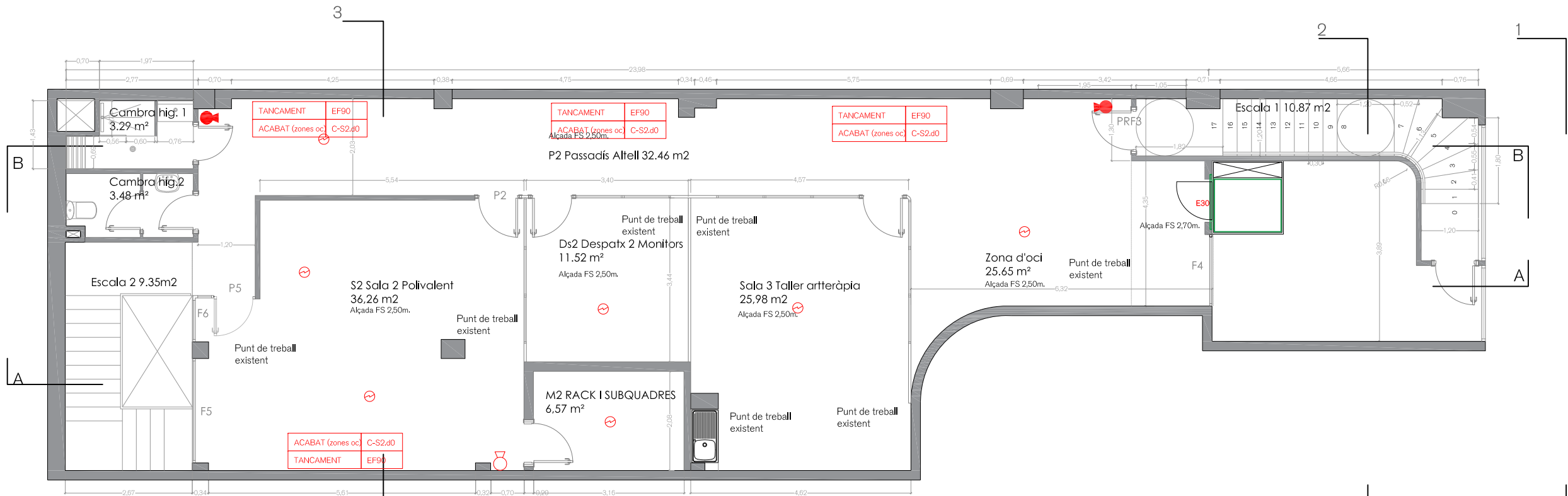
PLANTA ALTELL
