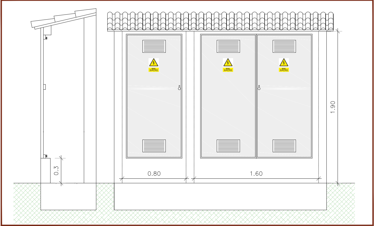
DETALL ARMARI ENCASTAT EN MUR EXISTENT INST. ENLLAÇ (CGP + MÒDUL COMPTADOR DE MESURA INDIRECTA TMF10) E: 1/25
