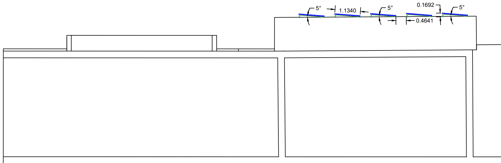
SECCIÓ A-A'
