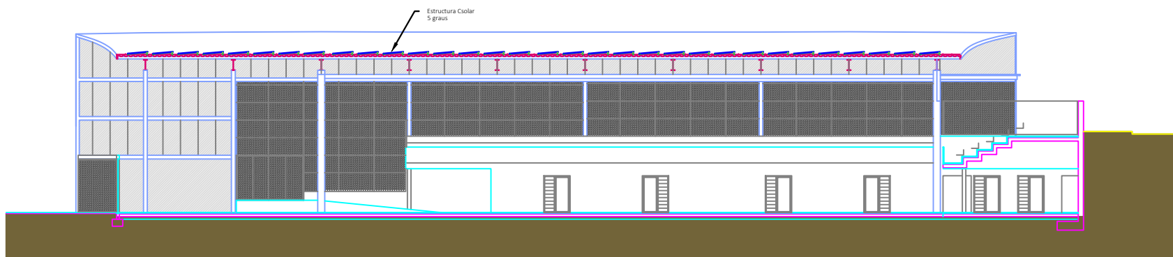
SECCIÓ A-A'
