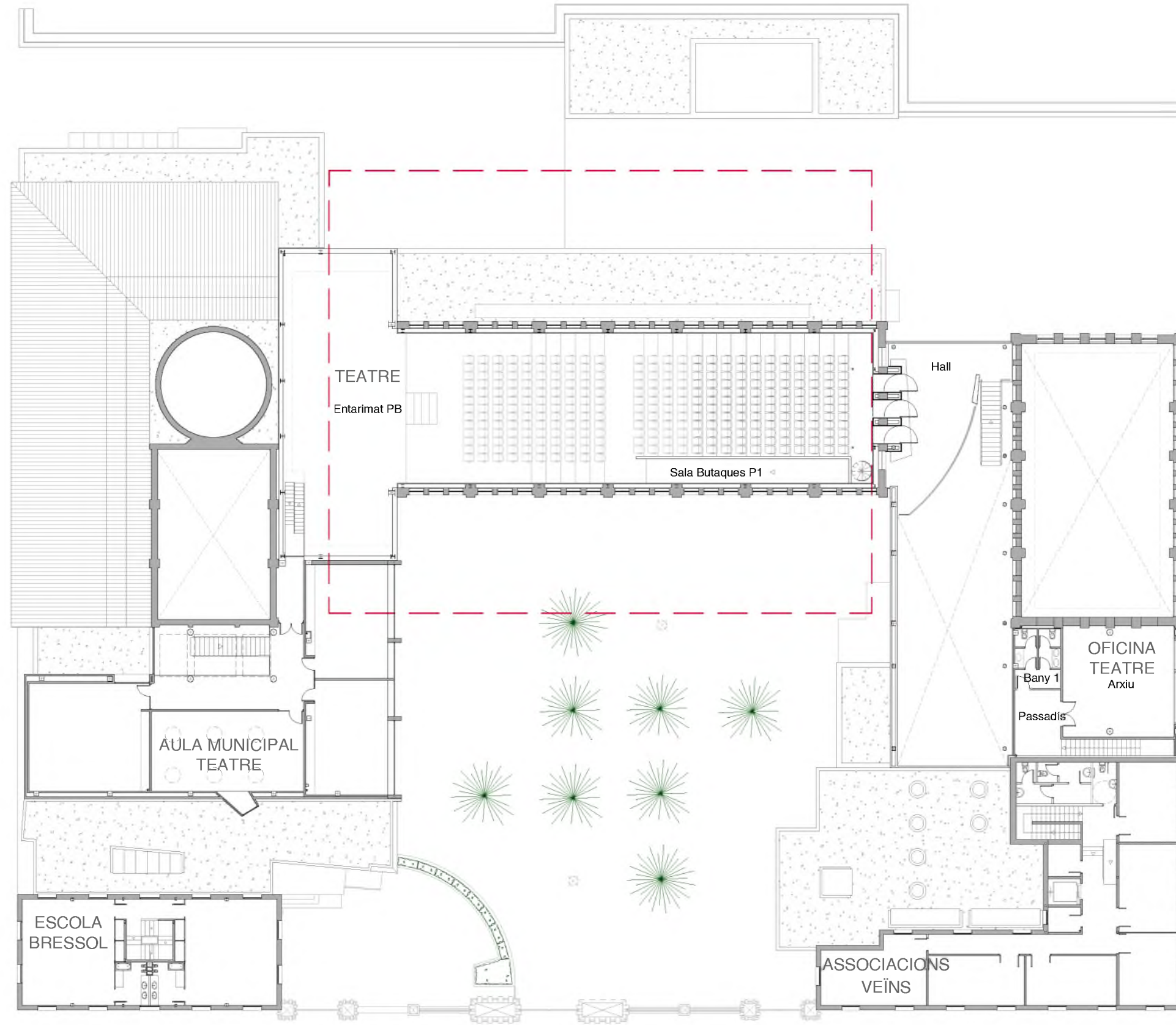
Planta primera
