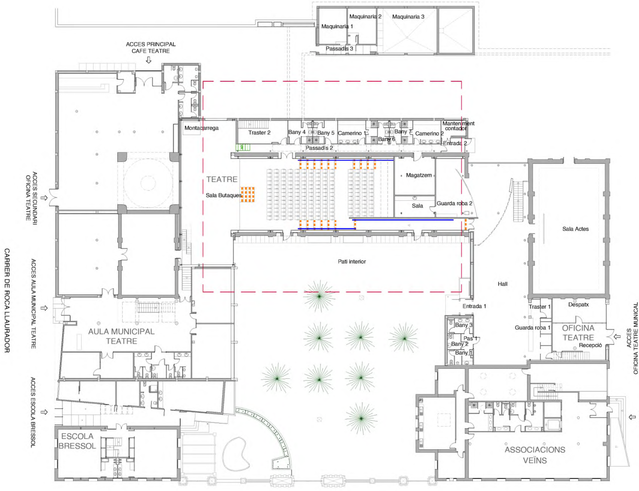
Planta baixa
