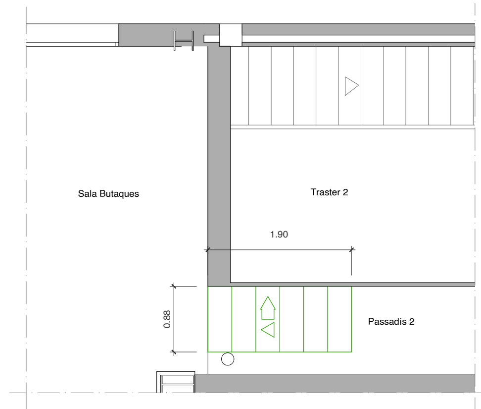
Planta
