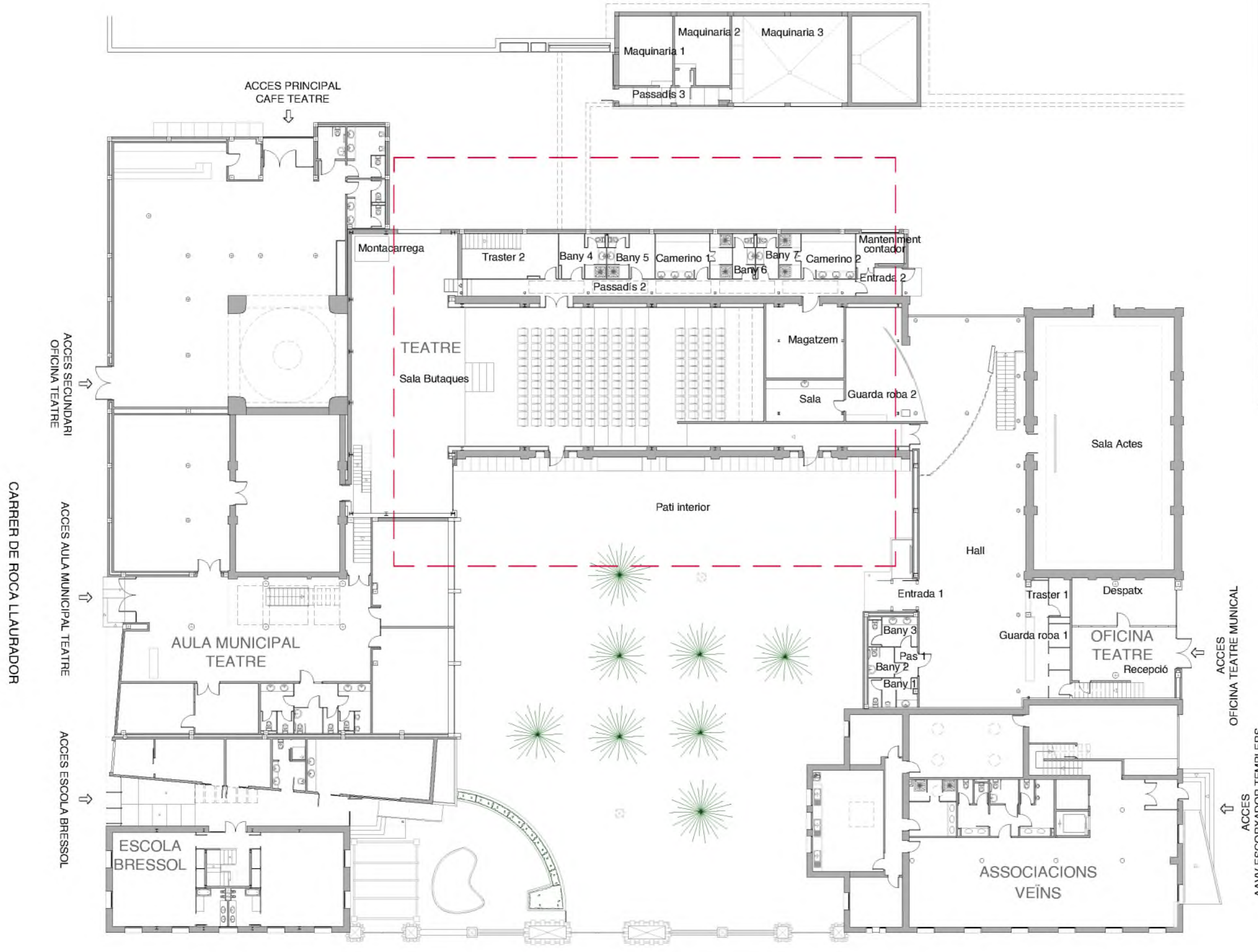
Planta baixa
