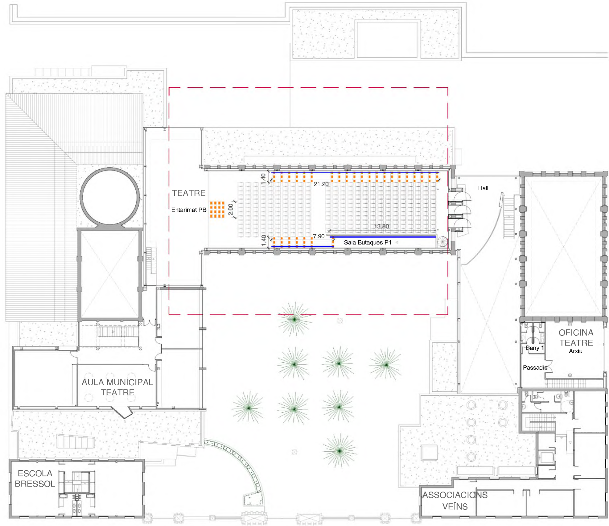
Planta primera
