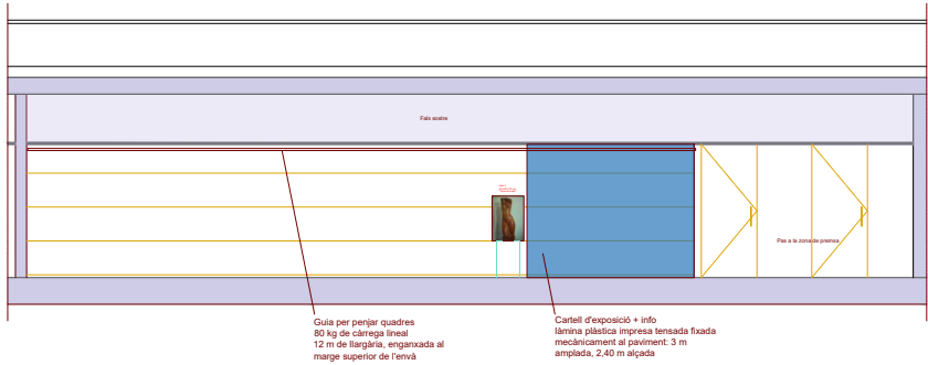
ALÇAT EST (D'AVANT ASCENSORS)
