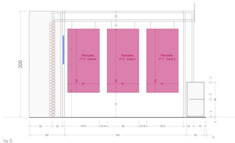
Plànol 6- Secció longitudinal
