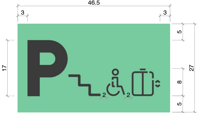
S-RE24 (Model 3) Vinil "Tipus acés" sobre xapa metàl·lica galvanitzada - Proposta
