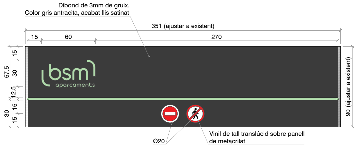
FRONTAL SORTIDA AV. DE LA REINA MARIA CRISTINA (R2)
