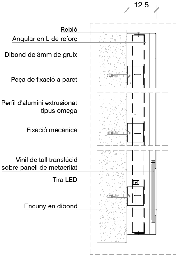
DETALL EN SECCIÓ DEL FRONTAL
