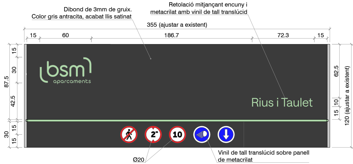
FRONTAL ENTRADA AV. DE LA REINA MARIA CRISTINA (R1)
