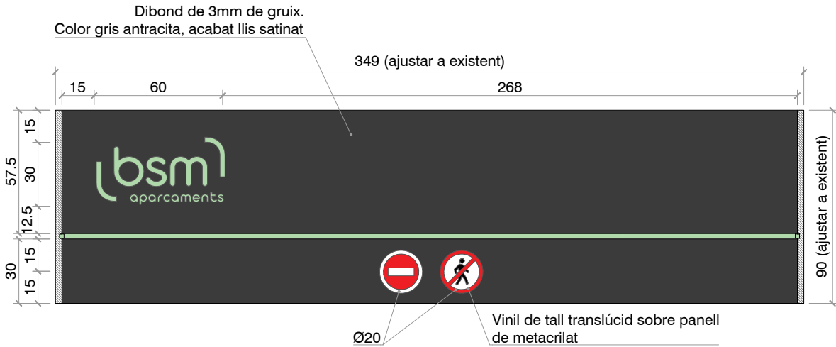
FRONTAL SORTIDA AV. DE RIUS I TAULET (R4)
