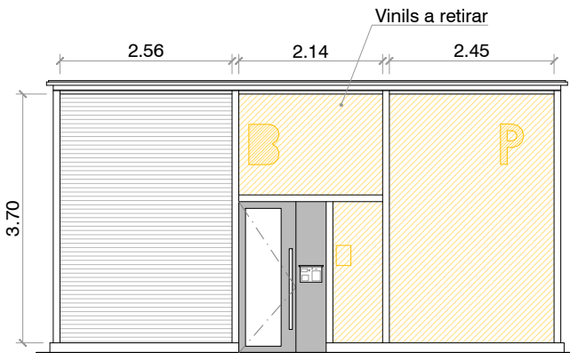
ESTAT ACTUAL (E.PN-1)
