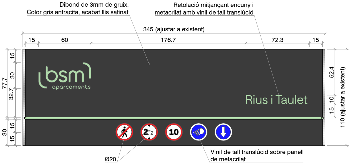
FRONTAL ENTRADA AV. DE RIUS I TAULET (R3)
