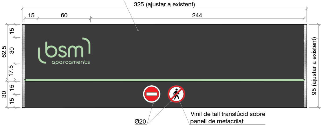
FRONTAL SORTIDA C/FLOS I CALCAT (R2)
