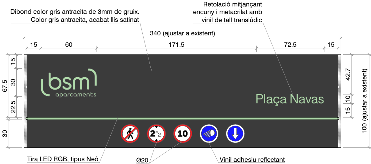
FRONTAL ENTRADA C/JAUME FABRE (R1)
