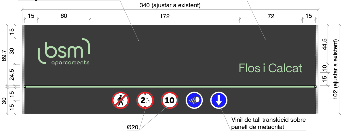
FRONTAL ENTRADA C/FLOS I CALCAT- GRAN VIA DE CARLES III (R3)
