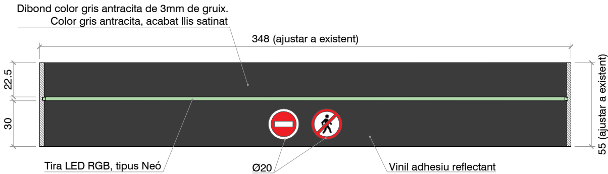
FRONTAL SORTIDA C/TEODOR BONAPLATA (R2)
