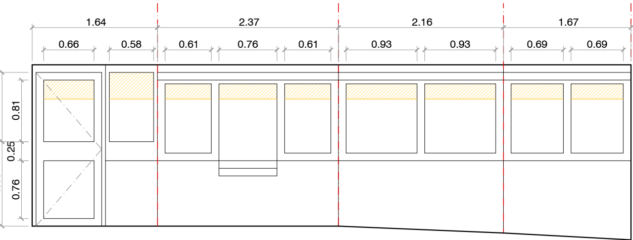
ESTAT ACTUAL E 1/50
