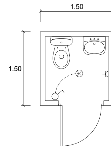
MÒDUL WC
