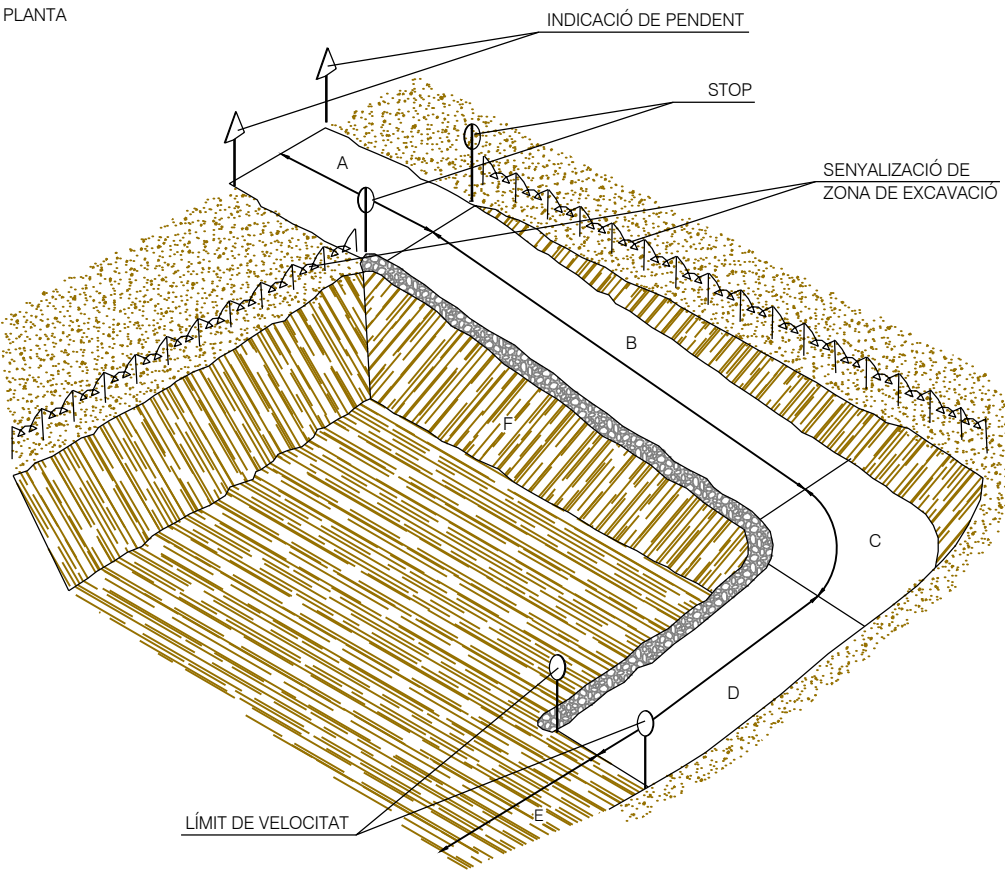
PLANTA
