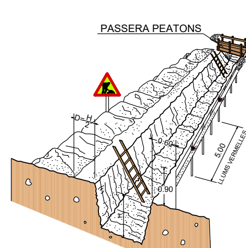
PROTECCIÓ EN RASES
