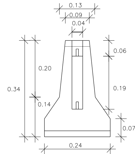
ALÇAT TRANSVERSAL
