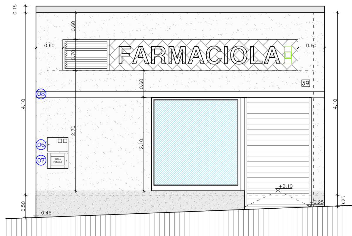
FAÇANA Av DON ÁLVARO
