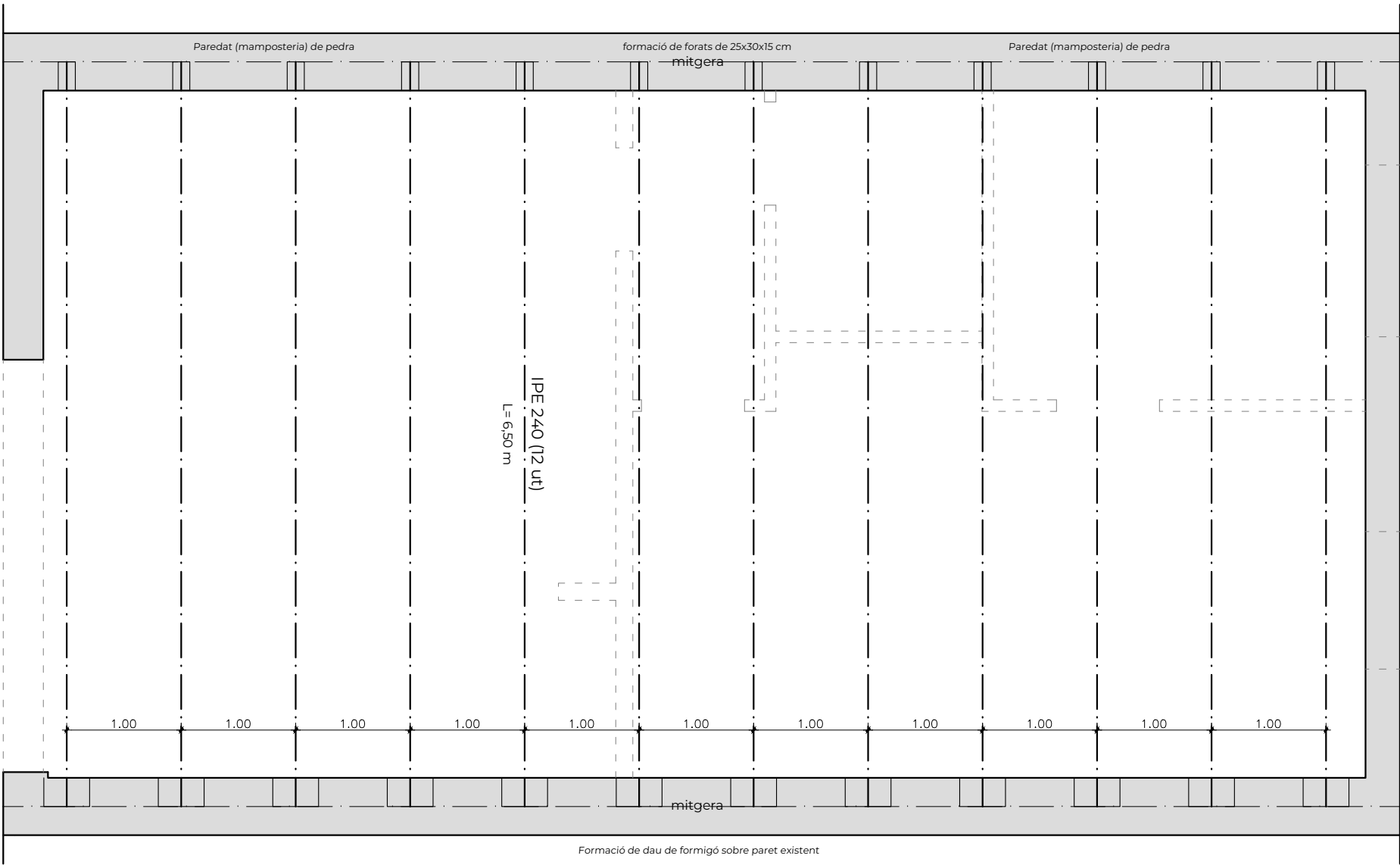
PLANTA ESTRUCTURA BIGUES
