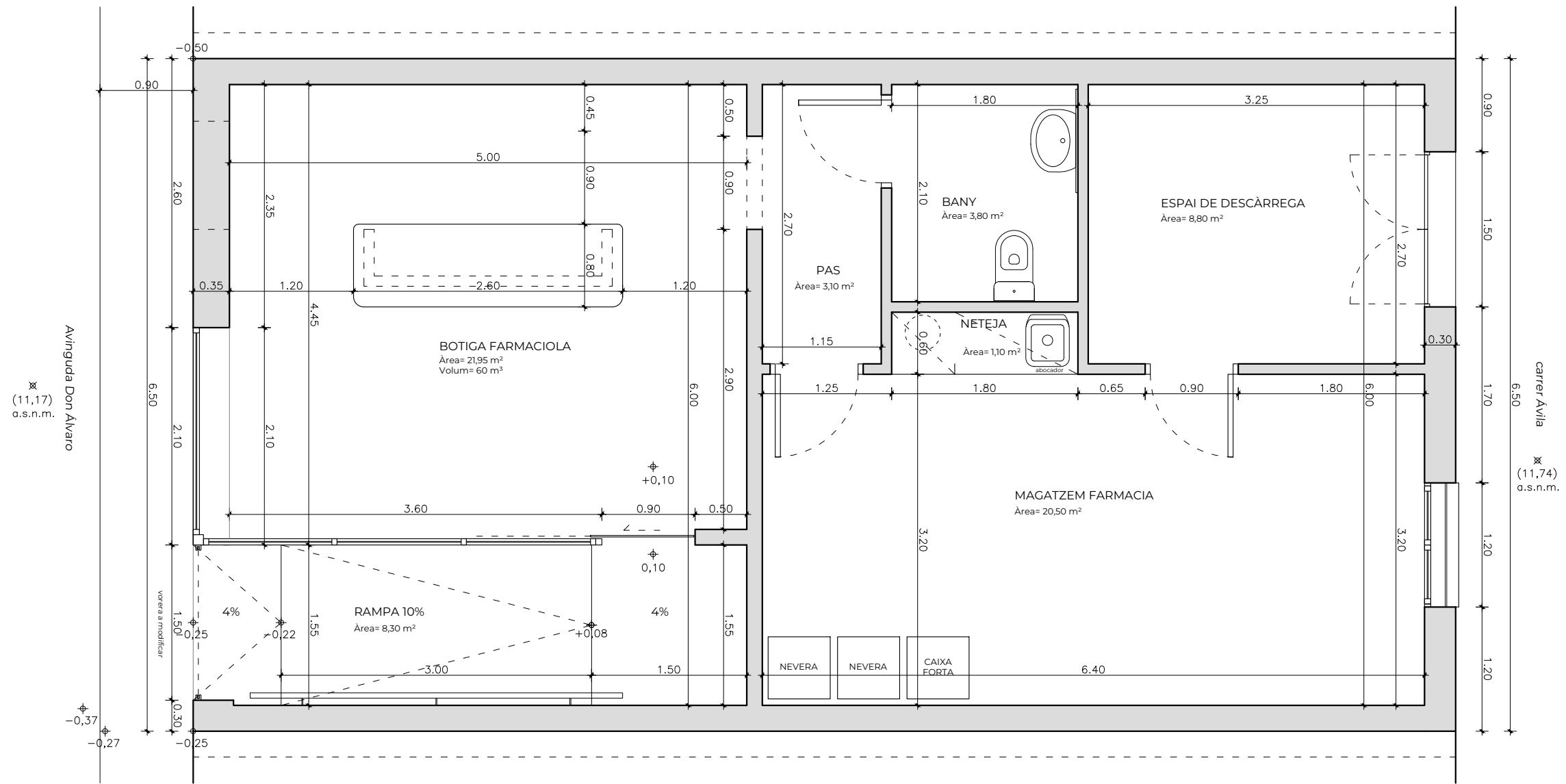
PLANTA COTES I SUPERFÍCIES
