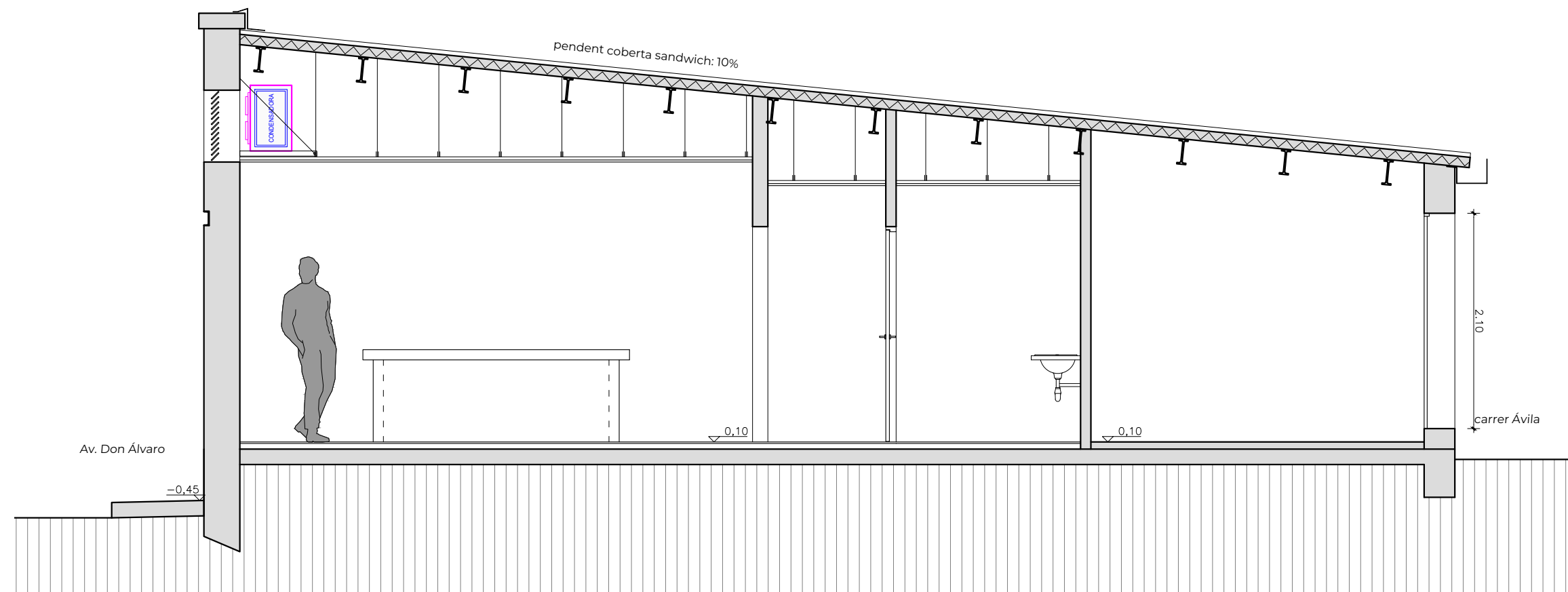
SECCIÓ INTERIOR LOCAL
