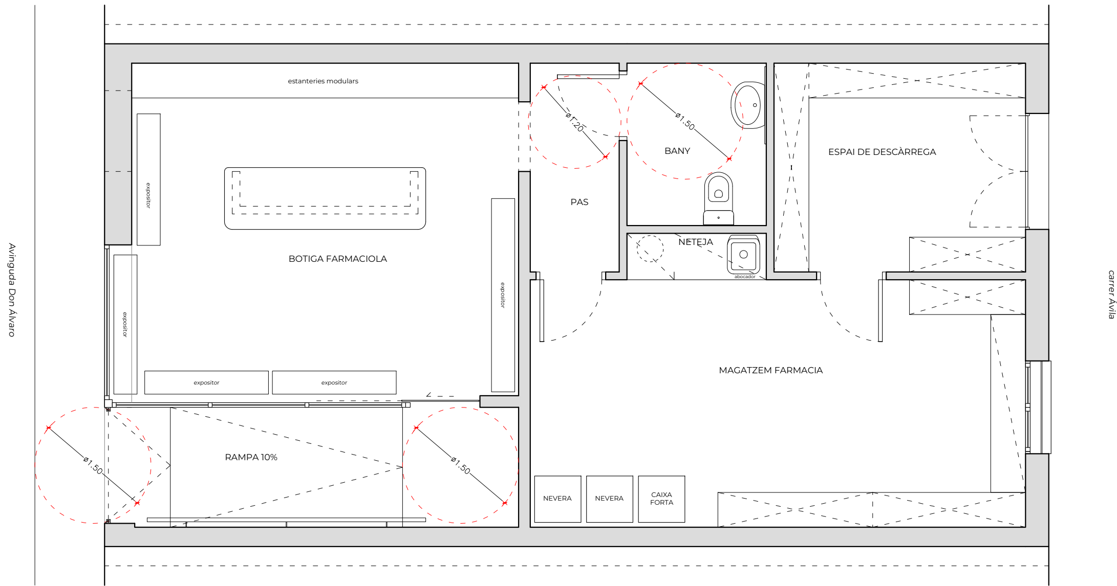
PLANTA DISTRIBUCIÓ I MOBILIARI
