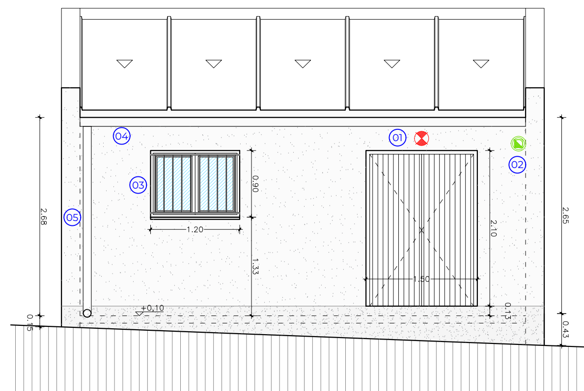
FAÇANA C/ ÀVILA
