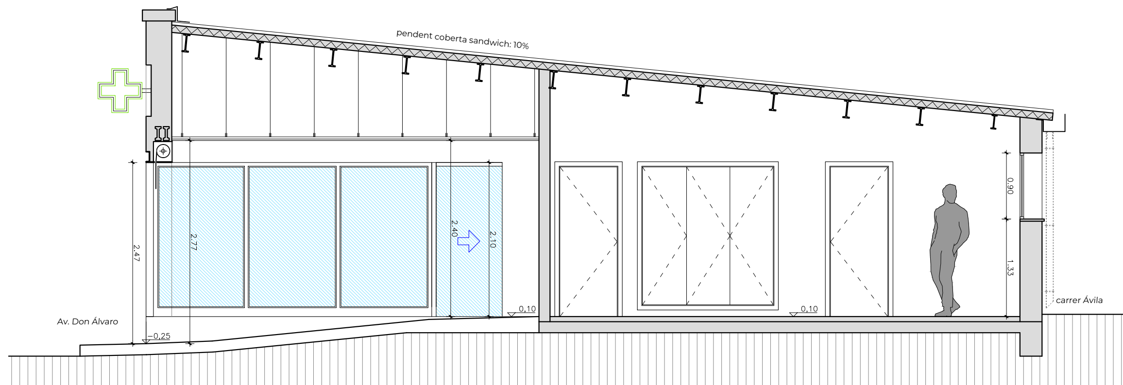
SECCIÓ PER LA PORTA D'ACCÉS
