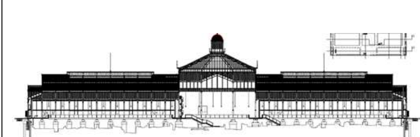
Secció longitudinal
