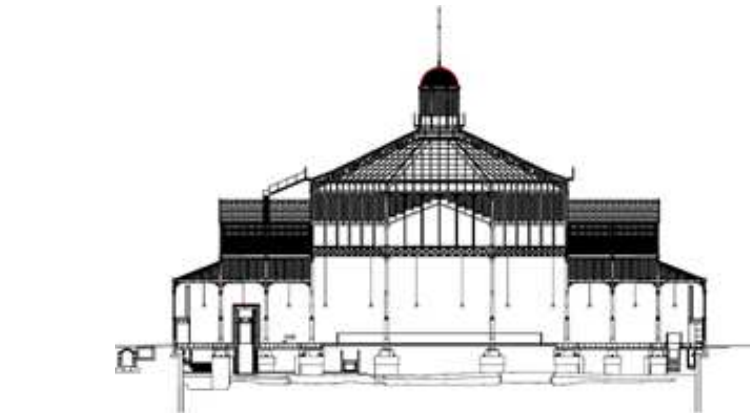
Secció transversal
