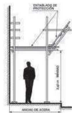
SECCIÓN TRANSVERSAL
