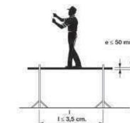
LONGITUD MAX. 3,5 m ESPESOR MIN. 50mm.
