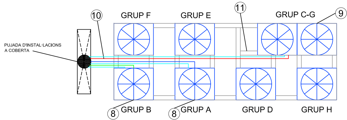
PLANTA COBERTA EDIFICI ECONOMIA I EMPRESA 696. UNITATS EXTERIORS ESTAT PROPOSAT
