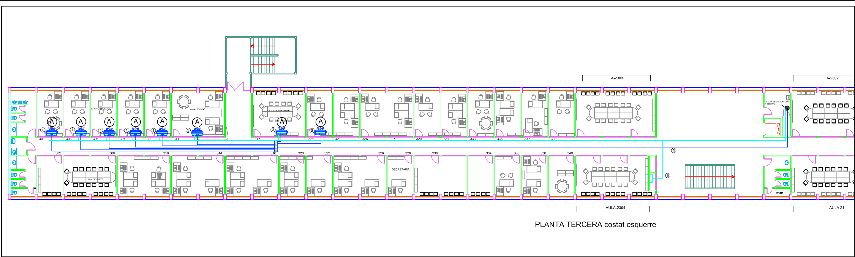
PLANTA 3ª EDIFICI ECONOMIA I EMPRESA 696. COSTAT ESQUERRRE. PROPOSTA GRUP A
