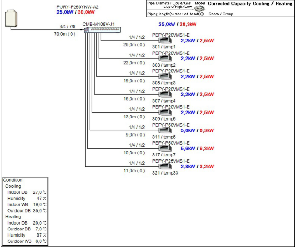
ESQUEMA DE LES LÍNIES FRIGORÍFIQUES GRUP A
