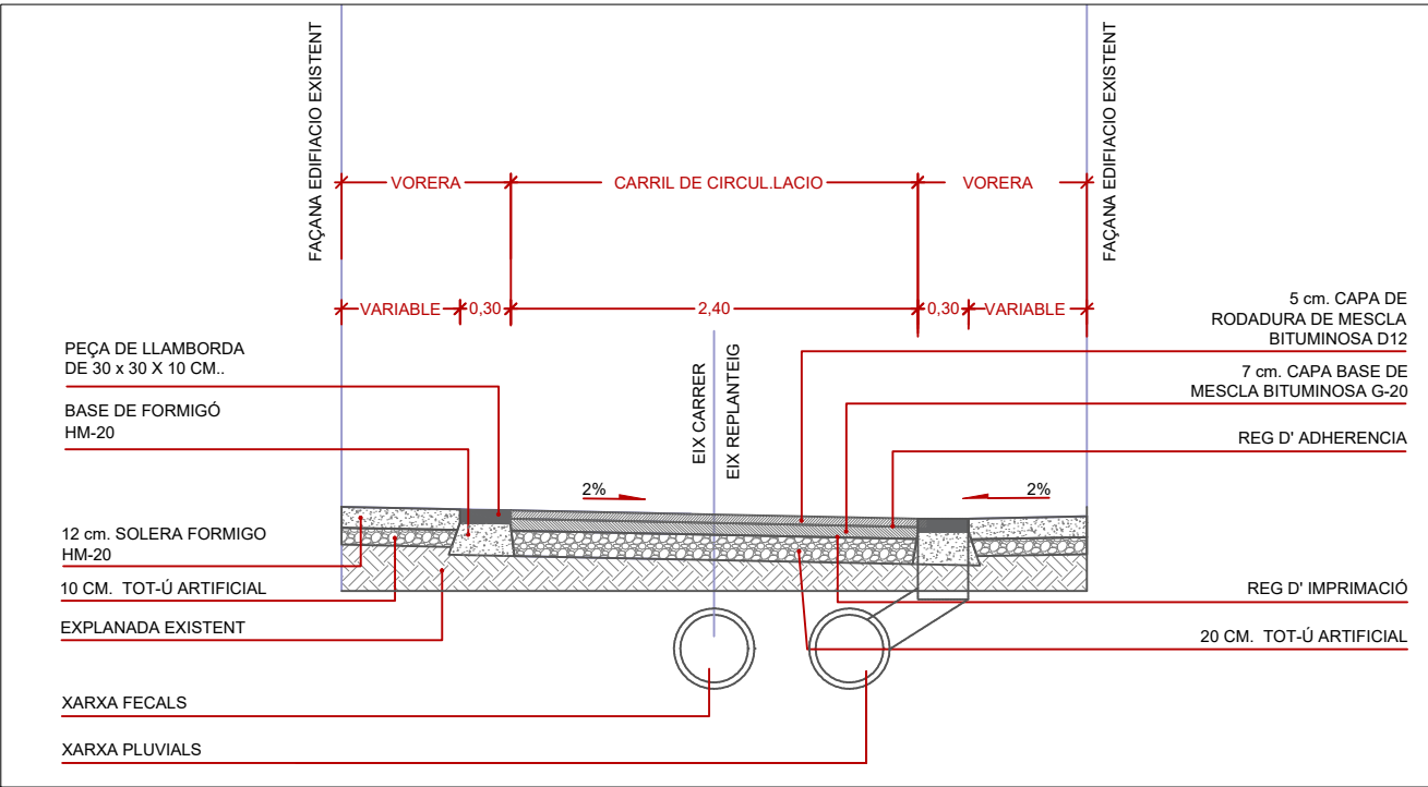
SECCI·O TIPUS escala 1/200
