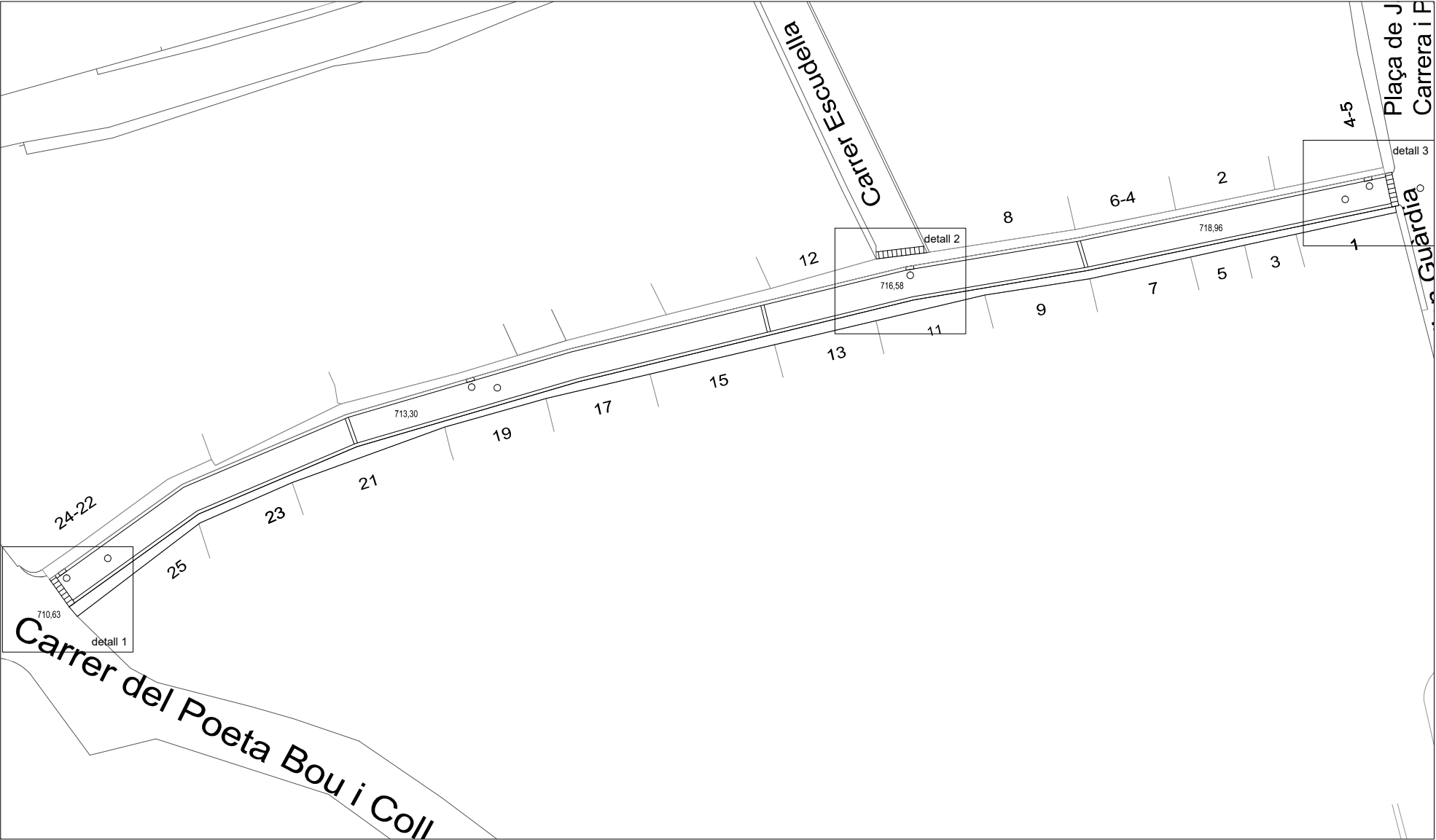
Proposta plataforma única escala 1/200
