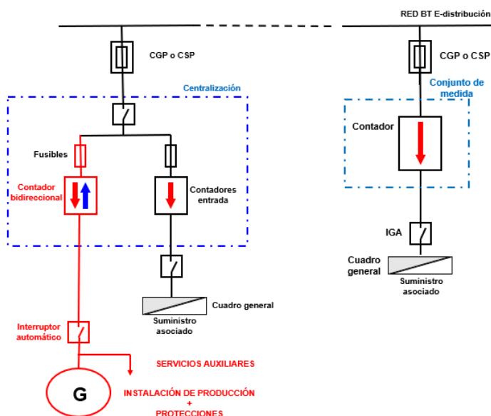
Esquema 15 de la Guía NRZ105 Endesa Distribución,SLU
