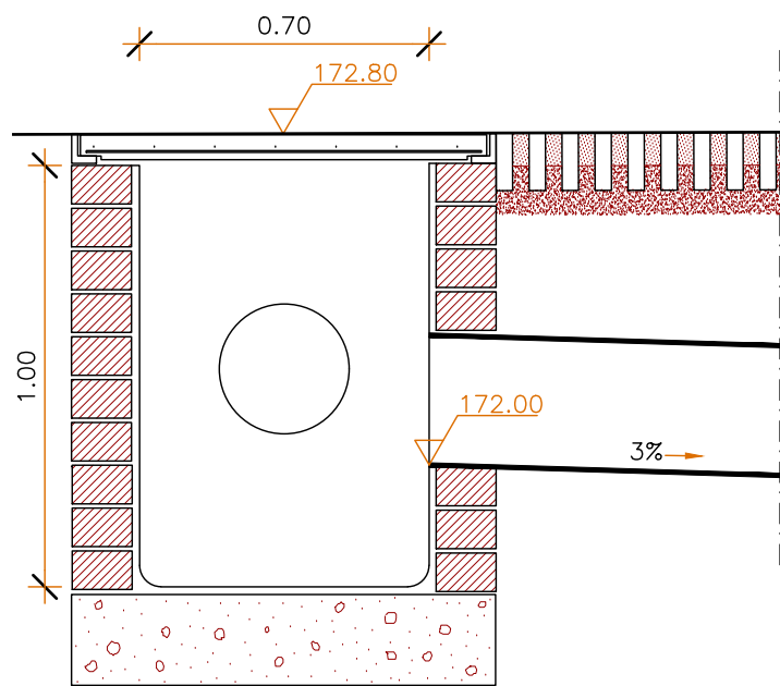
F Arqueta registrable 70x70x100cm
