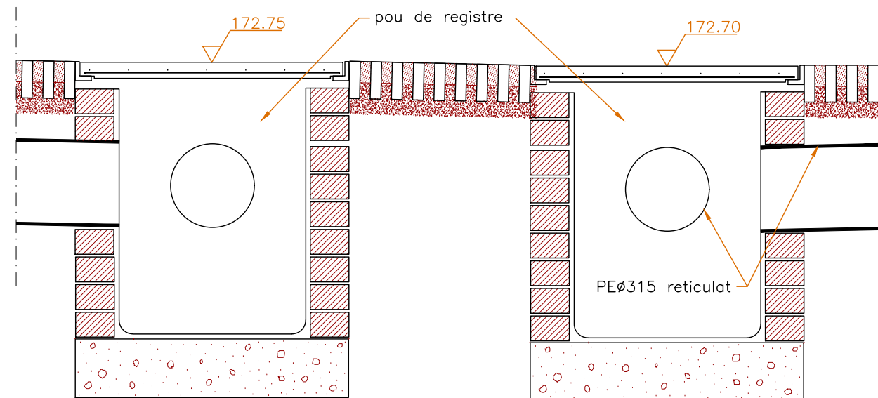
D Arqueta registrable de plujanes
