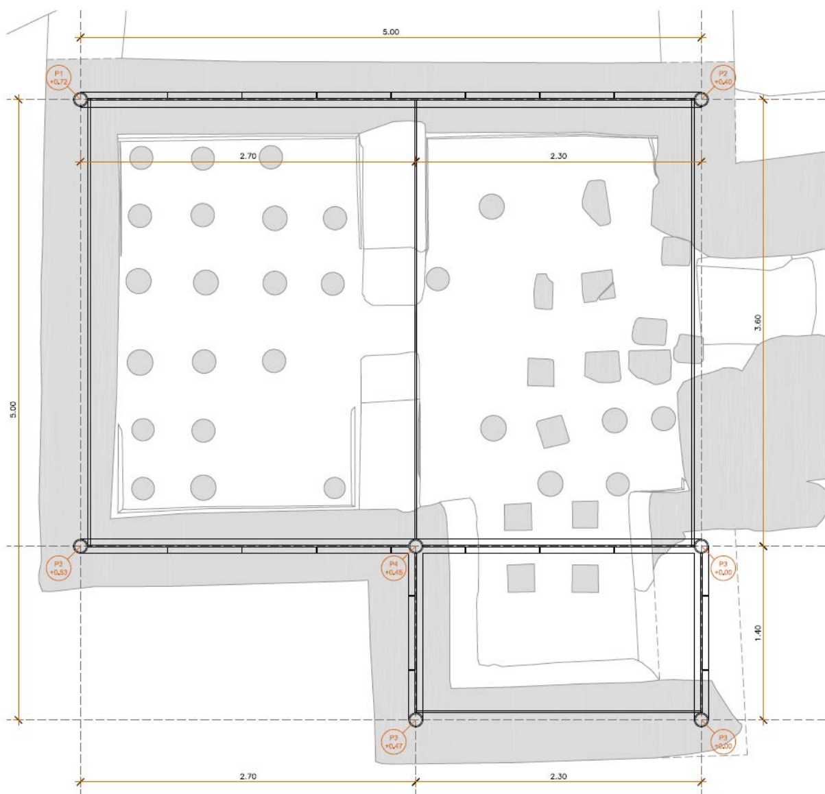
Planta d'implantació de l'estructura, orientació est-oest
