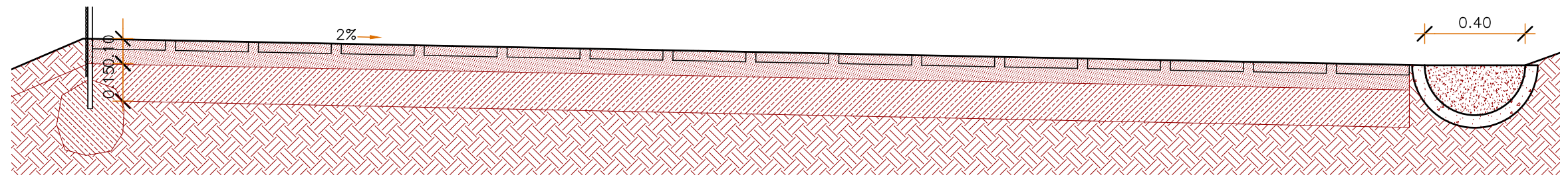
Detall constructiu pas i rigola
