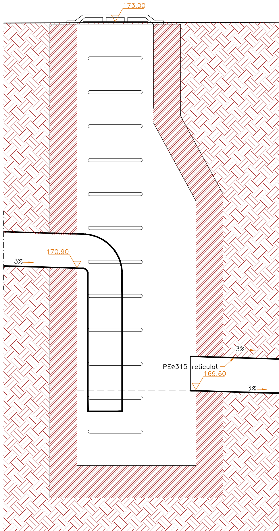
G Pou de descàrrega
