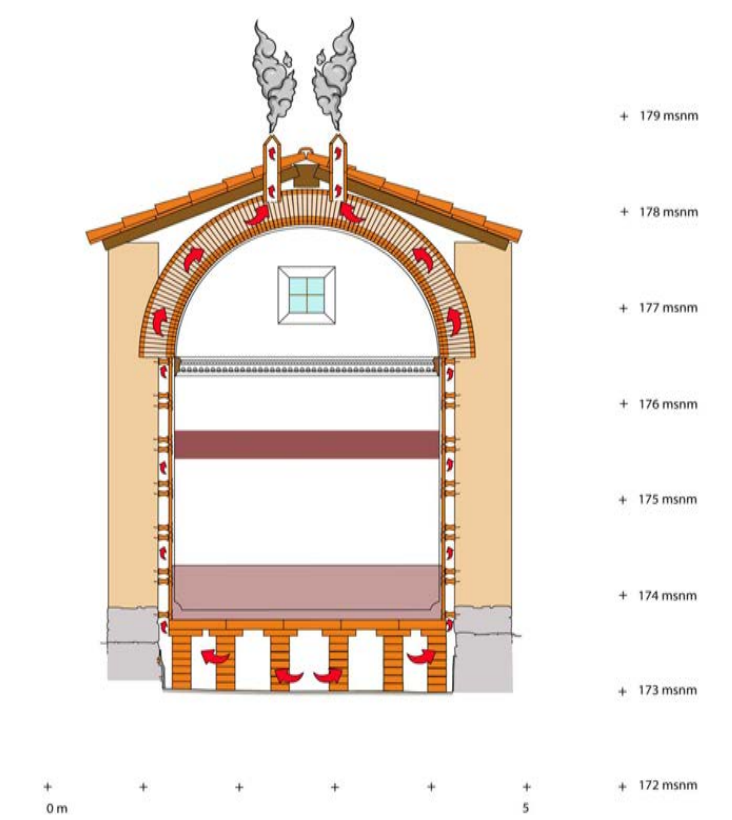
Esquema funcionament i cotes
