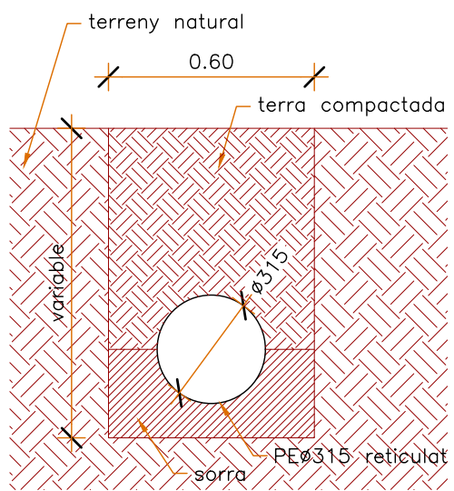
Detall rasa sanejament
