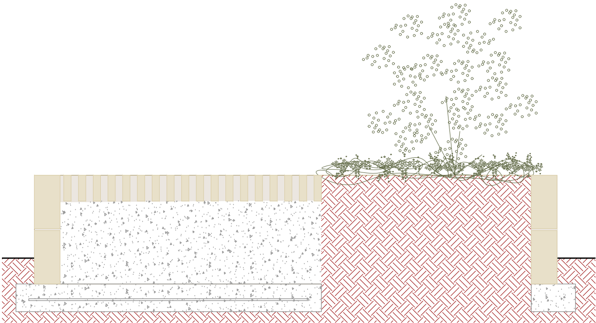
Secció B
