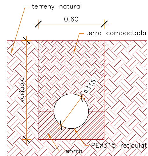
Detall rasa sanejament
