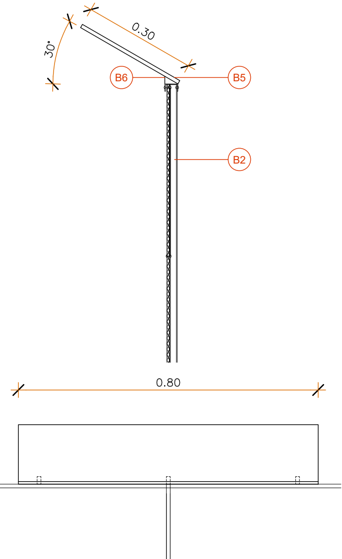
Detall rètols e 1:10
