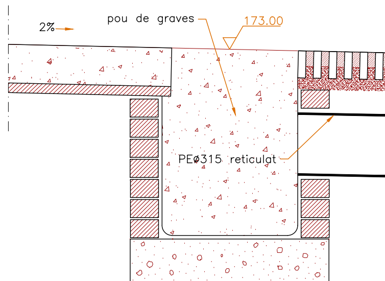
C Pou de graves de Plujanes
