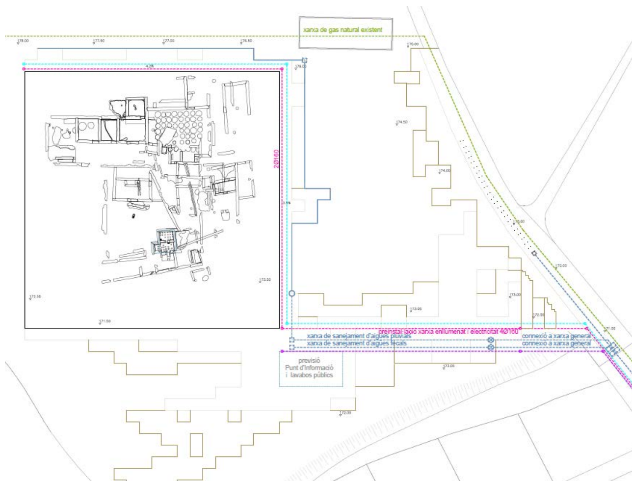
Distribució general dels serveis previstos i previsió d'instal·lacions, en superfície i soterrades. Veure documentació gràfica
