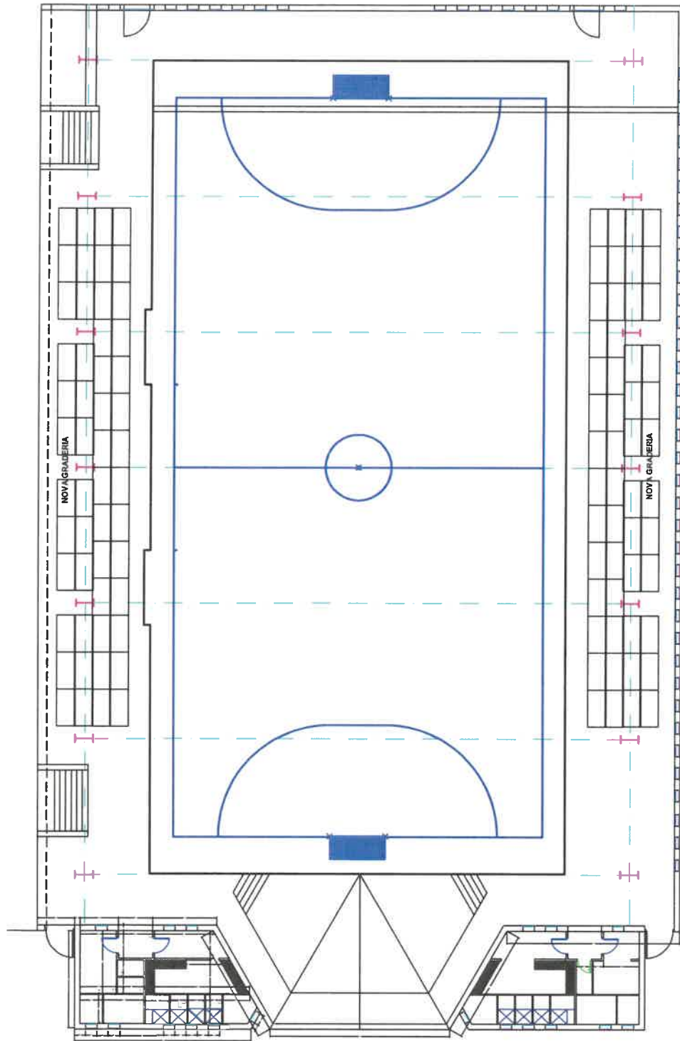
PLANTA DE SITUACIÓ E = 1:100
