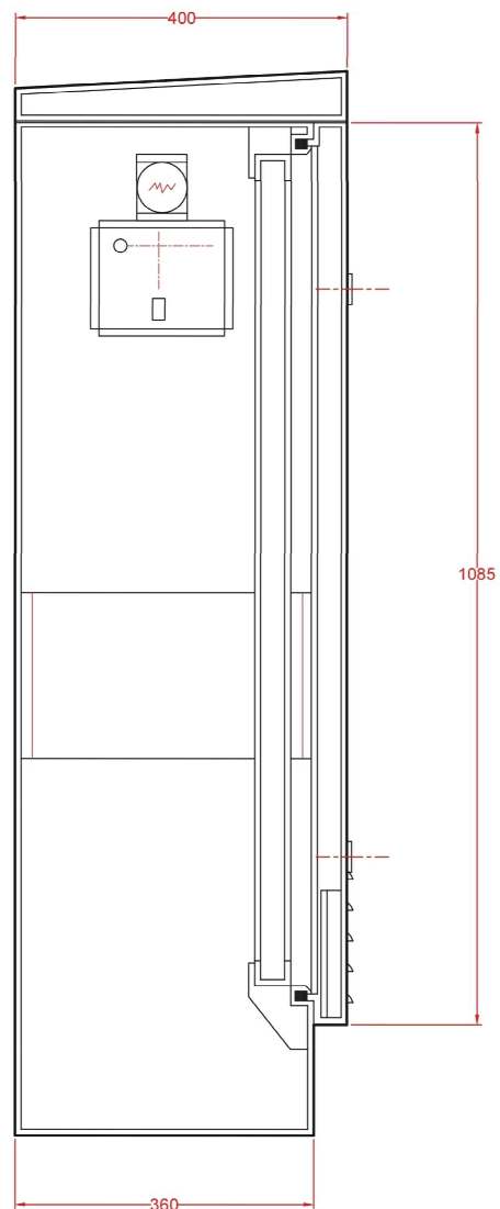
SECCIÓ A-A
