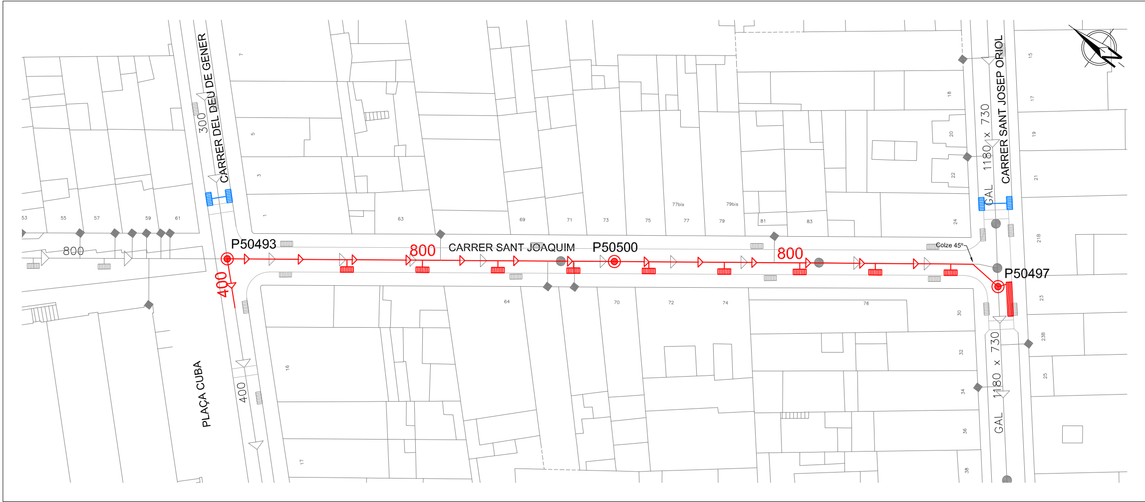
PLANTA (E:1/500)
