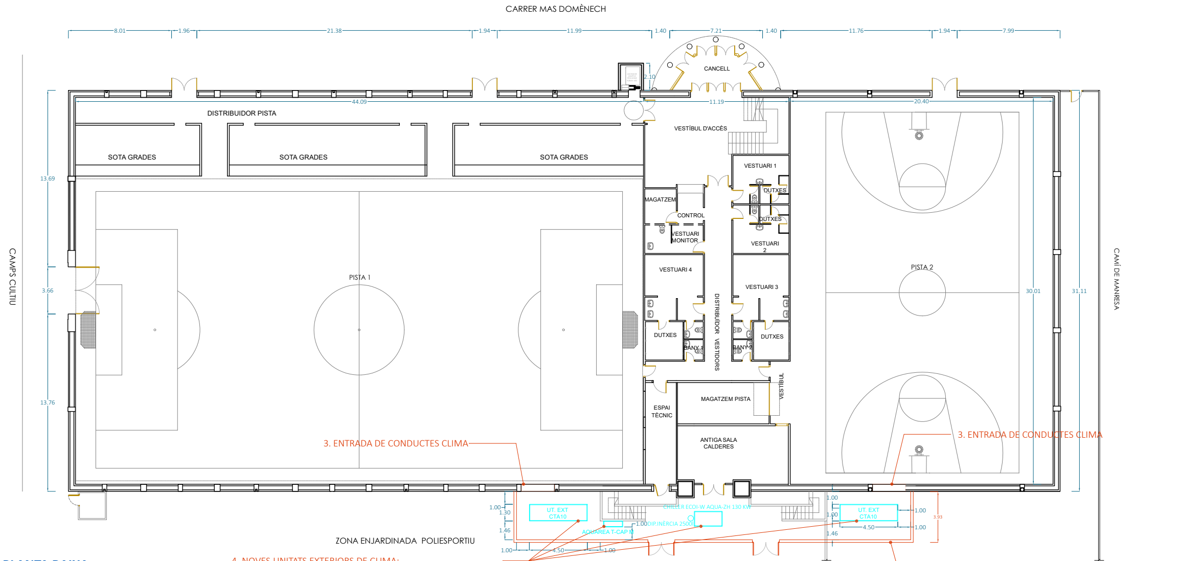
PLANTA BAIXA
