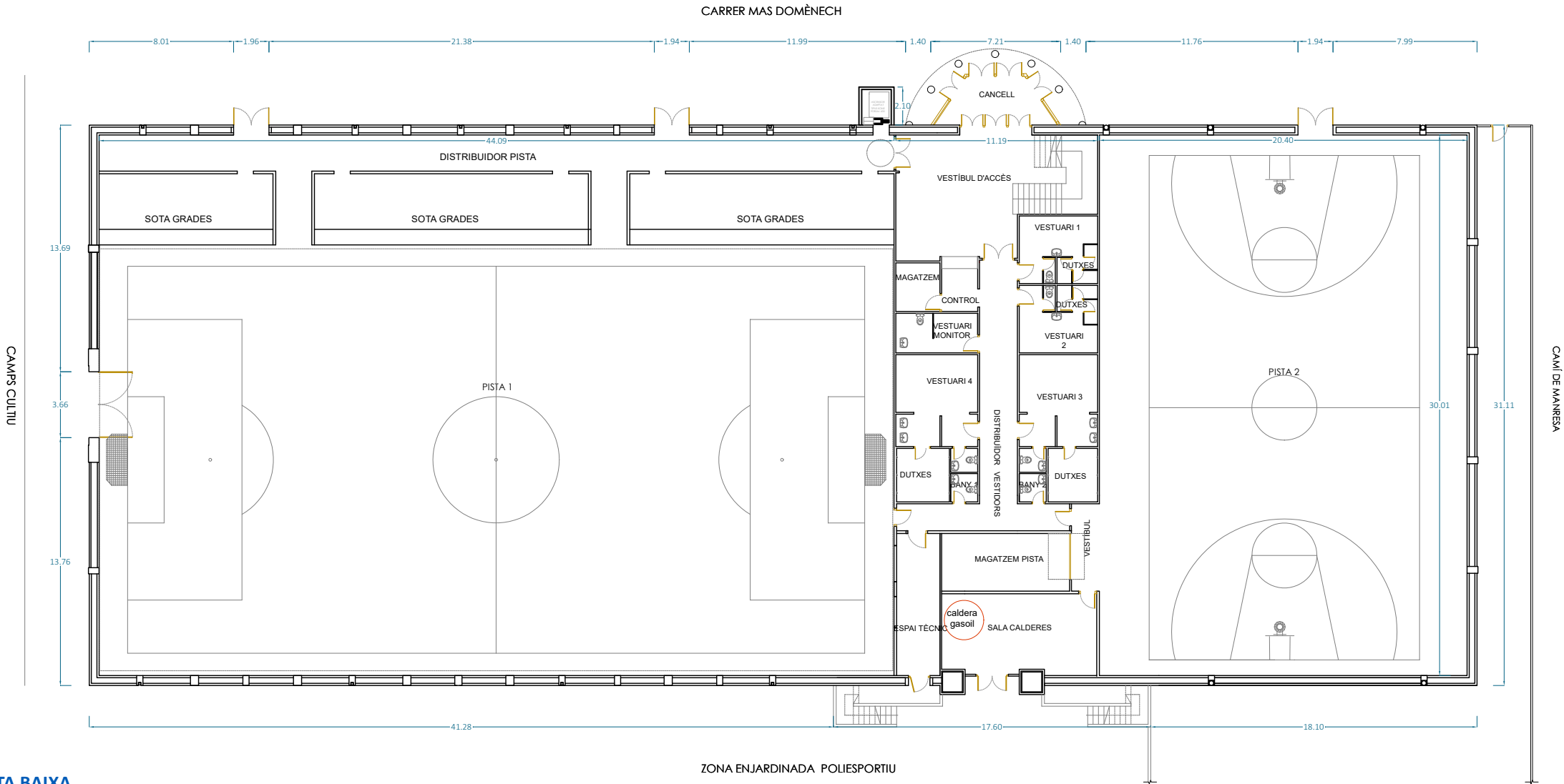
PLANTA BAIXA
