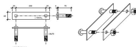
DETALL PLETINA FIXACIÓ PASSAREL·LES
