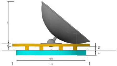
Àrea de seguretat de cada semiesfera, diàmetre 3m.
