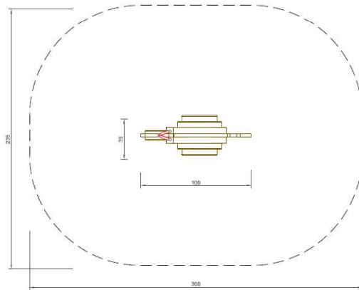
PLANTA Y ÁREA DE SEGURIDAD E: 1/20
