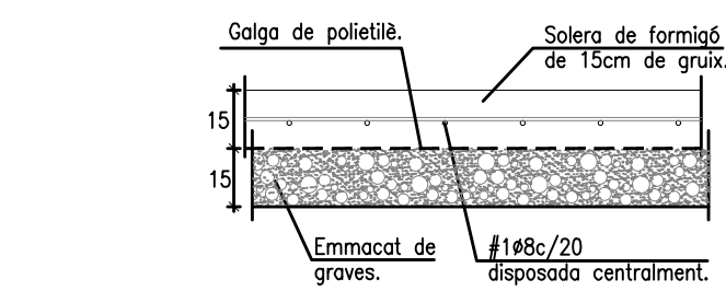
DETALL SOLERA E 1/20
