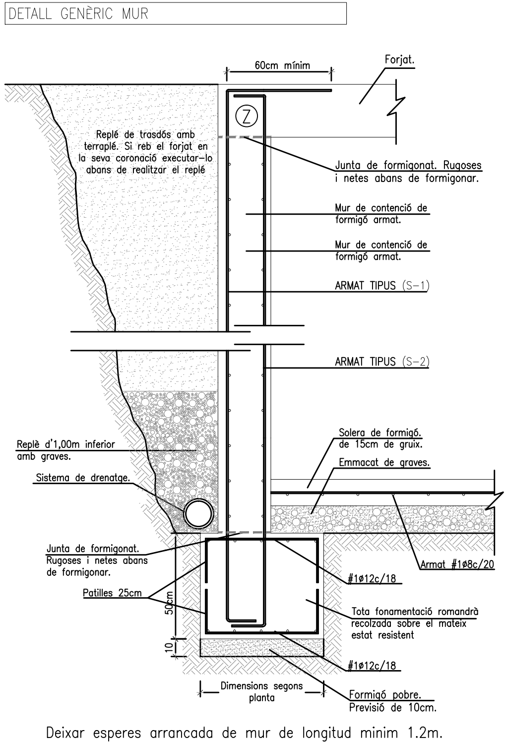
DETALL MUR DE CONTENCIÓ 35CM. E 1:20 - 1:50
