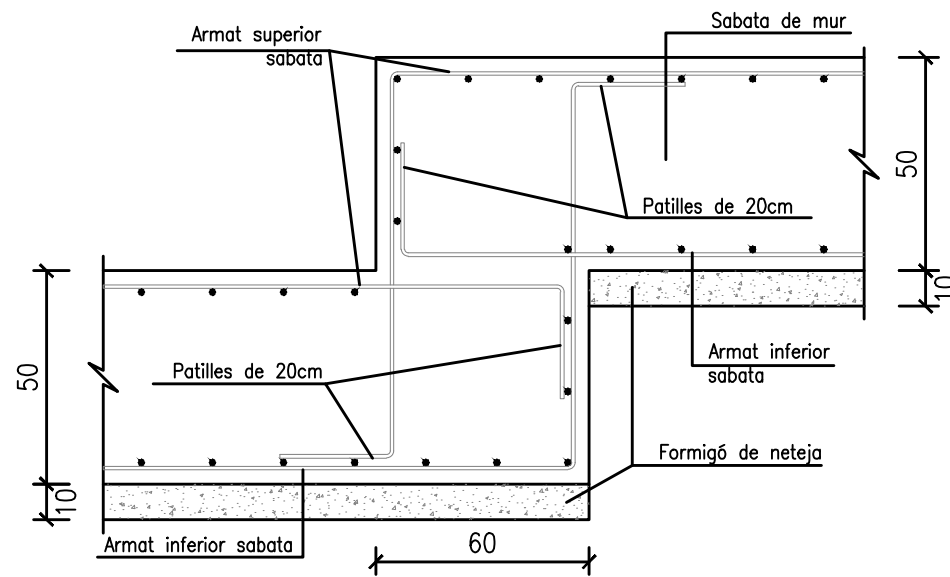
DETALL CANVI DE NIVELL EN SABATA DE MUR E 1:20
