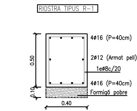
DETALL RIOSTRES E.1/20
