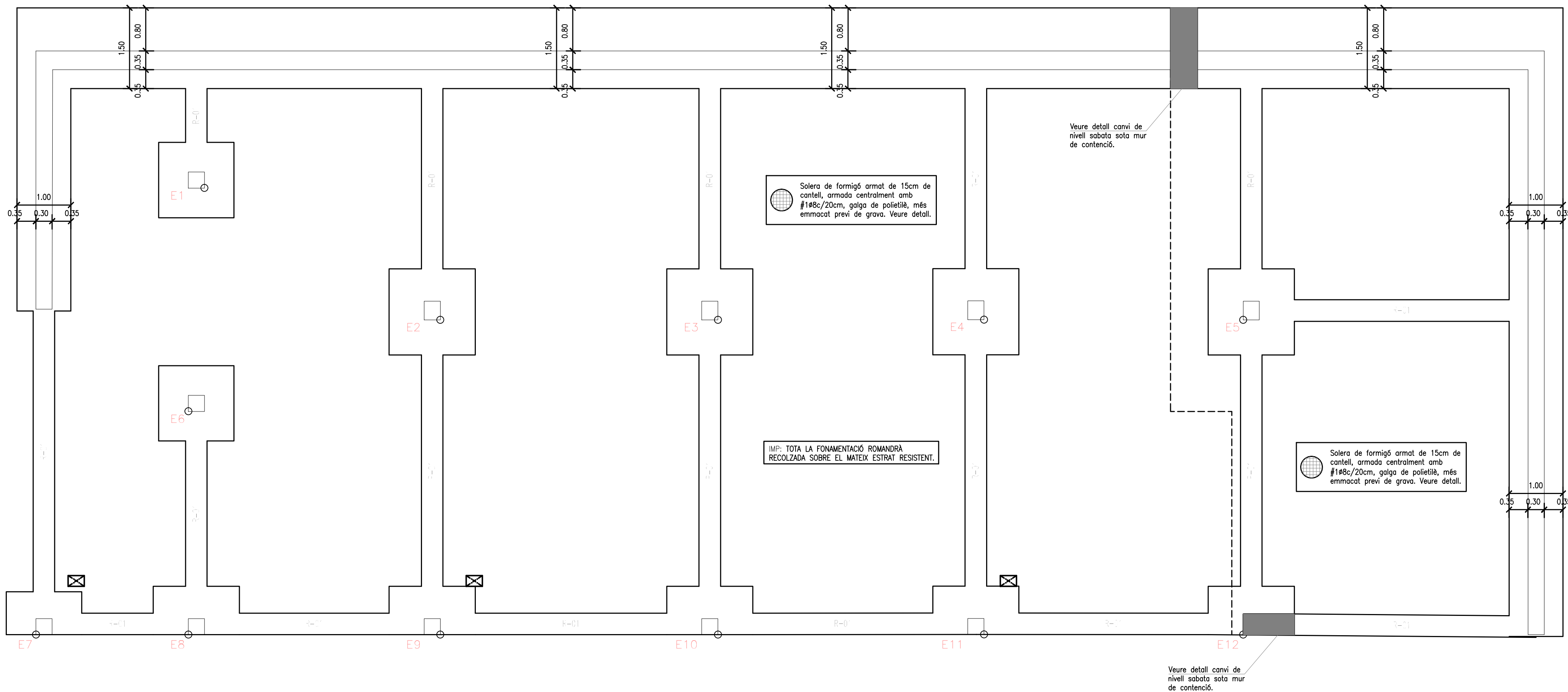
FONAMENTACIÓ E 1/50
