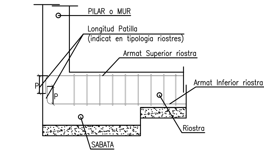
DETALL TROBAMENT SABATA AMB RIOSTRA DE FONAMENTACIÓ E 1/20
