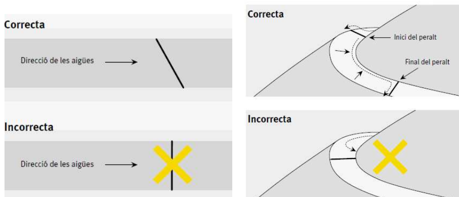
Figura 8: Posició dels trencaigües (FONT: DIBA. Fitxa 2. Arranjament de pistes forestals)
