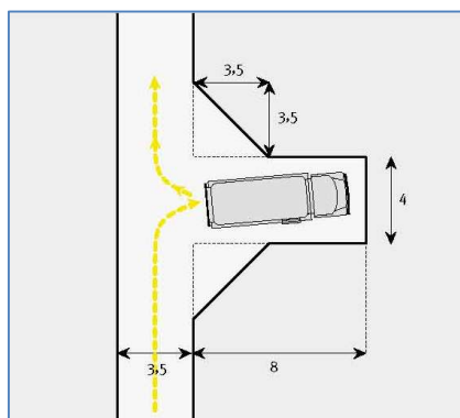
Figura 20: : Esquema d'un girador en forma de T (Font: Fitxa tècnica 02 de la Diba)
