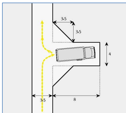
Figura 10: : Esquema d'un girador en forma de T (Font: Fitxa tècnica 02 de la Diba)
