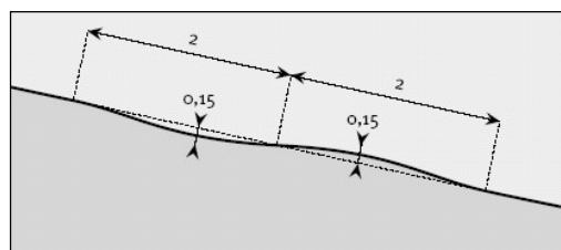
Figura 9: Tall paral·lel a la direcció del camí del trencaigües FONT: DIBA. Fitxa 2. Arranjament de pistes forestals
