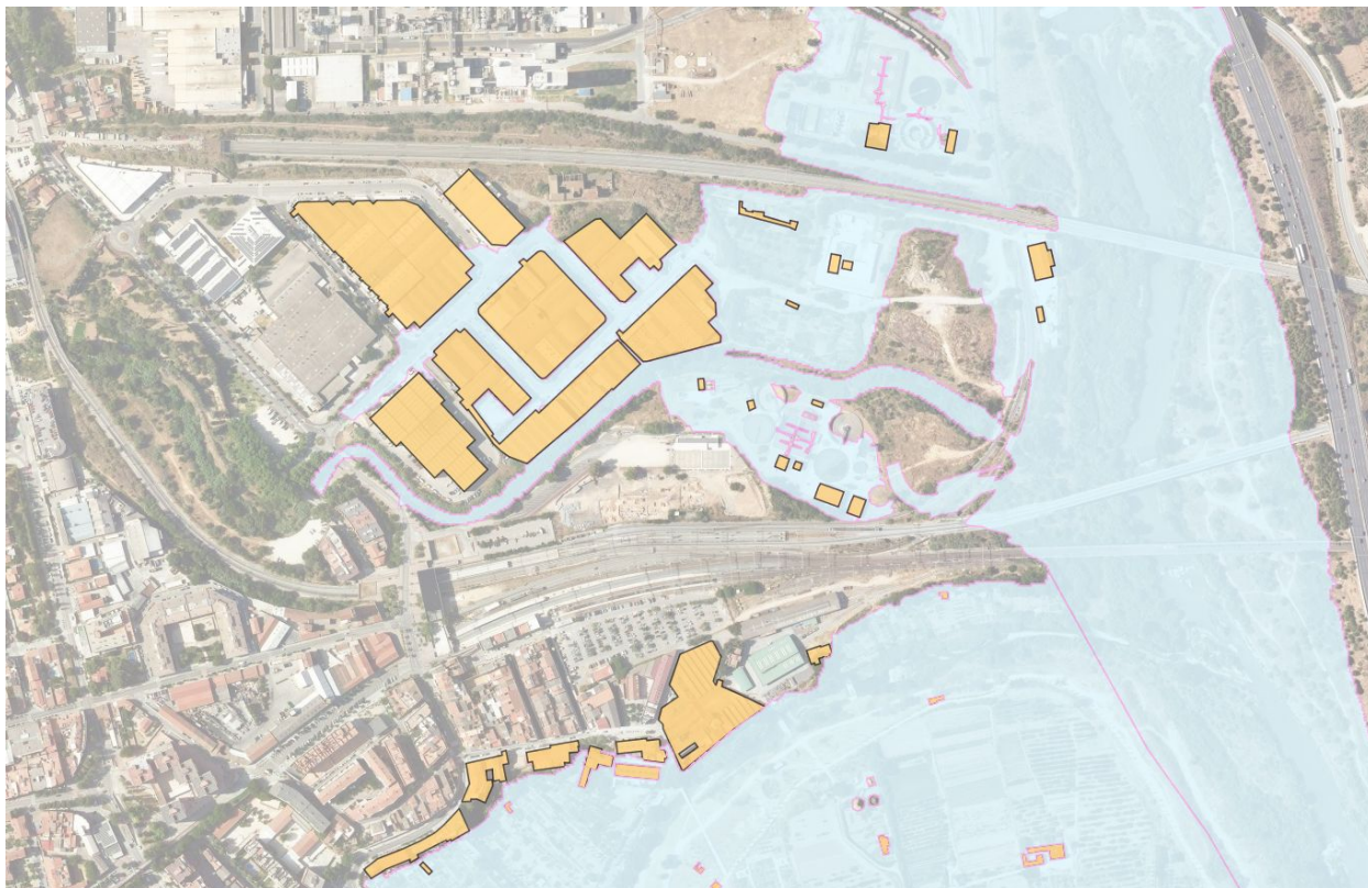
Plànol de l'ACA d'inundabilitat 100 anys de període de retorn en l'àmbit del Polígon La Torre
