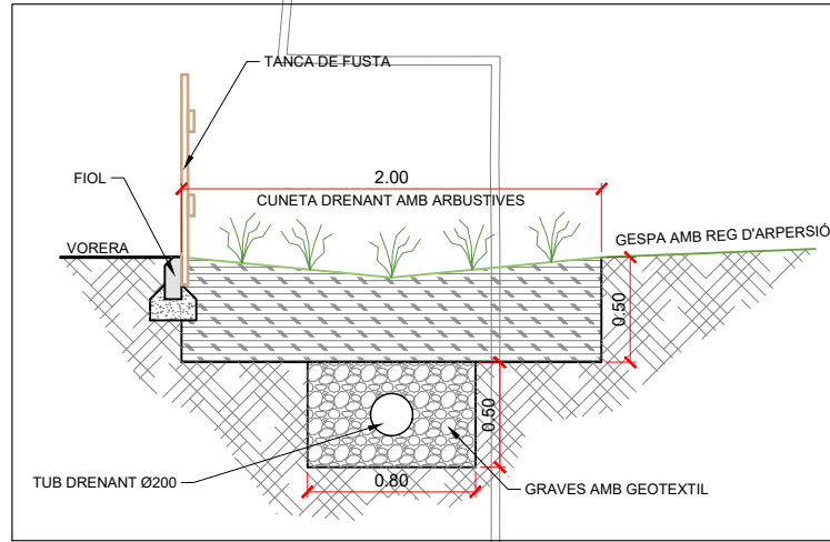
DETALL CUNETA DRENANT
