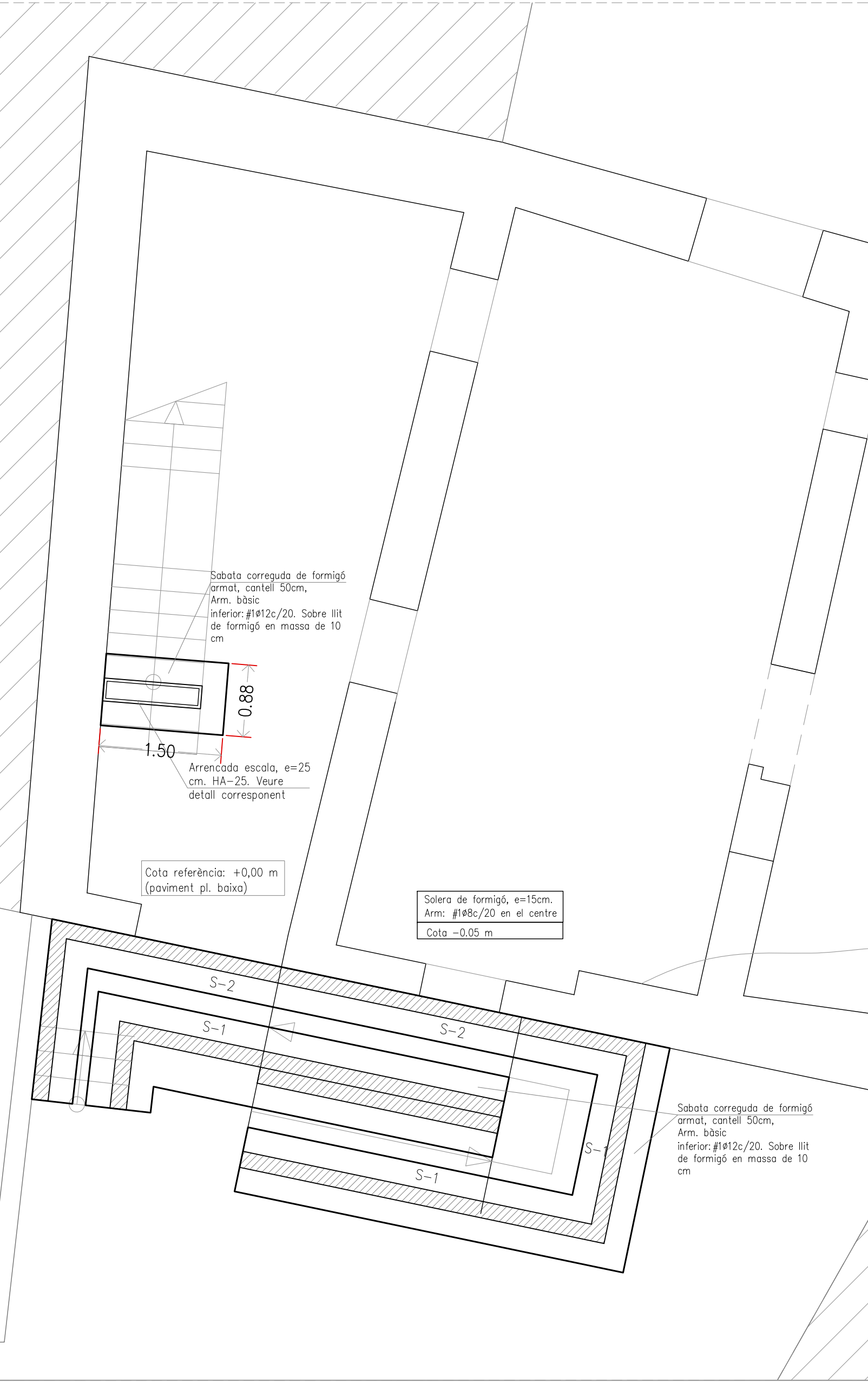
PLANTA FONAMENTACIÓ
