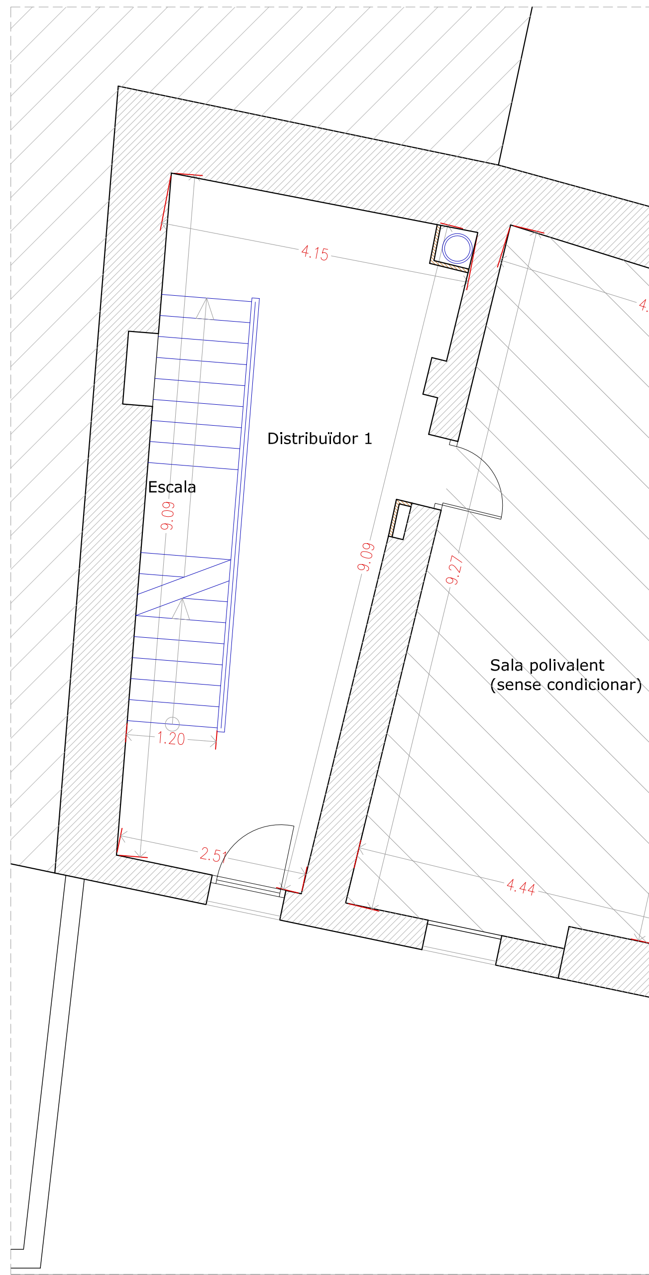
PLANTA PRIMERA
