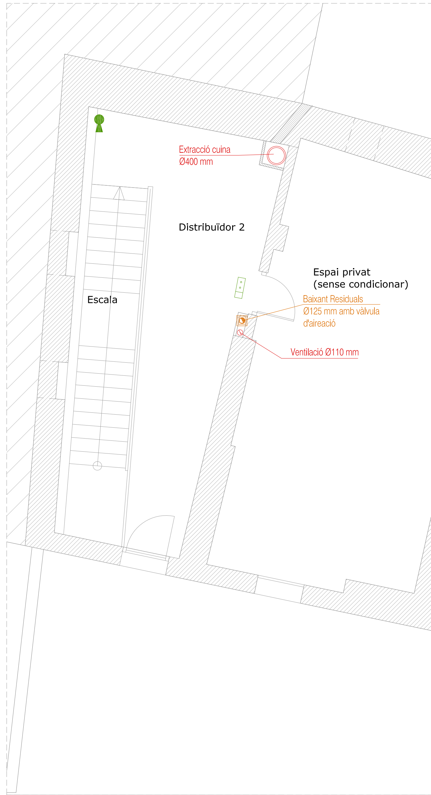
PLANTA SEGONA
