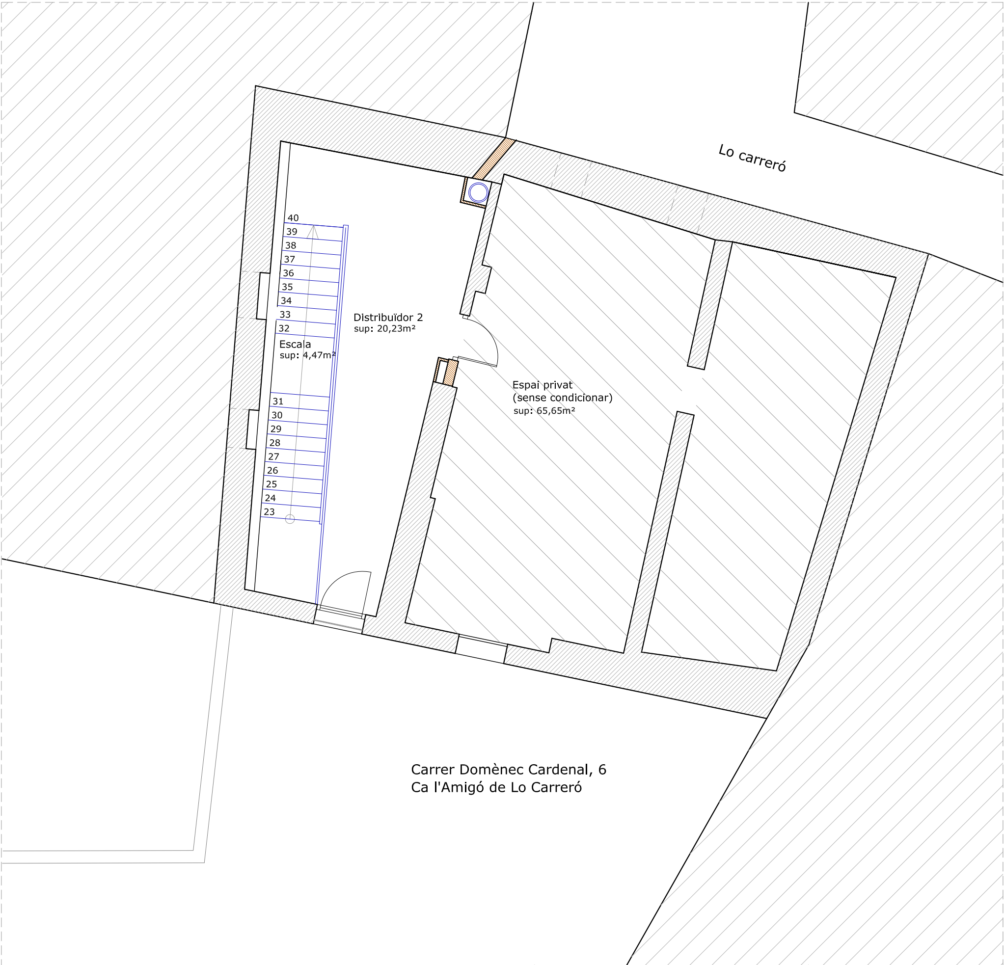
PLANTA SEGONA
