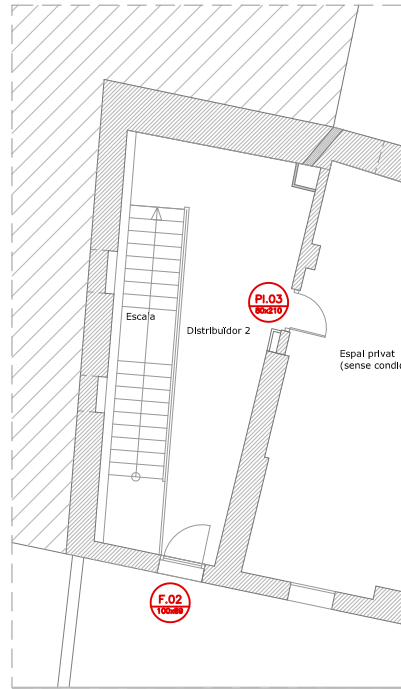
PLANTA SEGONA
