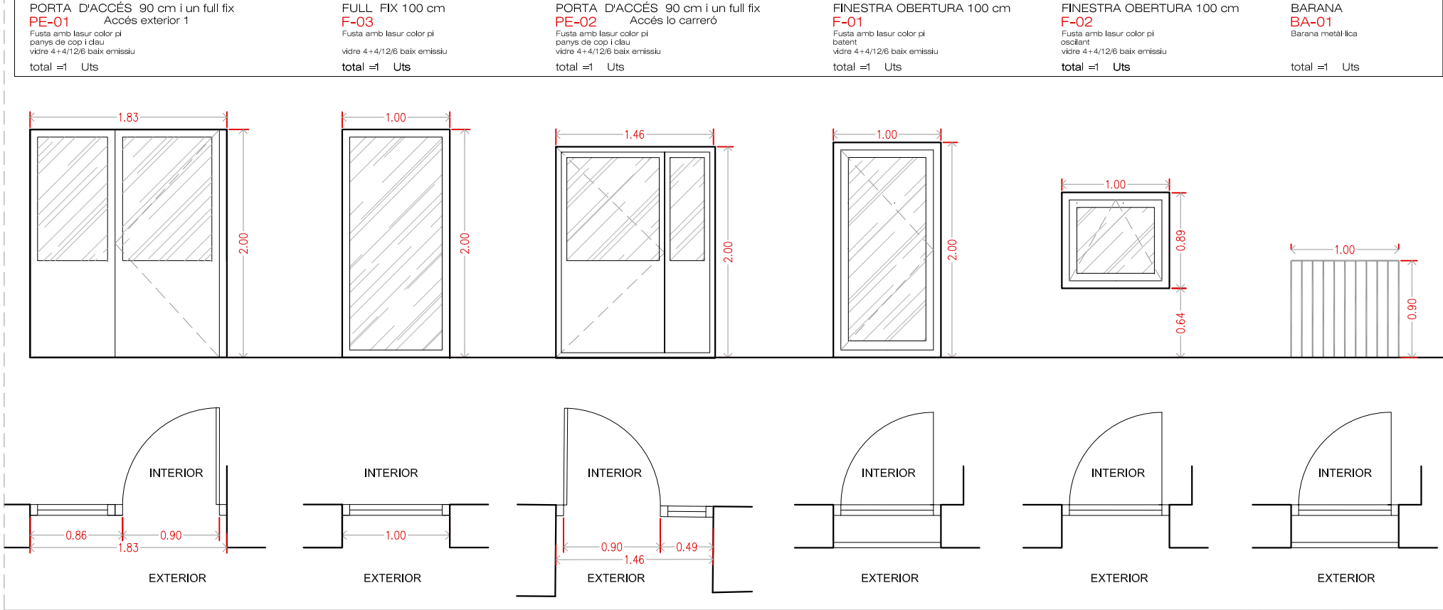
FUSTERIA EXTERIOR
