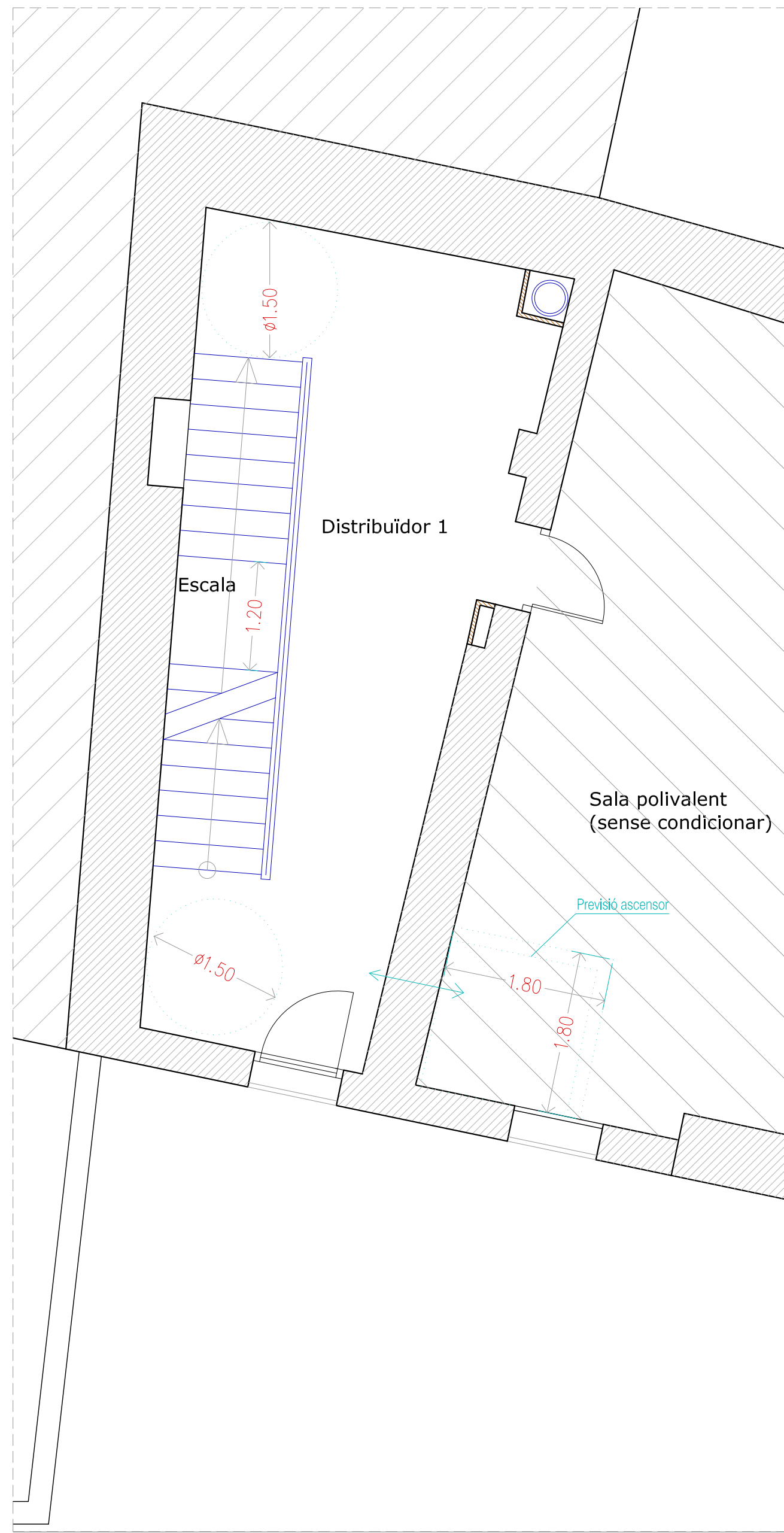
PLANTA PRIMERA
