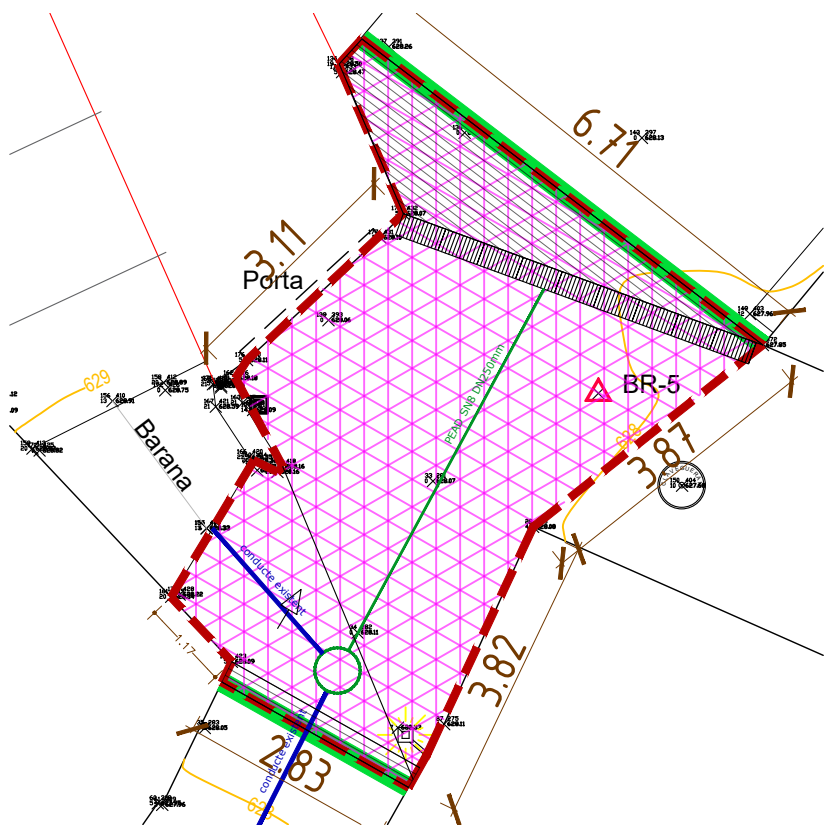
PLANTA ENDERROCS I CLAVEGUERAM 1/100
