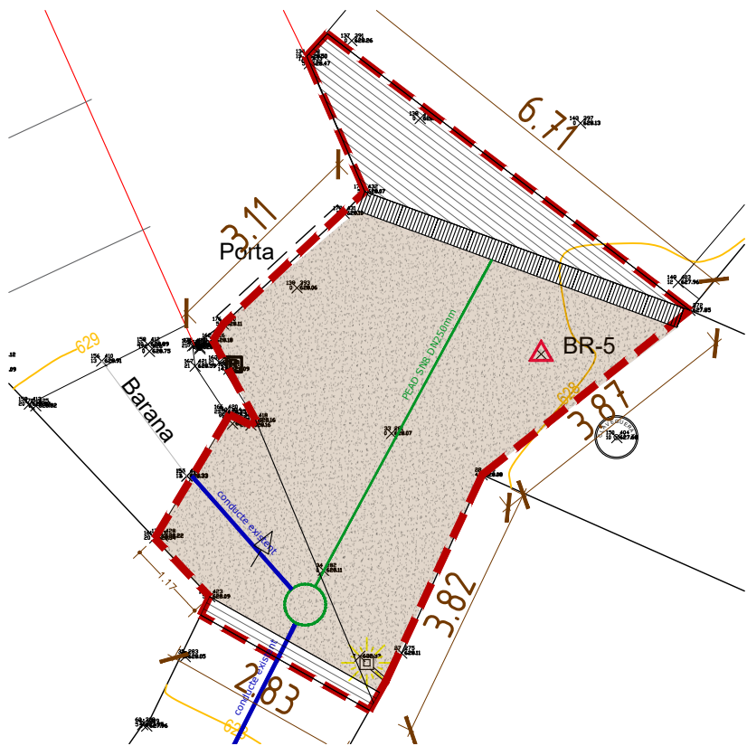
PLANTA PROPOSTA 1/100
