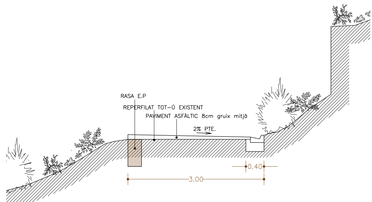
SECCIÓ TRANSVERSAL PROPOSTA 1/50
