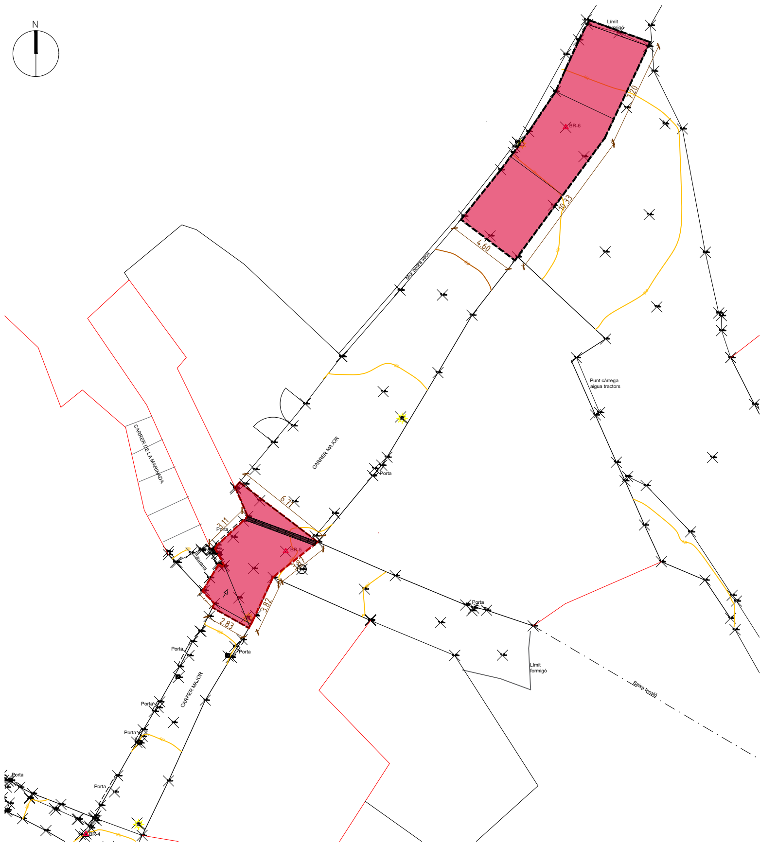
ZONES DE TREBALL CARRER MAJOR FINS A VIAL DE CONNEXIÓ 1/250
