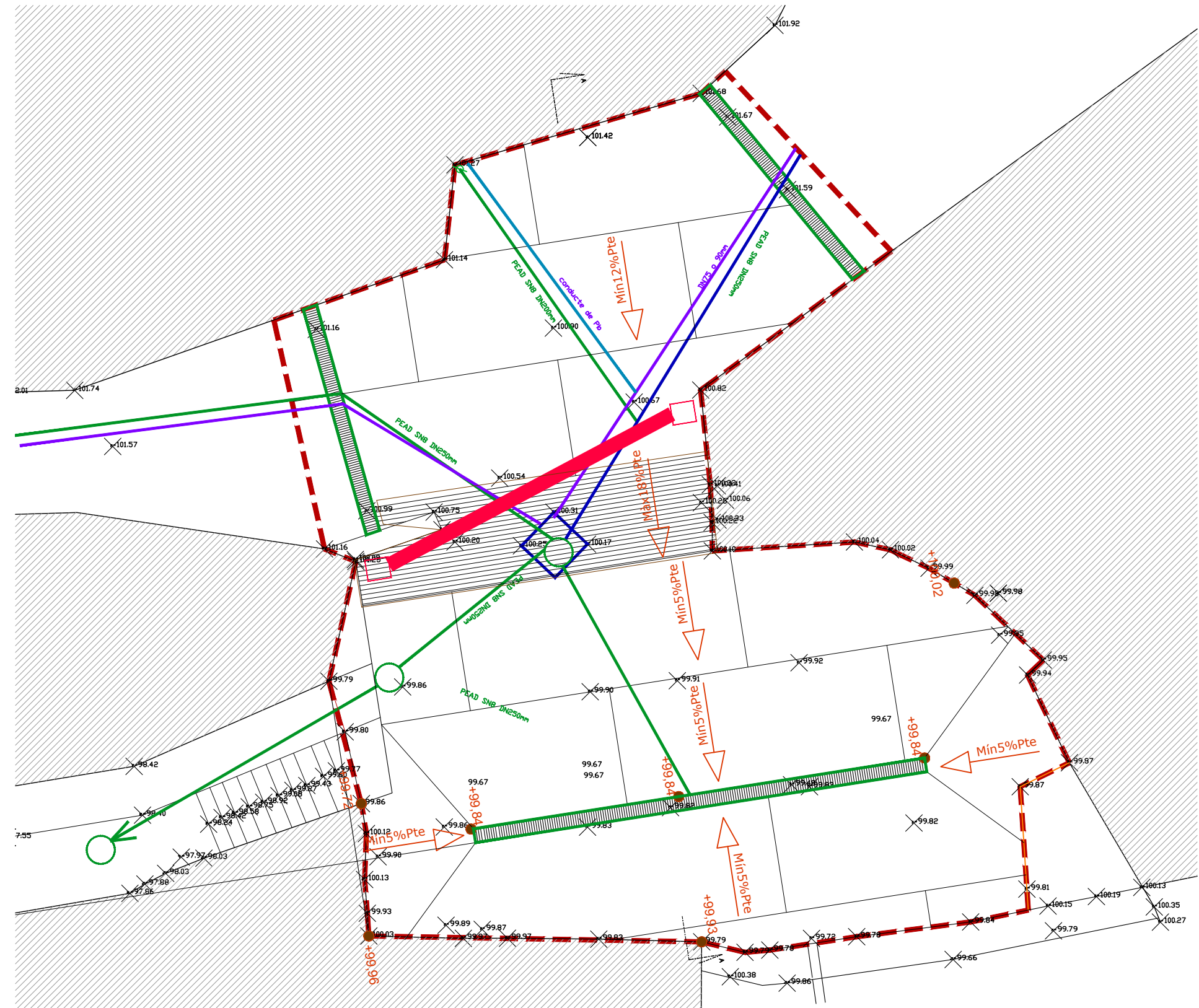
PLANTA CLAVEGUERAM PLAÇA MAJOR 1/100
