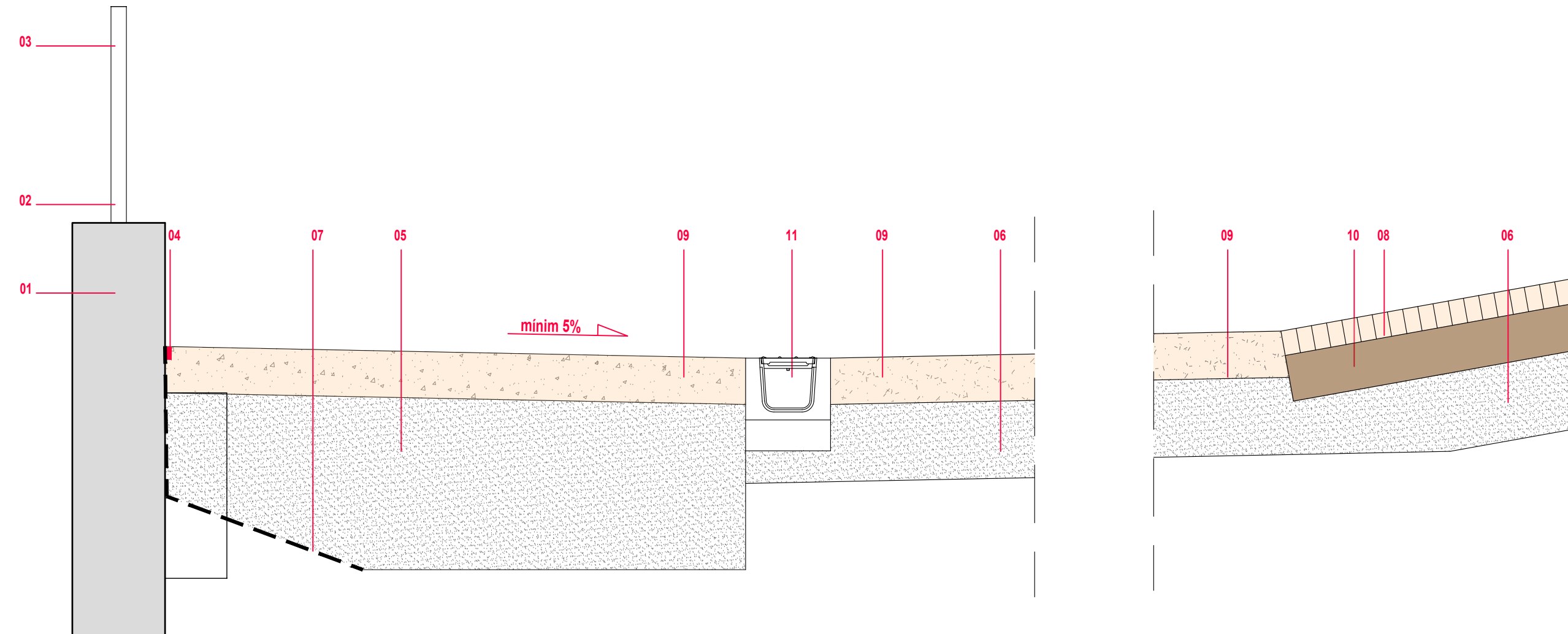
DETALL PLAÇA MAJOR 1/15
