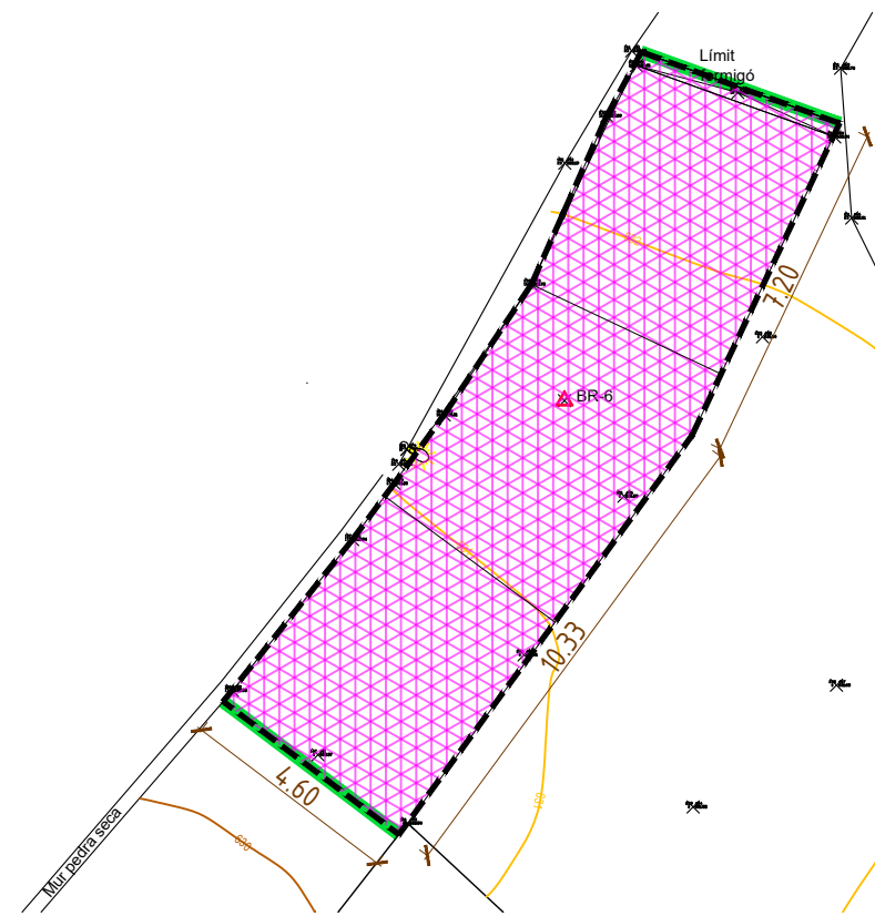
PLANTA ENDERROCS I CLAVEGUERAM 1/100
