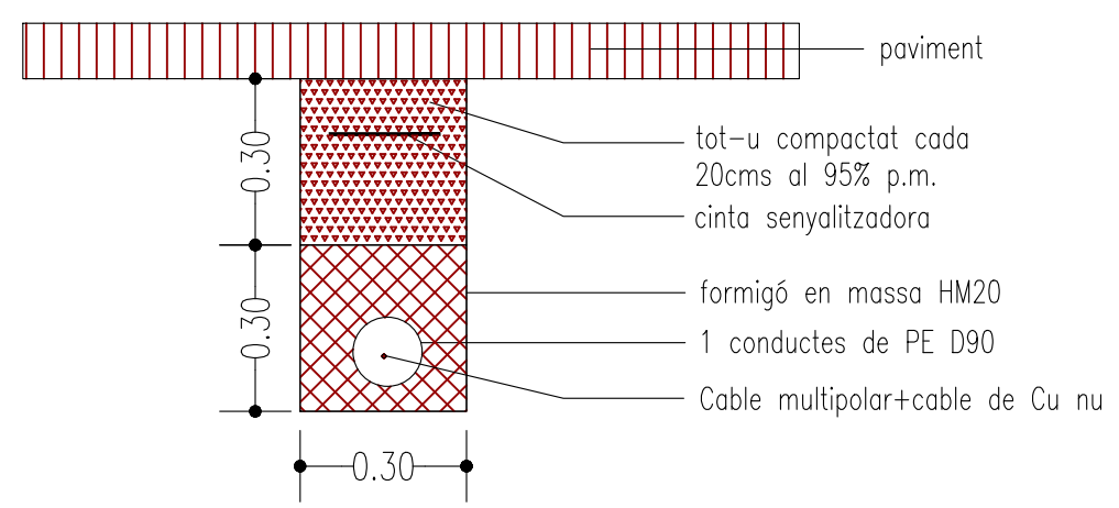
SECCIÓ TRANSVERSAL PROPOSTA 1/50
