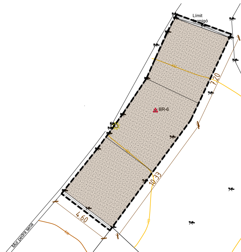
PLANTA PROPOSTA 1/100
