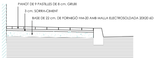
DETALL REPOSICIÓ VORERA ON CIRCULEN VEHICLES SECCIÓ TRANSVERSAL
