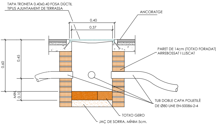
PERICO DE REGISTRE - E. 1 : 10
