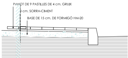
DETALL REPOSICIÓ VORERA SECCIÓ TRANSVERSAL
