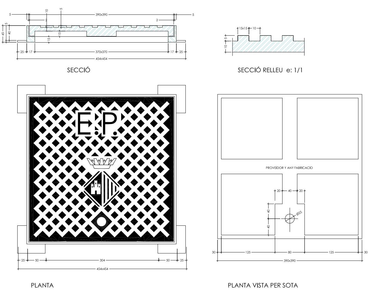
MARC I TAPA PERICÓ (B-125) ENLLUMENAT PÚBLIC - E. 1 : 3 - COTES EN mm. -FOSA DÚCTIL-
