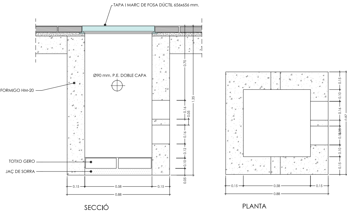
PERICÓ DE REGISTRE PAS DE SERVEIS - E. 1 : 10
