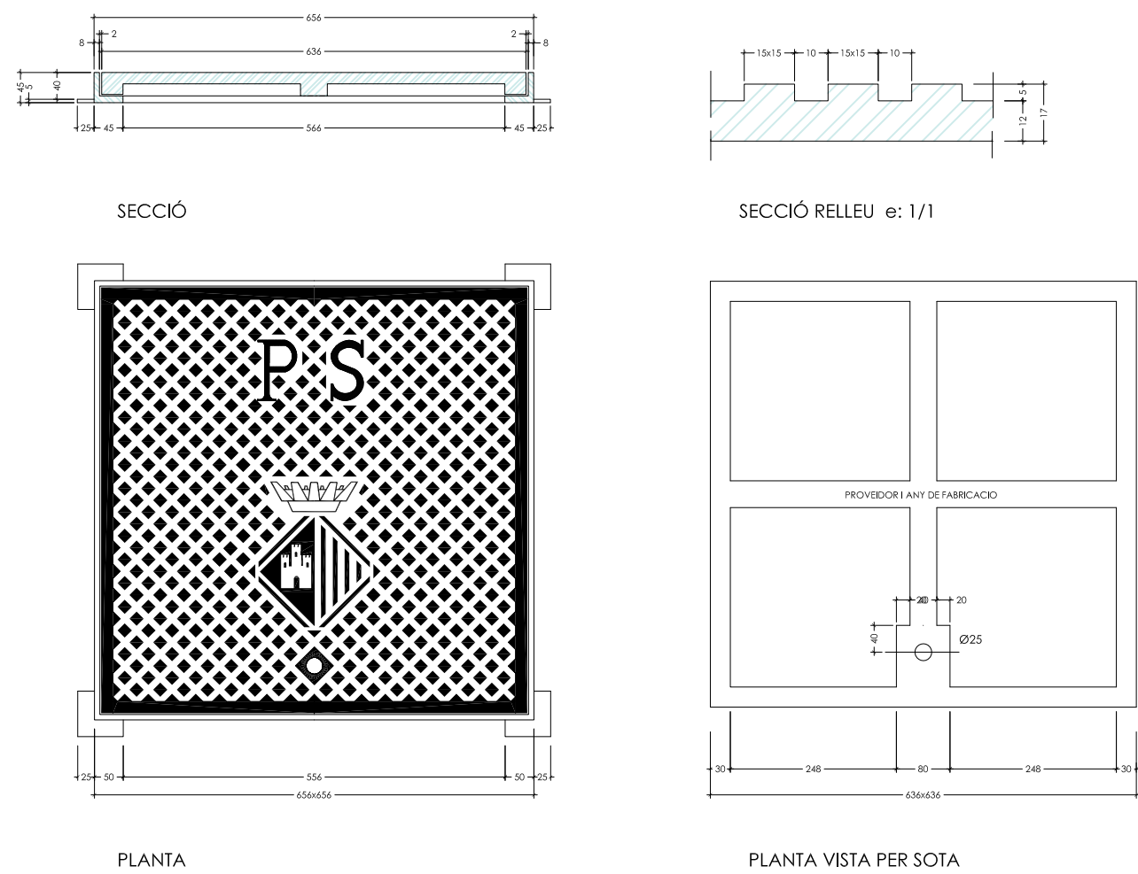
MARC I TAPA PERICÓ PAS DE SERVEIS (C-250) - E. 1 : 5 -COTES EN mm. -FOSA DÚCTIL-
