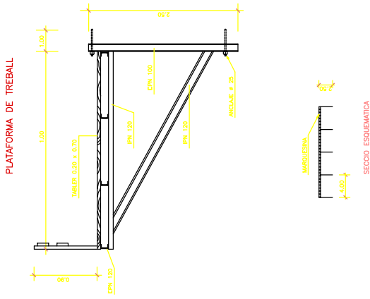
GUINDOLA DE SOLDADURA PER A ESTRUCTURES D' ACER
