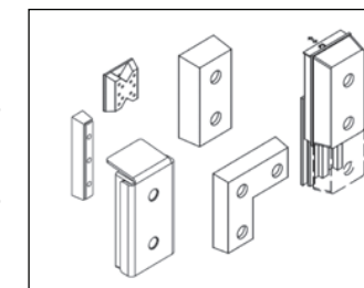
Figura 22. Tipos de topes de goma.
