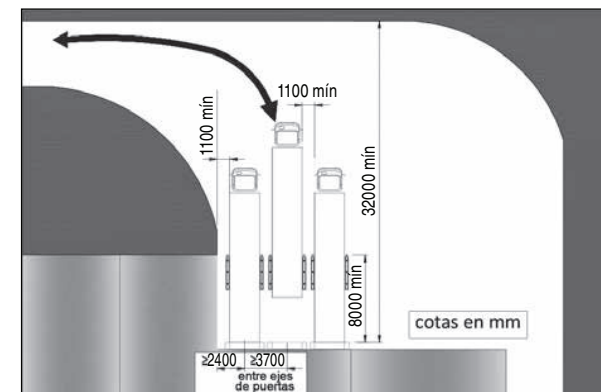
Figura 7. Distancias entre las estaciones de carga y descarga.
