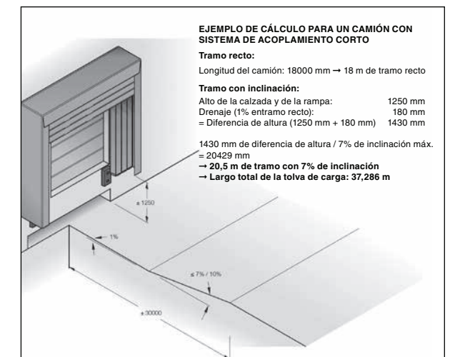
Figura 9. Ejemplo de cálculo de la longitud de una tolva de carga.
