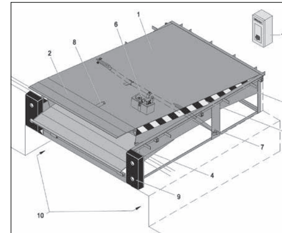
Figura 20. Rampa nivelable motorizada. Partes principales.
