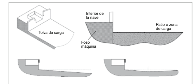
Figura 8. Tolva de carga. Vista general y tipos de secciones.
