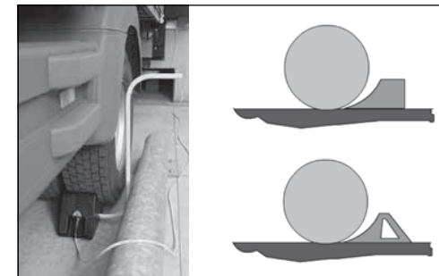
Figura 29. Tipos de calzos.
