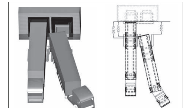
Figura 23. Cotas de montaje de una instalación incorrecta de guías de rueda.
