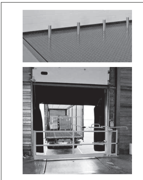
Figura 33. Rampa con bulones extraídos y barrera metálica.
