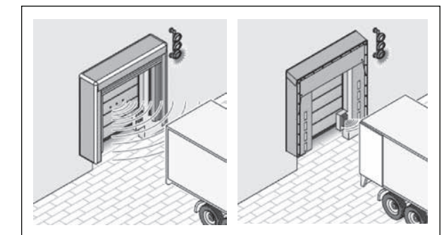
Figura 32. Asistente de acoplamiento mediante sensores y semáforo.
