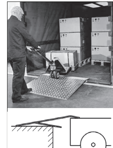
Figura 16. Puentes de carga.
