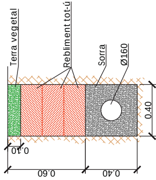
SECCIÓ PAV. TERRA
