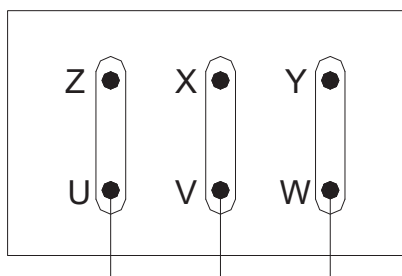
FIG. 1 Bobinado 230/400 red 230V Bobinado 400/690 red 400V
