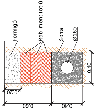
SECCIÓ PAV. FORMIGÓ
