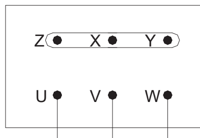
FIG. 2 Bobinado 230/400 red 400V
