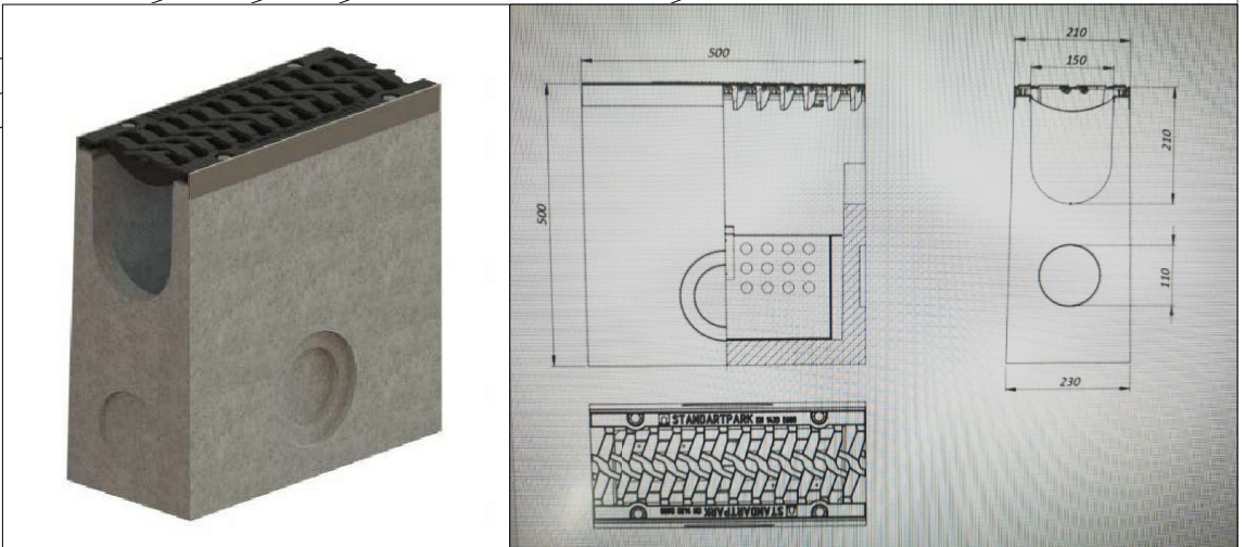
CANALETA DE DESGAIGUE TIPUS BETOMAX DRIVE
