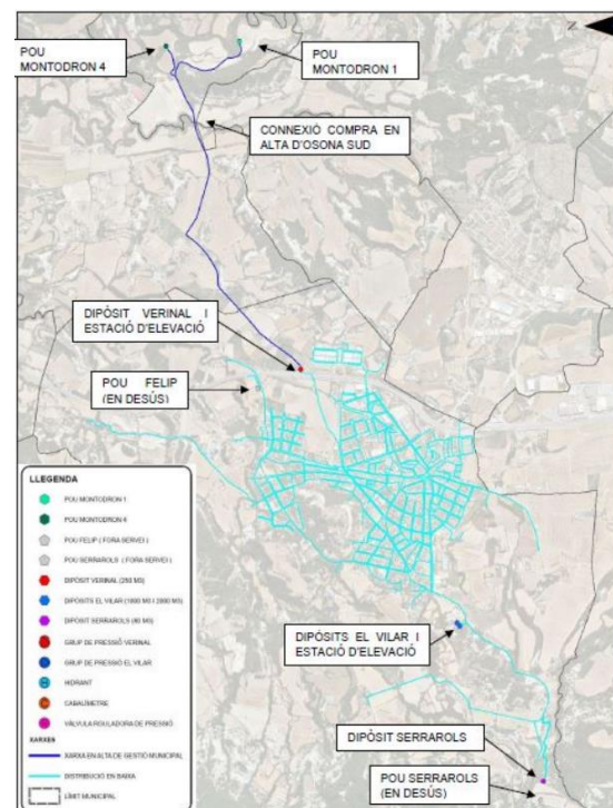
Figura 1. Plànol de la xarxa distribució-impulsió
