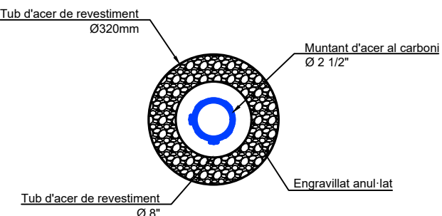
SECCIÓ A-A
