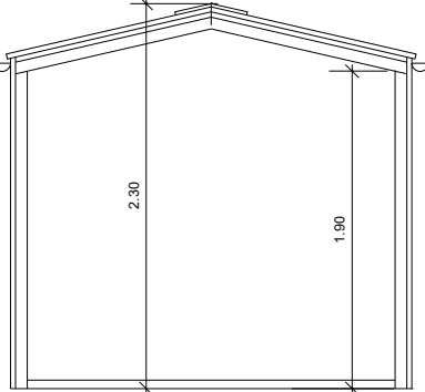
SECCIÓ A-B
