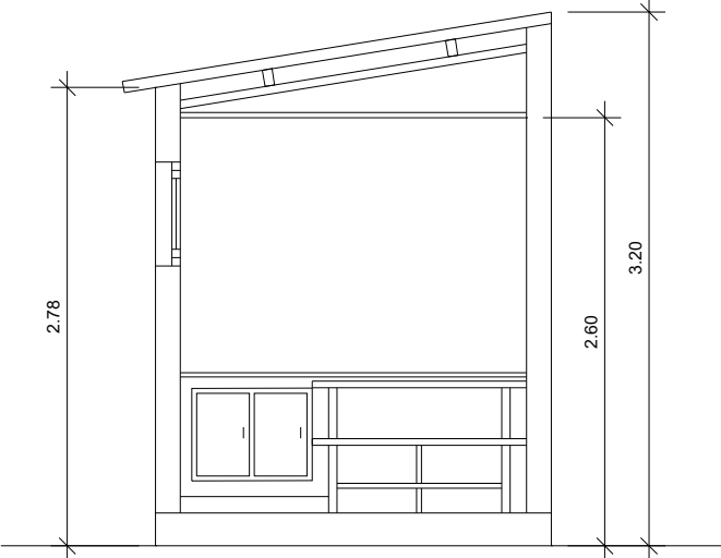
SECCIÓ A-B
