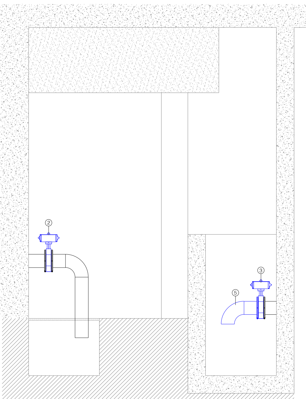
SECCIÓ B Escala: 1/25
