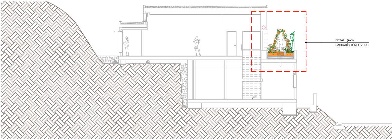
DETALLS PASSAIS TÚNEL VERD SECCIÓ B-B'
