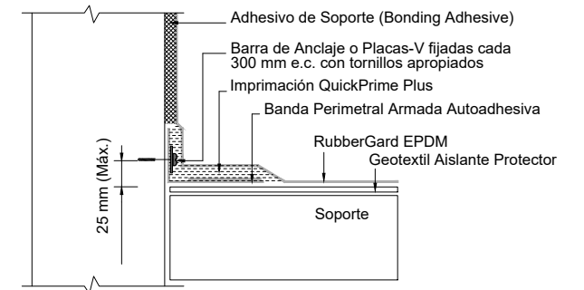
DETALL DE BANDA PREIMETRAL ARMADA AUTOADHESIVA VERTICAL
