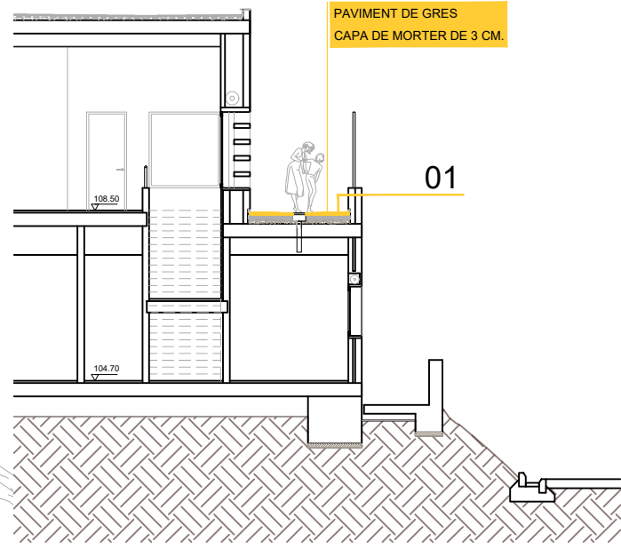
SECCIÓ 1-1'
