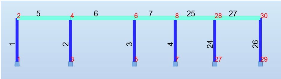
Fig: 7.1: vista del model de càlcul
