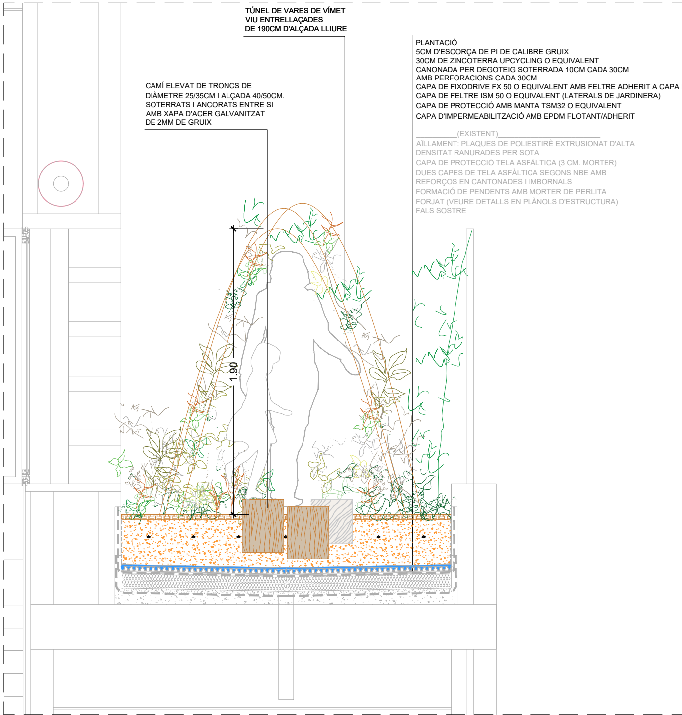
DETALLS PASSAIS TÚNEL VERD SECCIÓ A-A'
