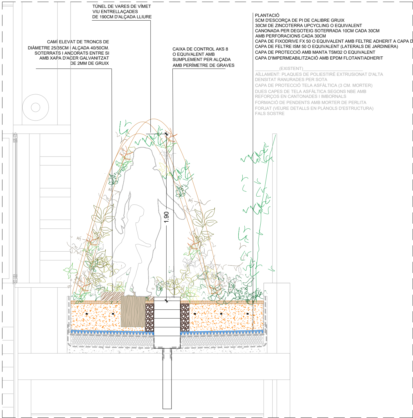
DETALLS PASSAIS TÚNEL VERD SECCIÓ B-B'
