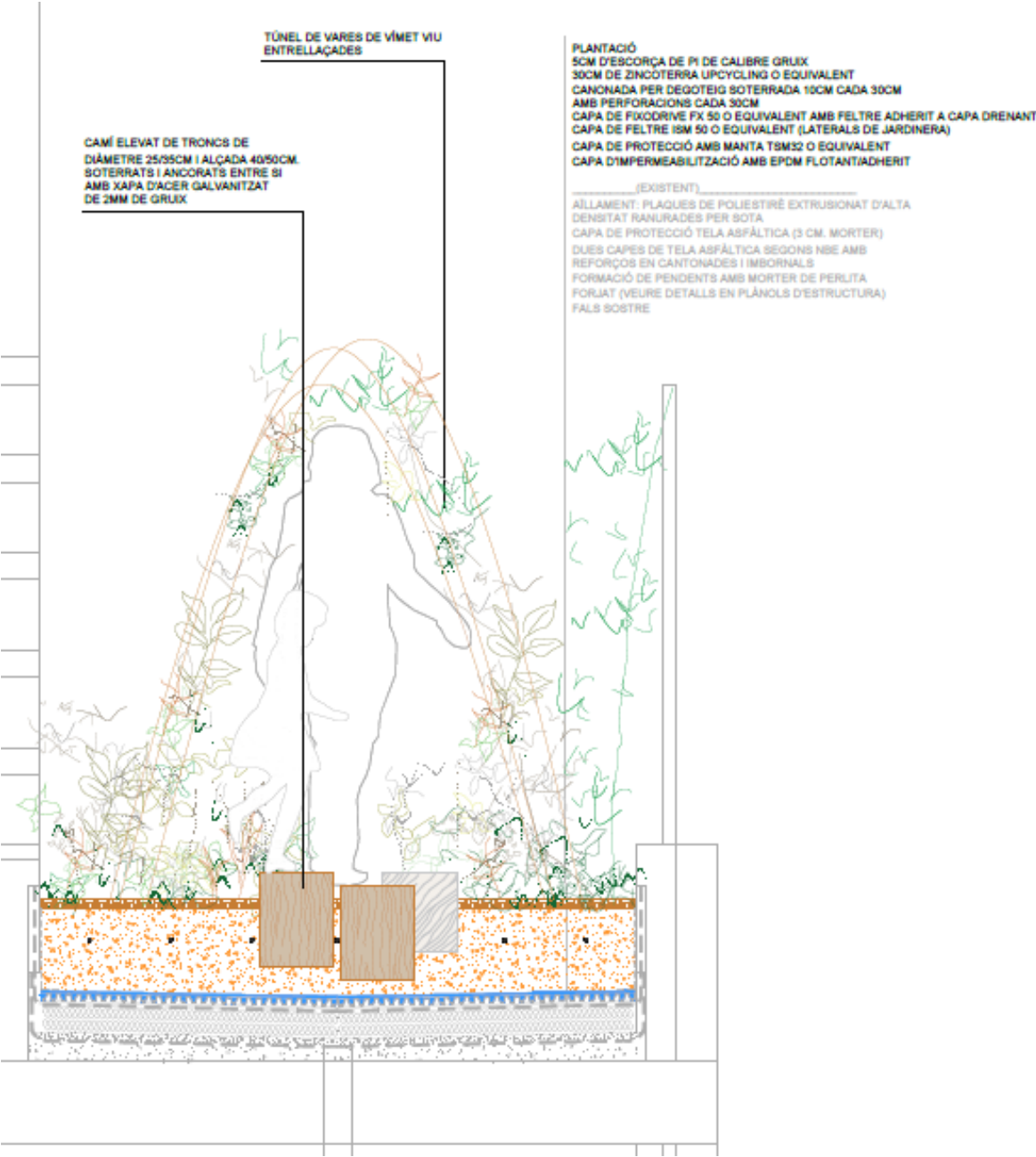
Secció tipus del túnel d'aventura
