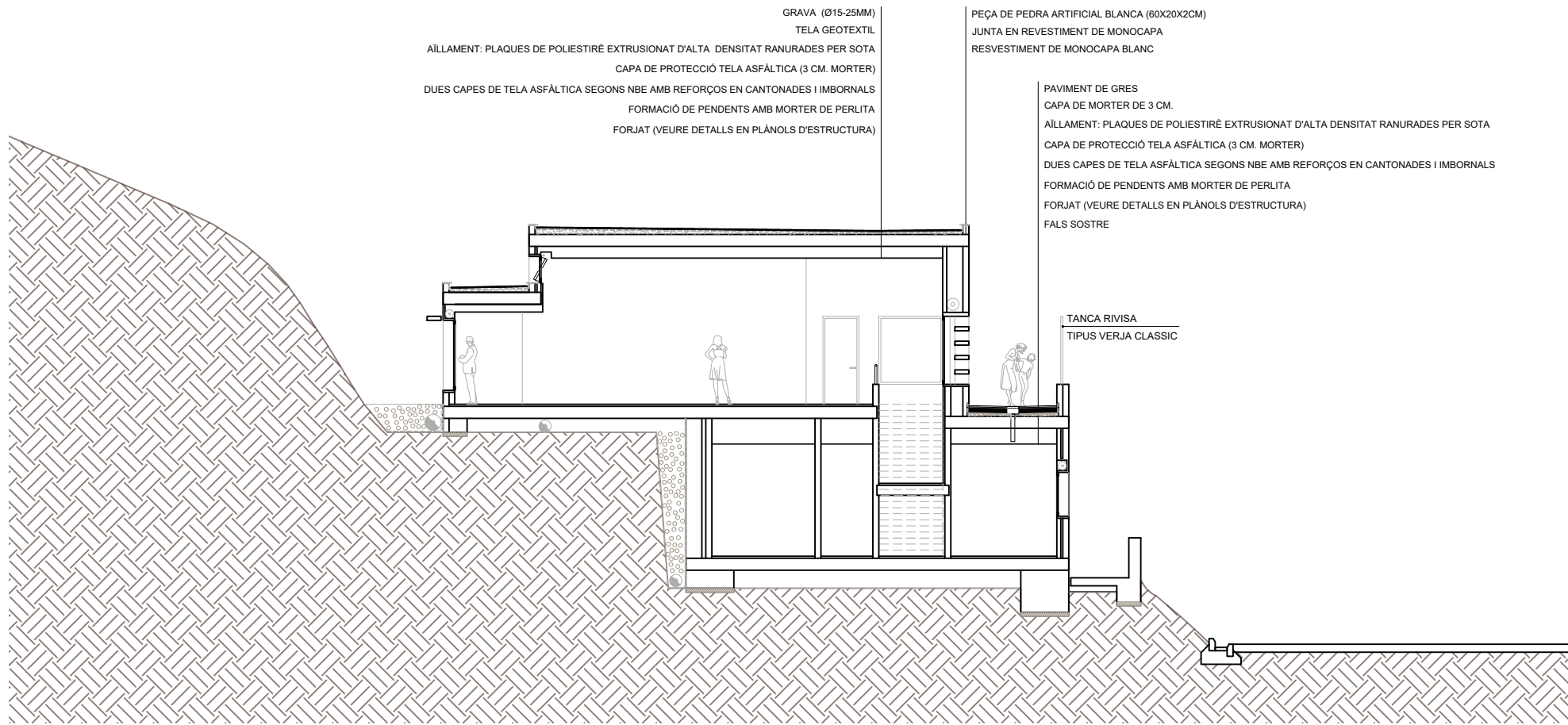
SECCIÓ 1-1'
