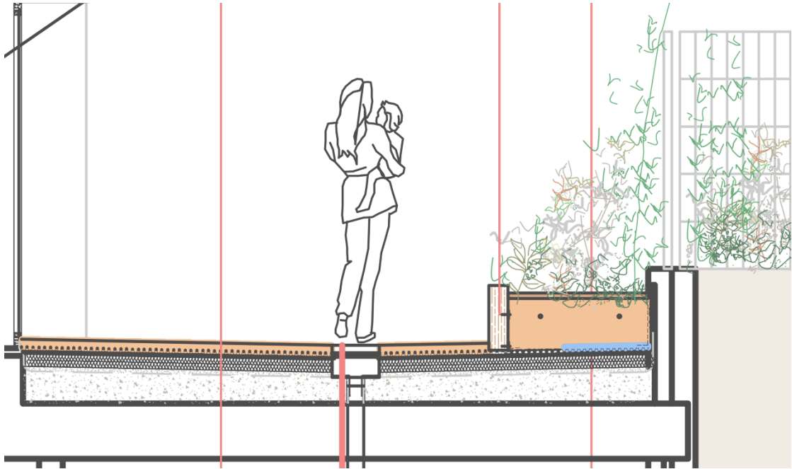
Secció de la coberta amb zona enjardinada amb muret de contenció
