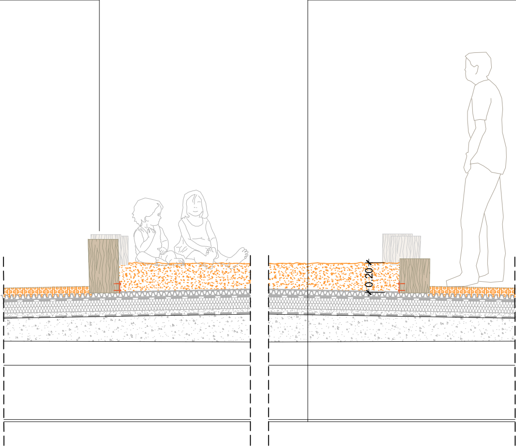
DETALL SORRAL SECCIÓ A-A'
