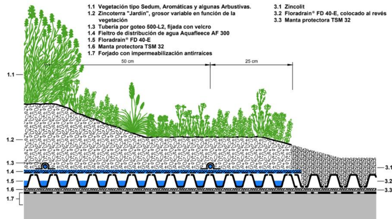
Esquema de la solució amb terres fins a 20-30cm d'espessor amb sistema de reg per degoteig integrat i micro-aljub integrat
