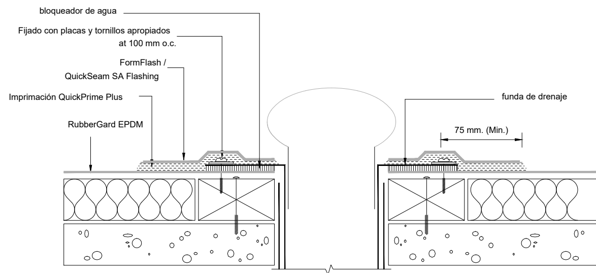
DETALL DE BAIXANT/SUMIDER
