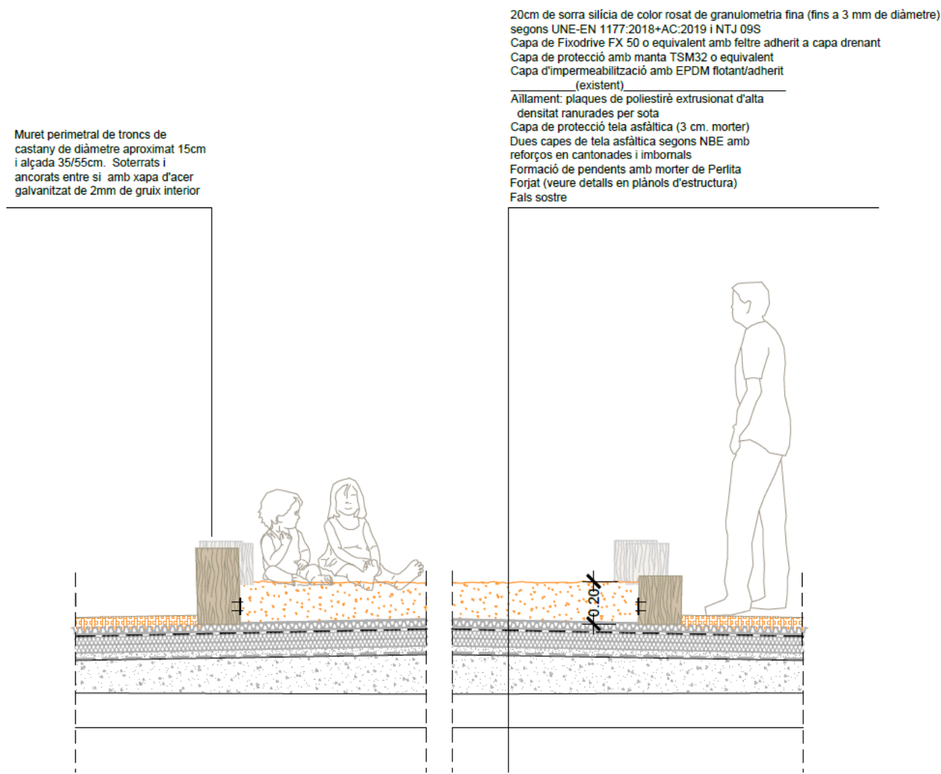
Planta i Secció de detall de la solució tècnica
