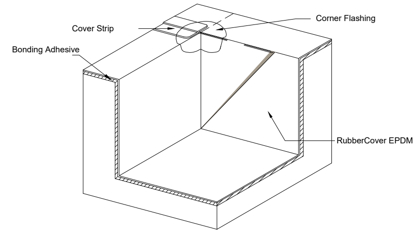
DETALL DE CANTONADA 2
