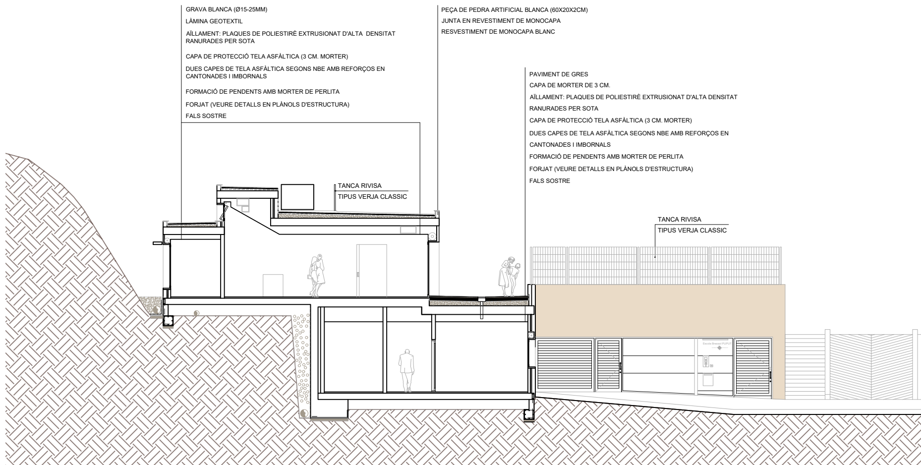
SECCIÓ 2-2'
