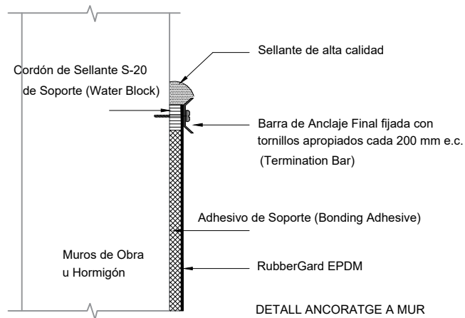
DETALL ANCORATGE A MUR
