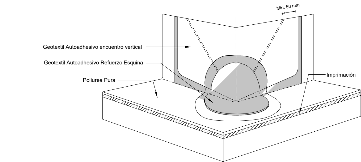
DETALL DE CANTONADA 1
