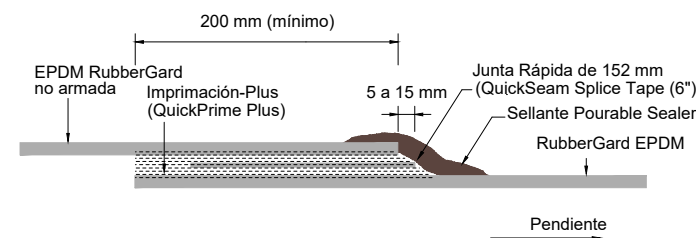
DETALL DE JUNTA STANDARD
