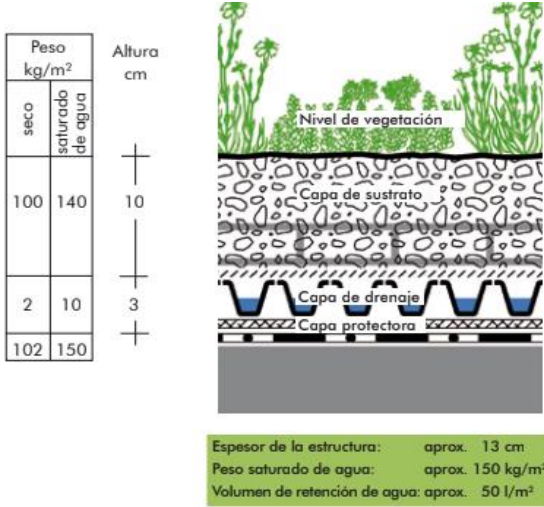
Esquema del pes saturat del sistema de coberta verda
