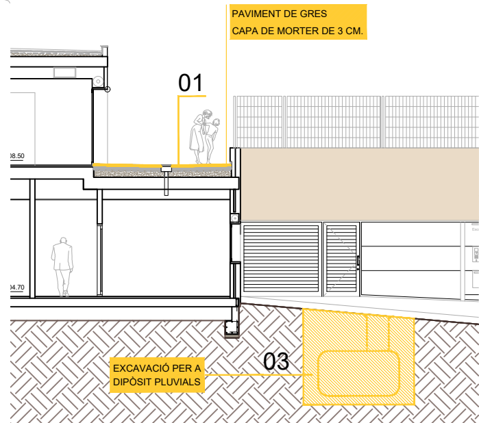
SECCIÓ 2-2'
