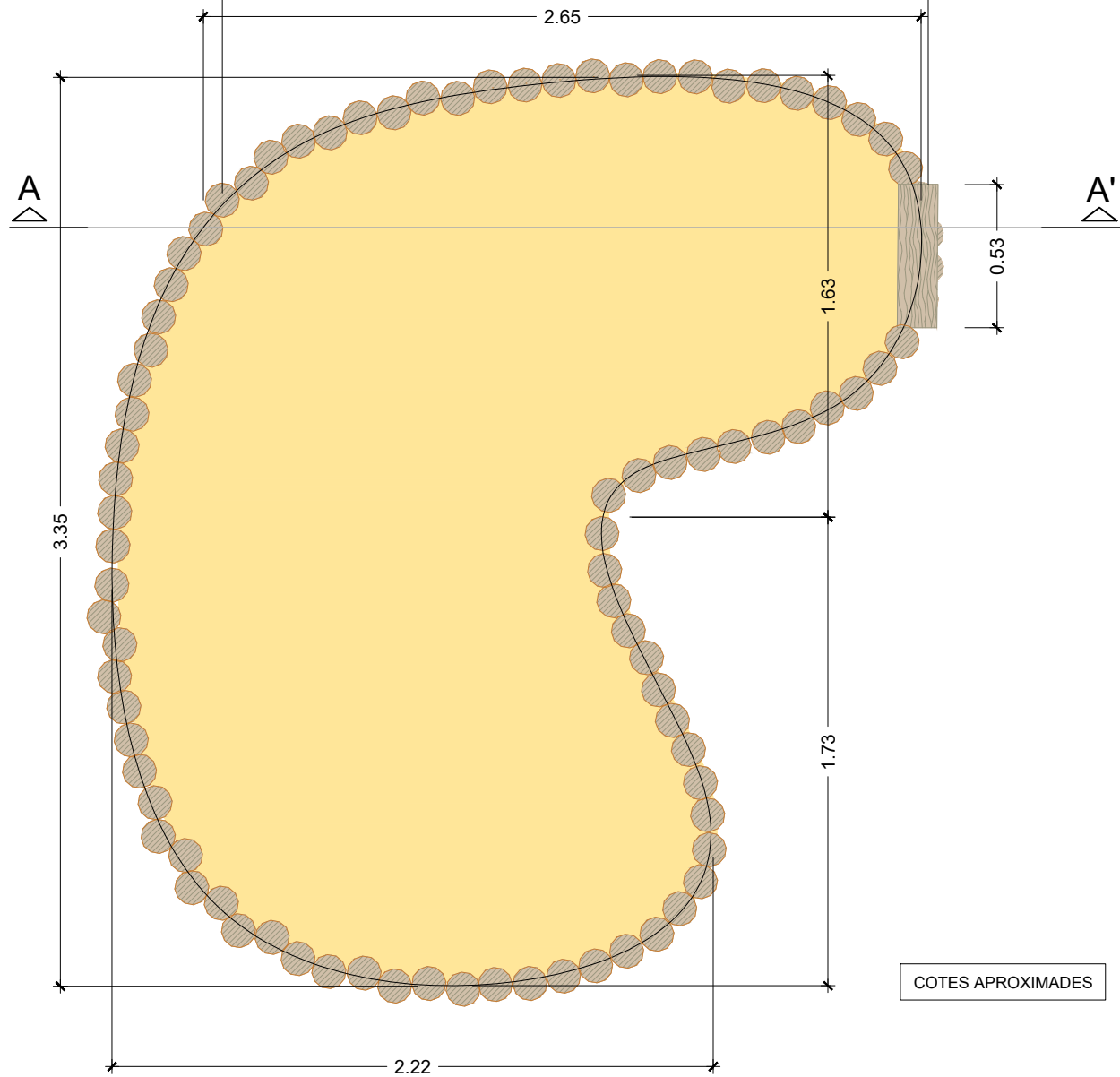
DETALL SORRAL PLANTA
