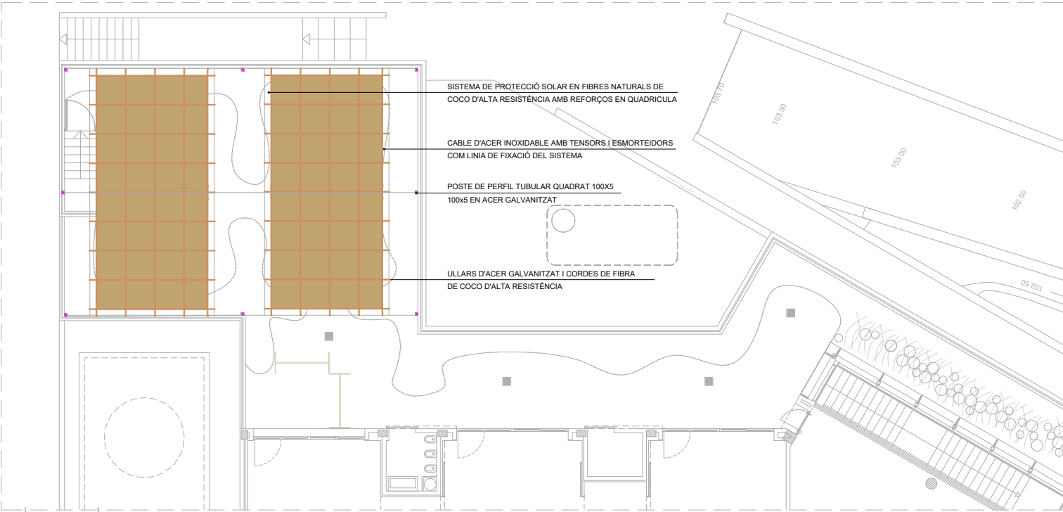
PLANTA
