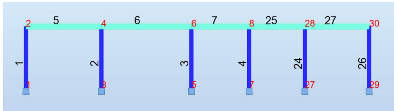
Fig: 6.1: vista esquemàtica del model estructural
